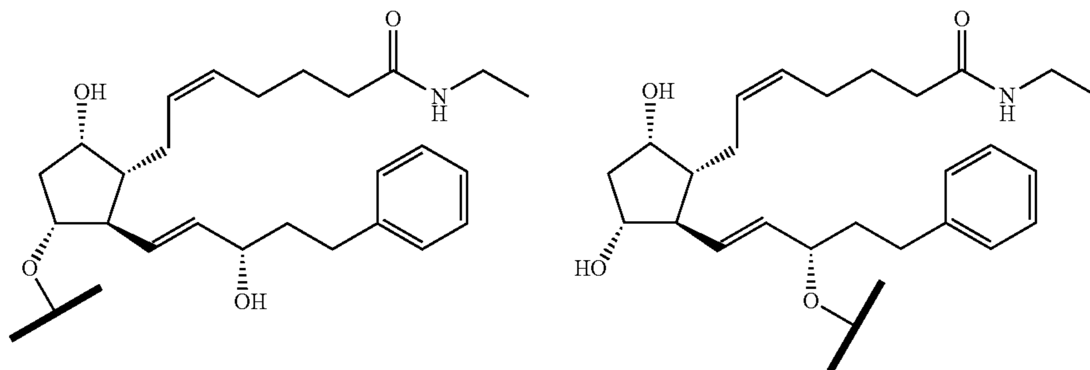
Bimatoprost
