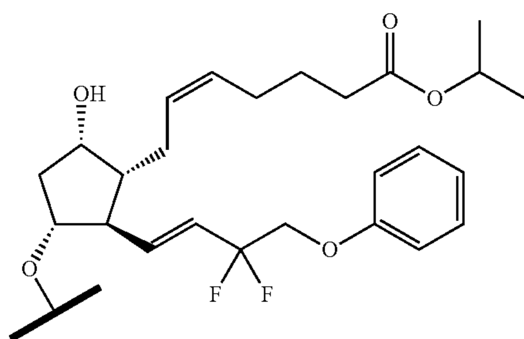
Tafuprost
