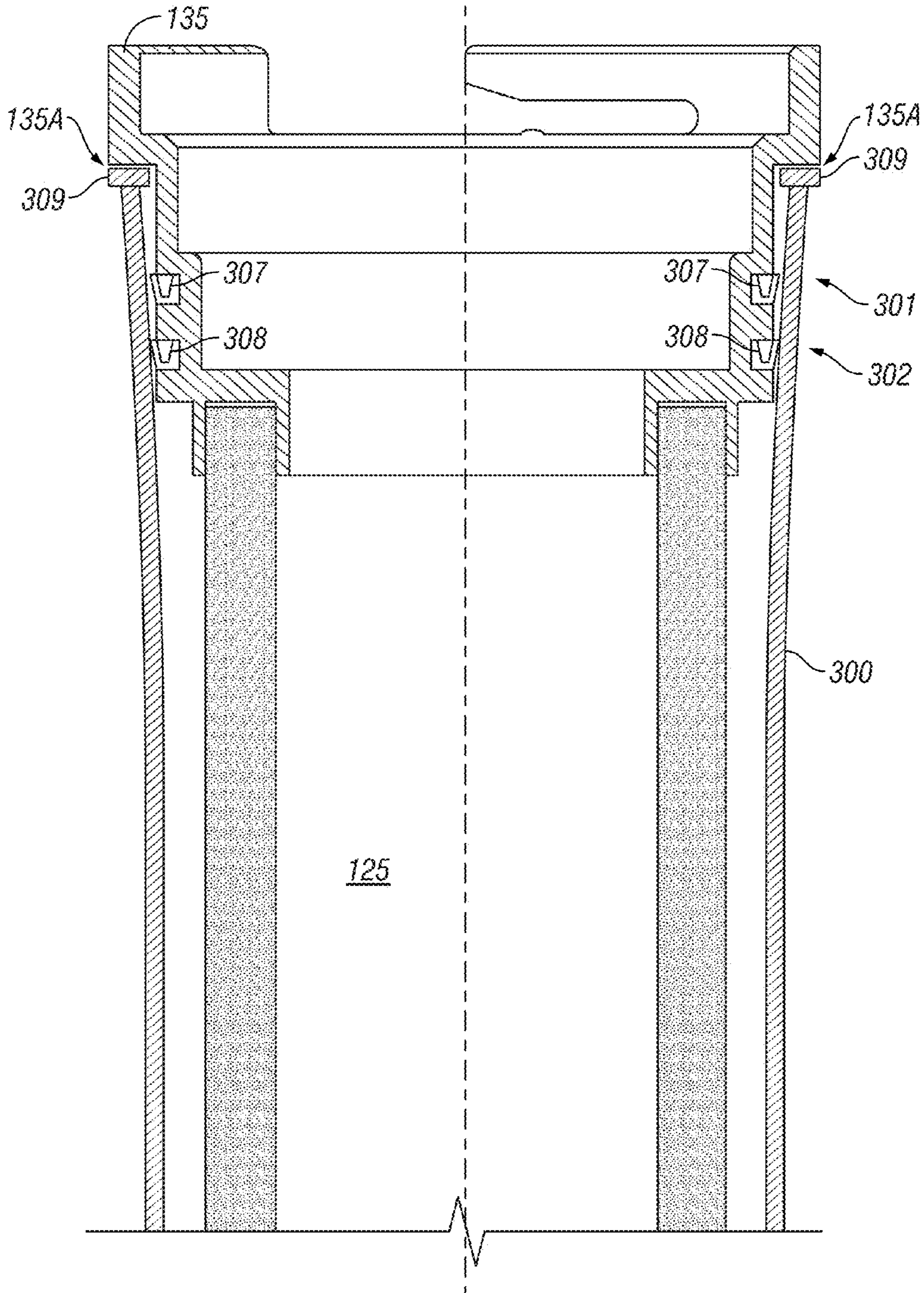
FIG. 19
