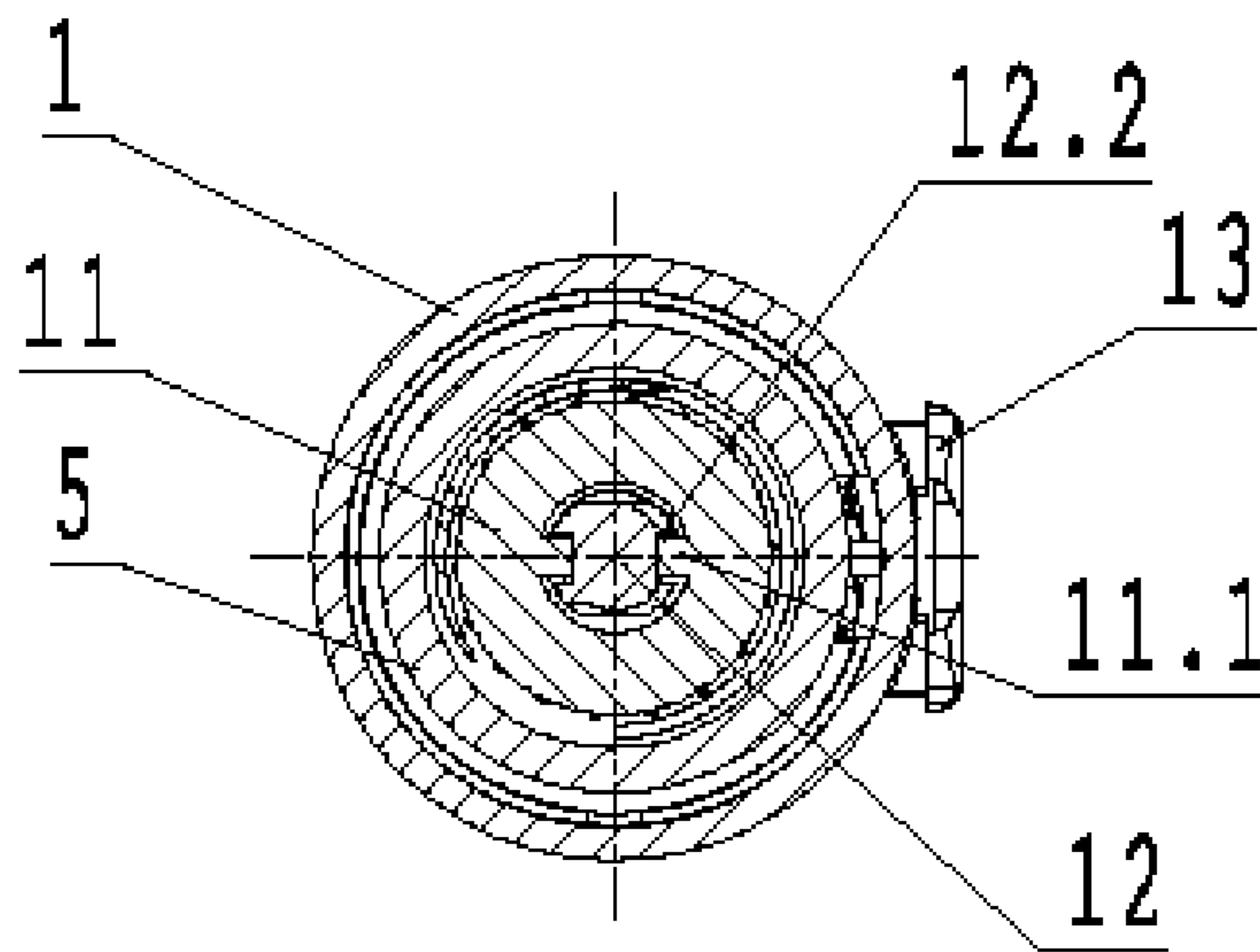
Przek. E-E
