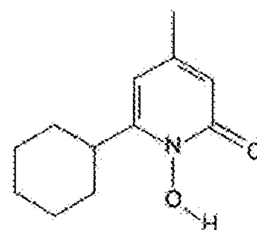
Ciclopirox
