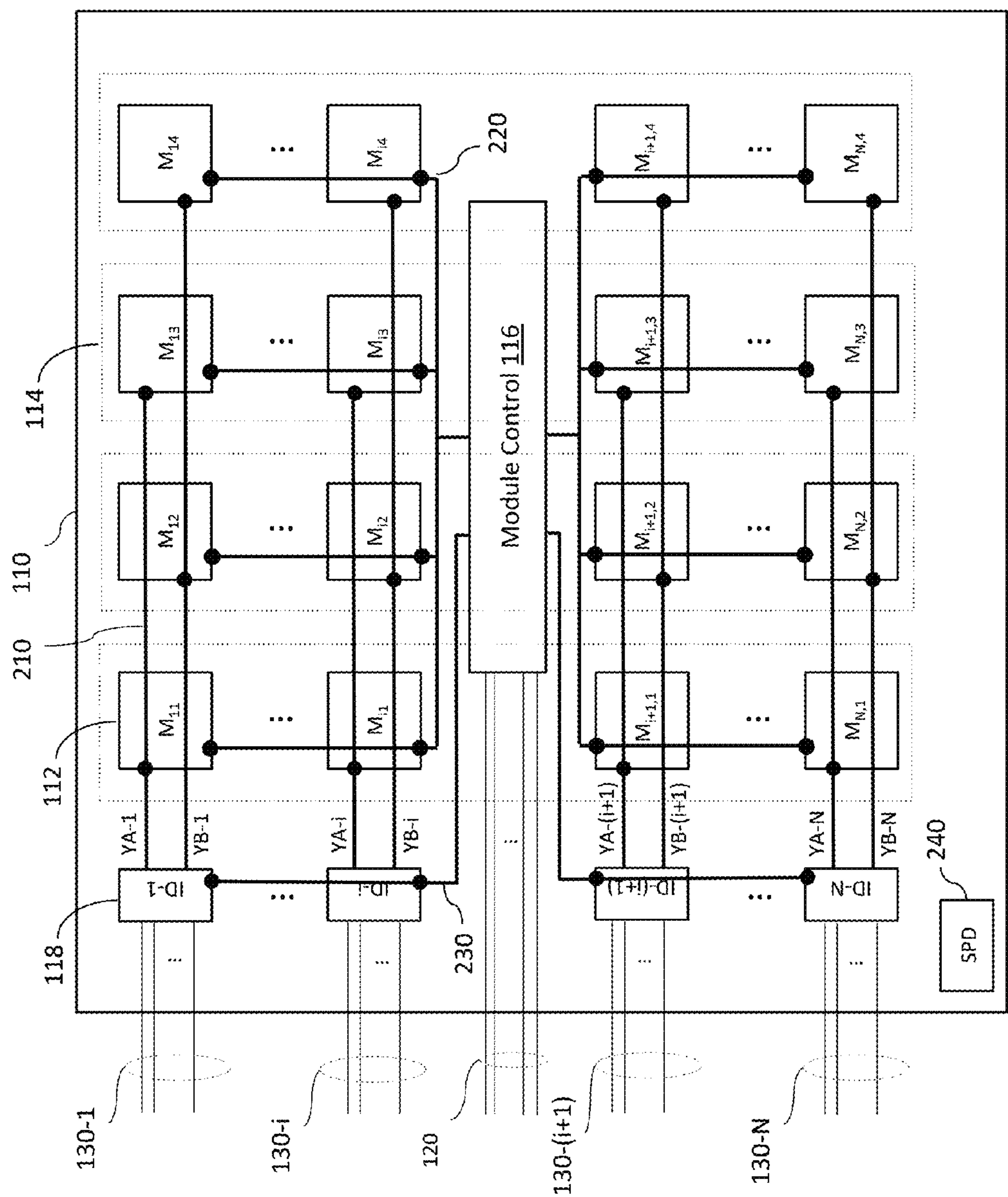
FIG. 2B
