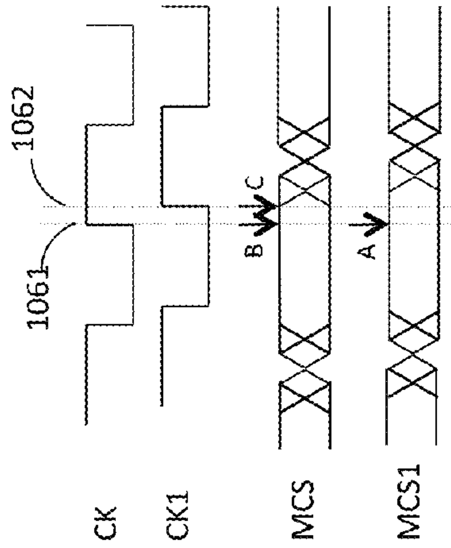
FIG. 10B
