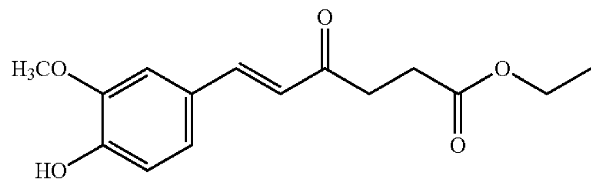
Monomer-7
