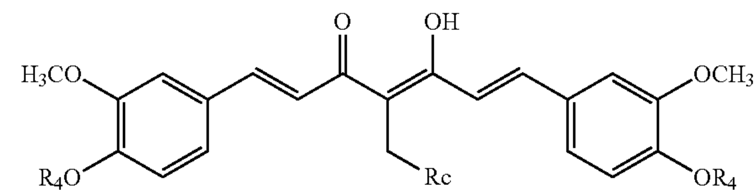
Monomer-6
