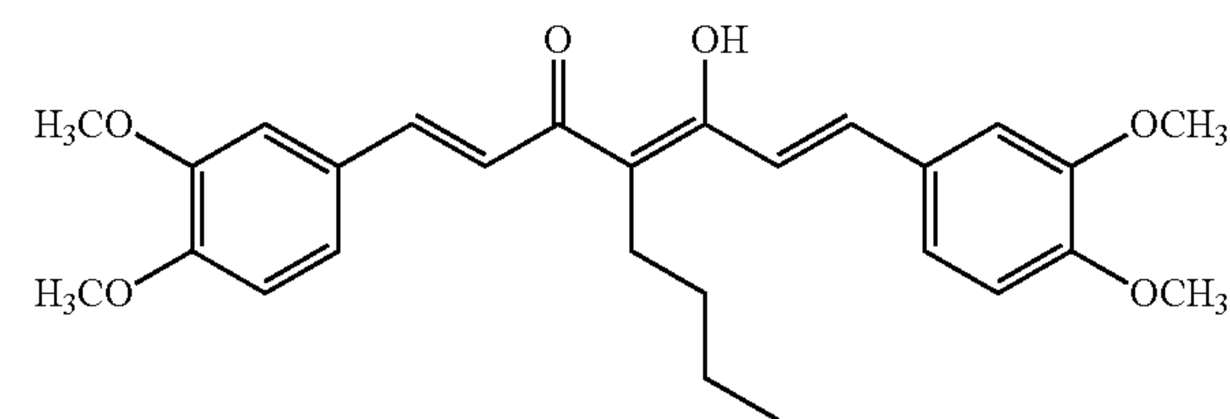
Monomer-5
