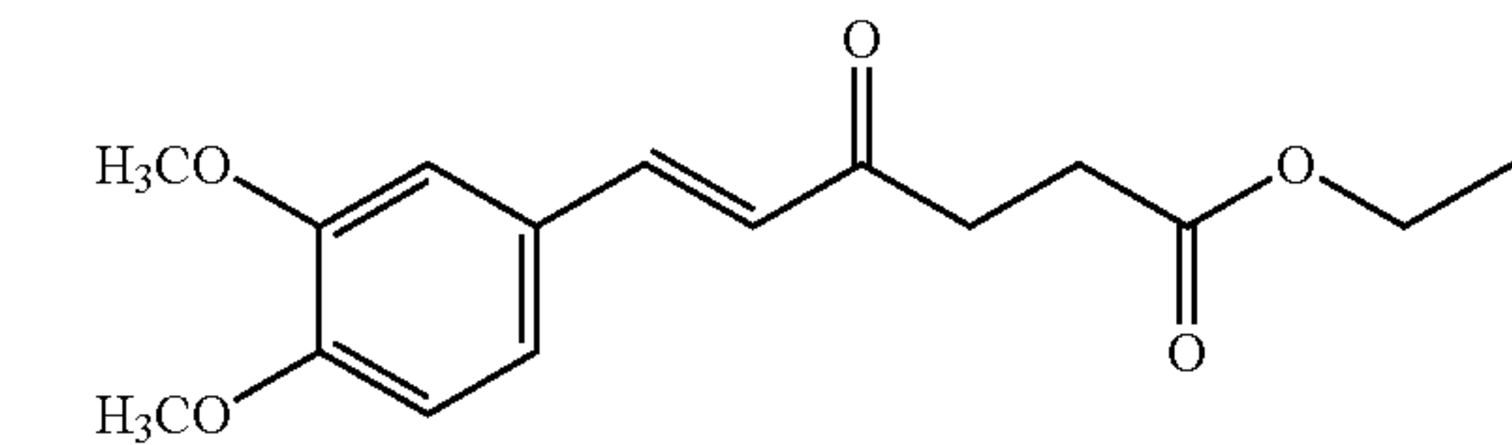
Monomer-6
