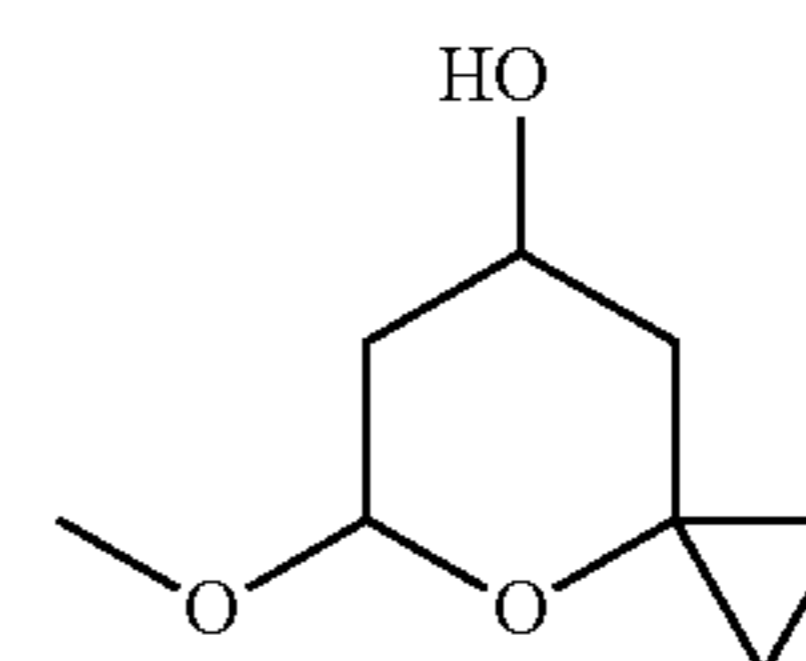
Cap 5, step f
