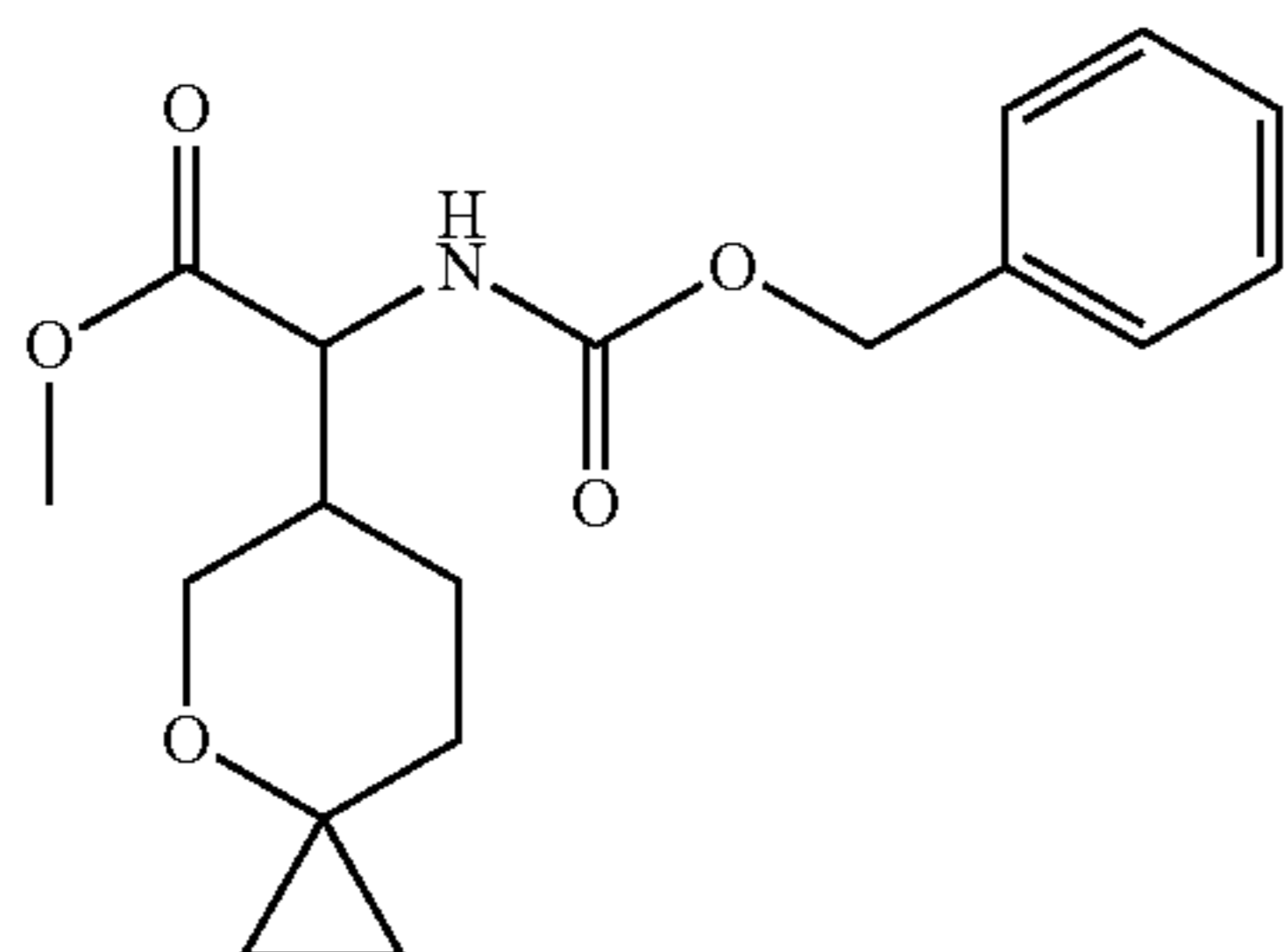
Cap 8, step i
