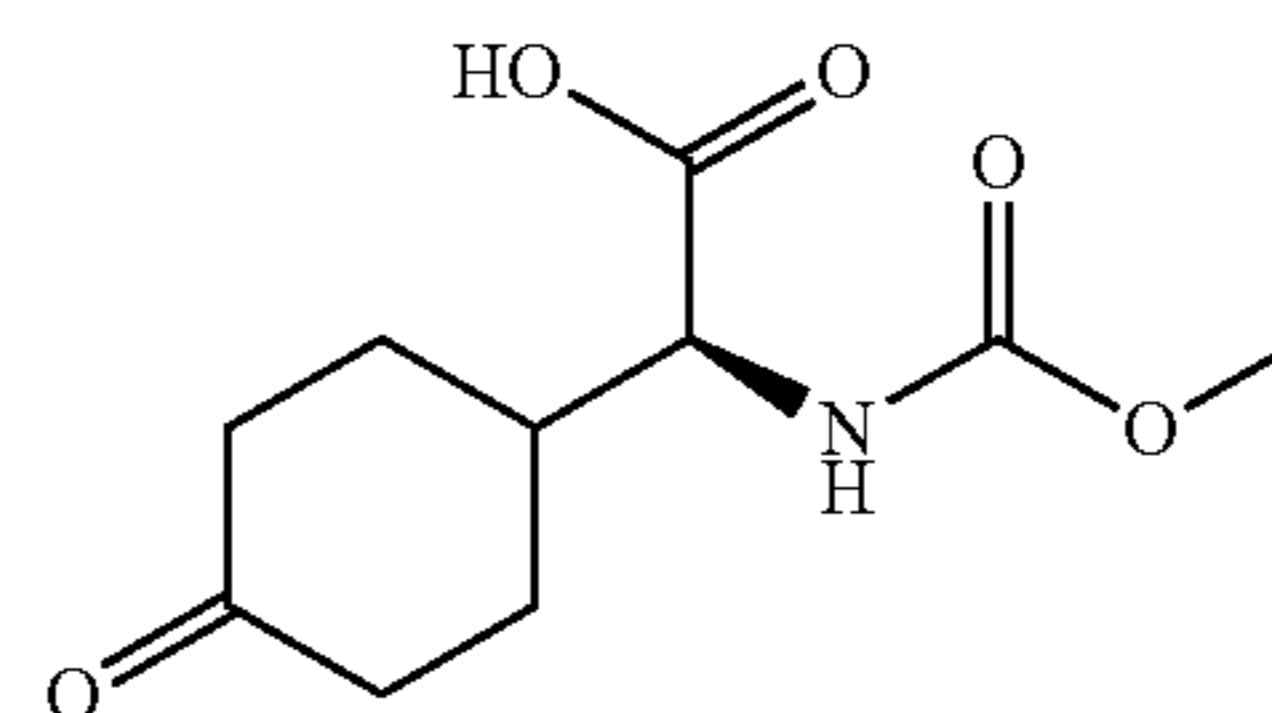
Cap-6
