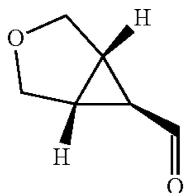
Cap-1 step c
