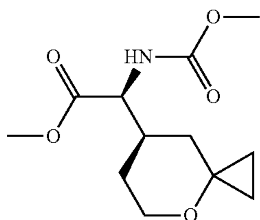
Cap 5.1, step k
