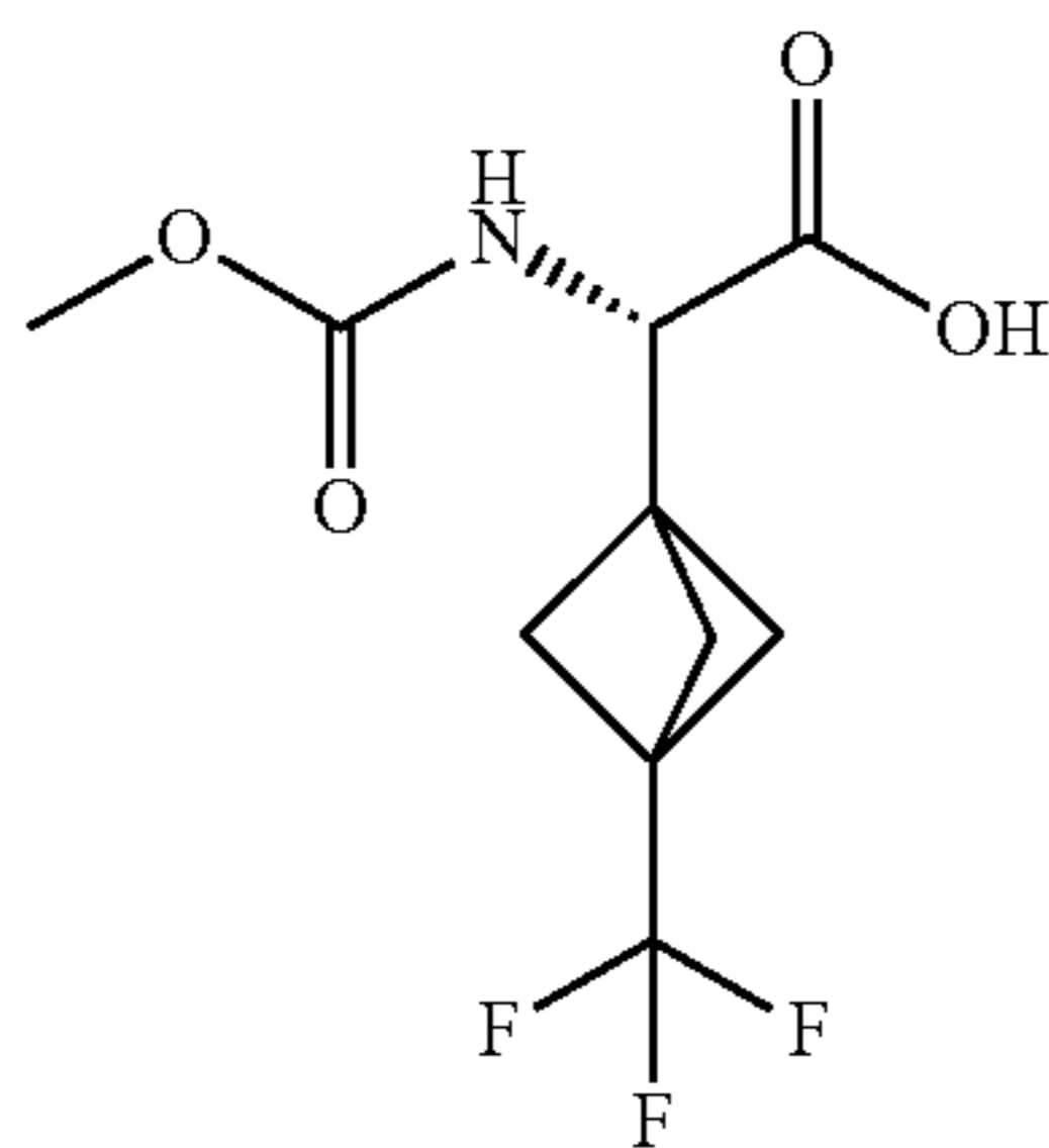
Cap-7
