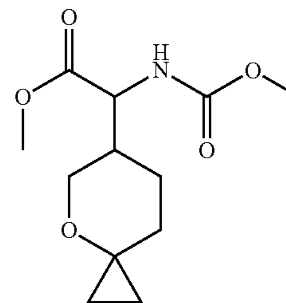
Cap 8, step j.1
