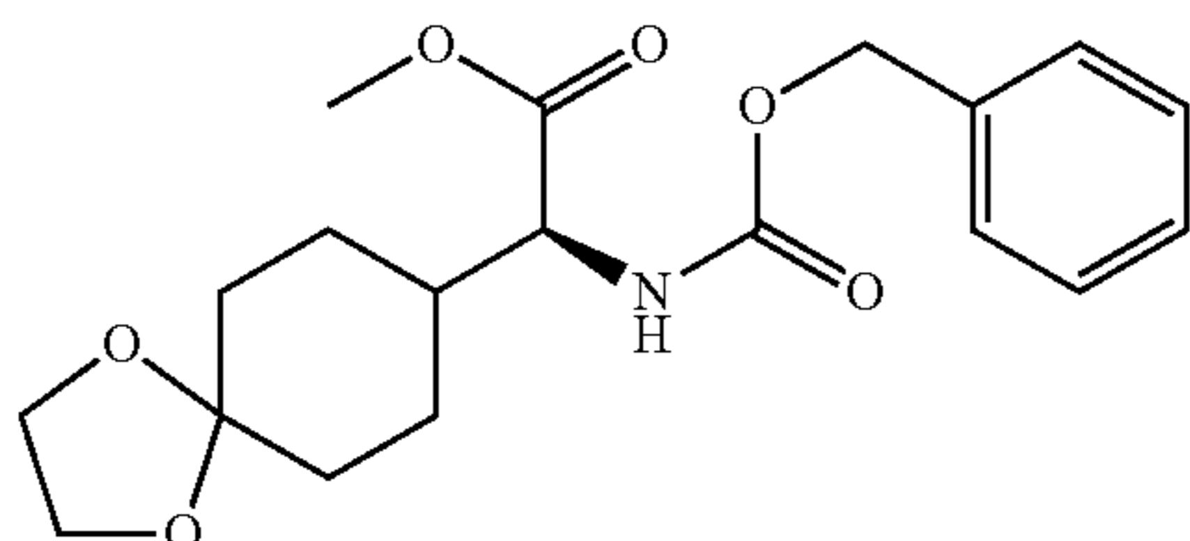
Cap-6, step b
