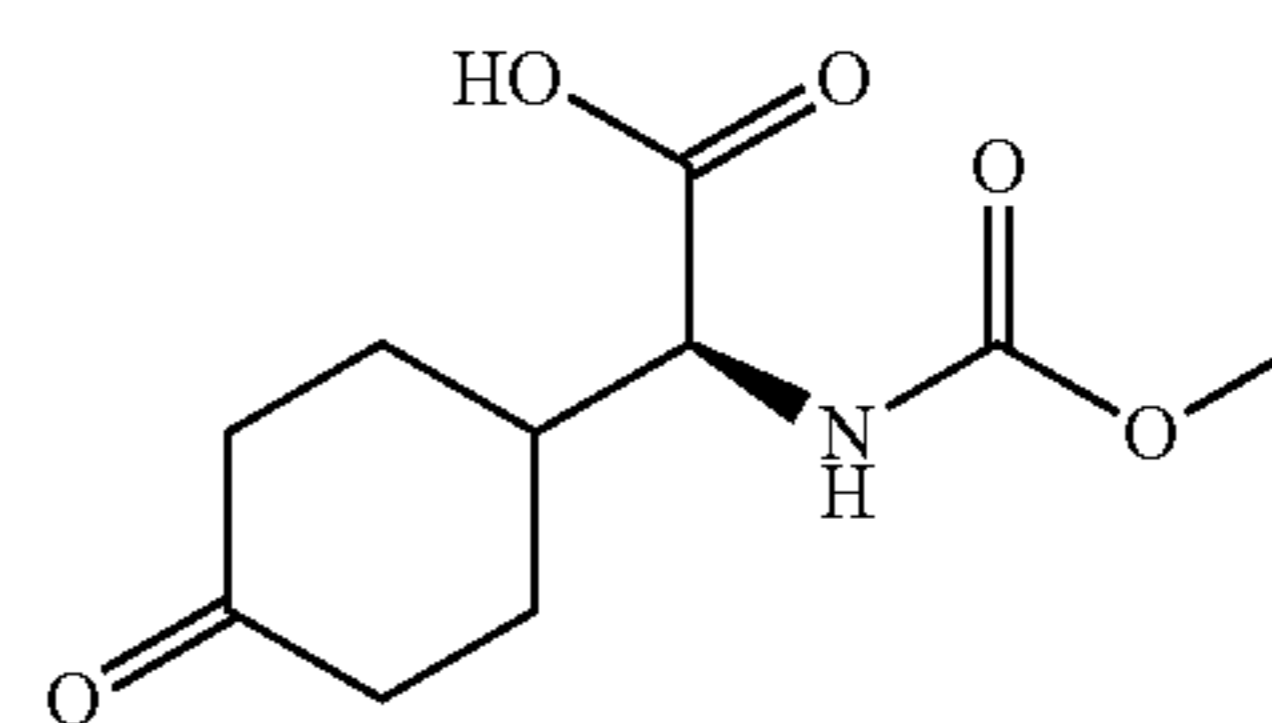
Cap-6, step a
