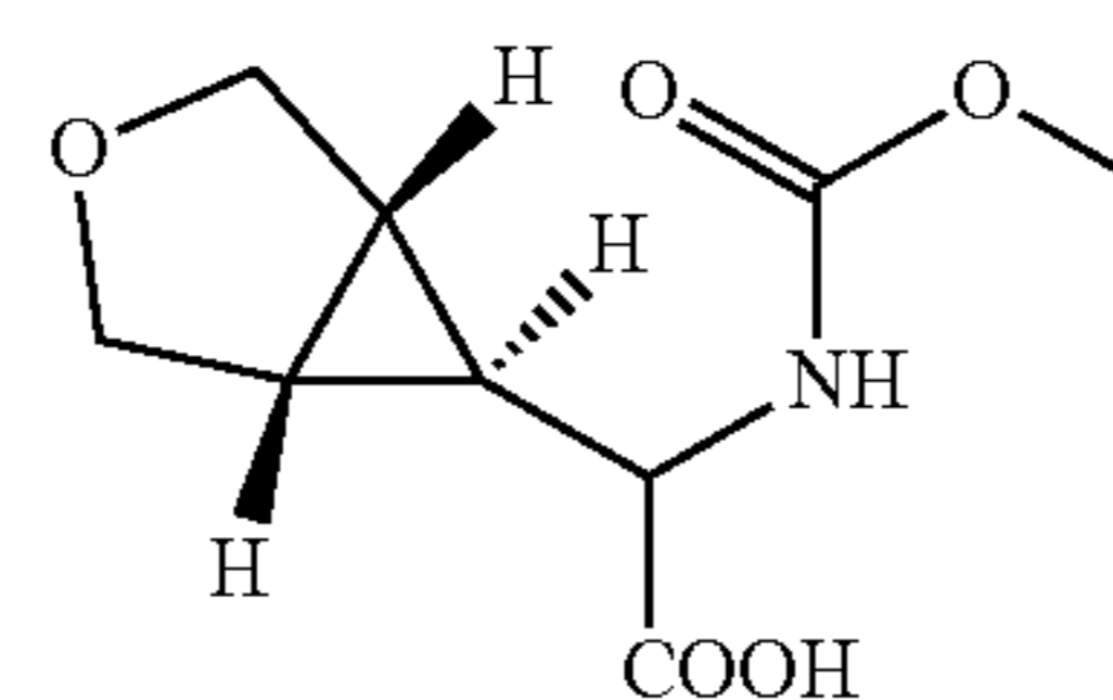
Cap-1
