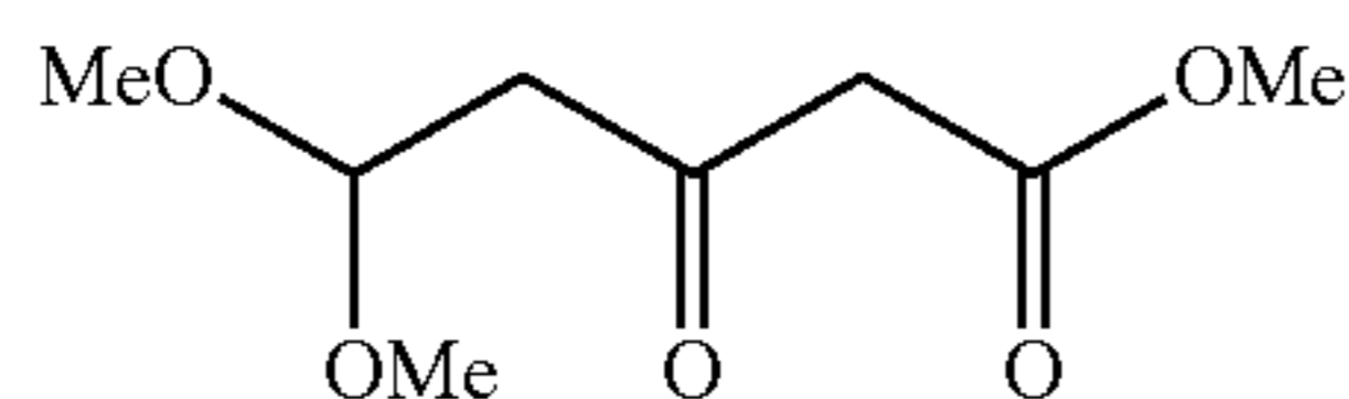
Cap 5, step b
