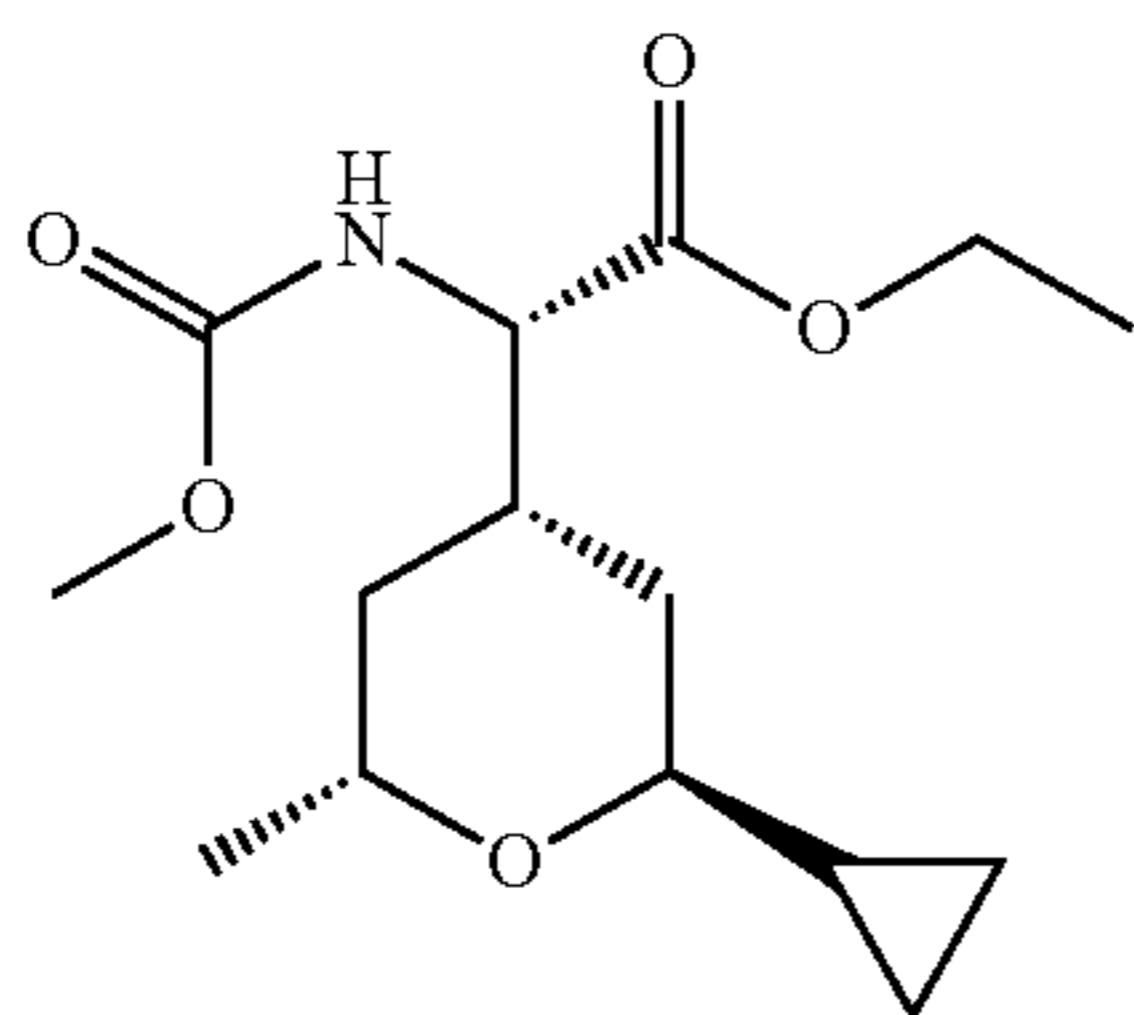
Cap 15.4, step d
