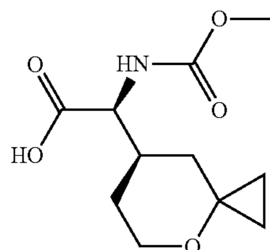
Cap 5.1
