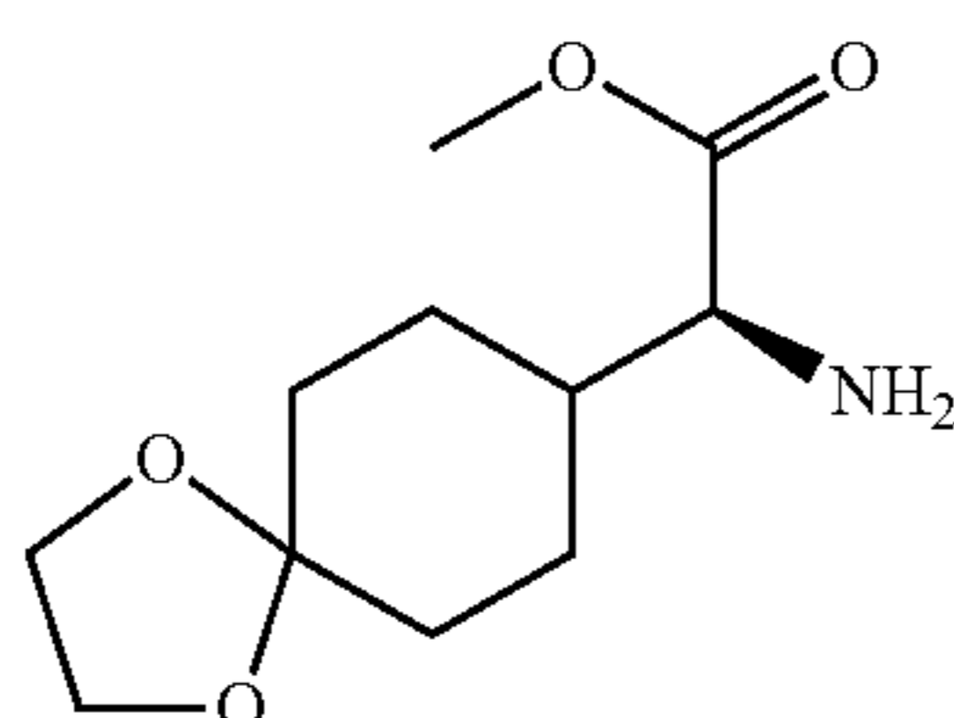
Cap-6, step c
