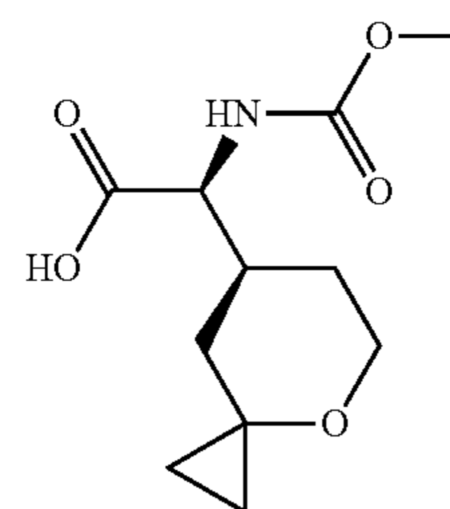
Cap 5.2
