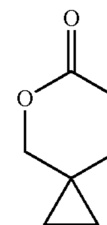
Cap 8, step g
