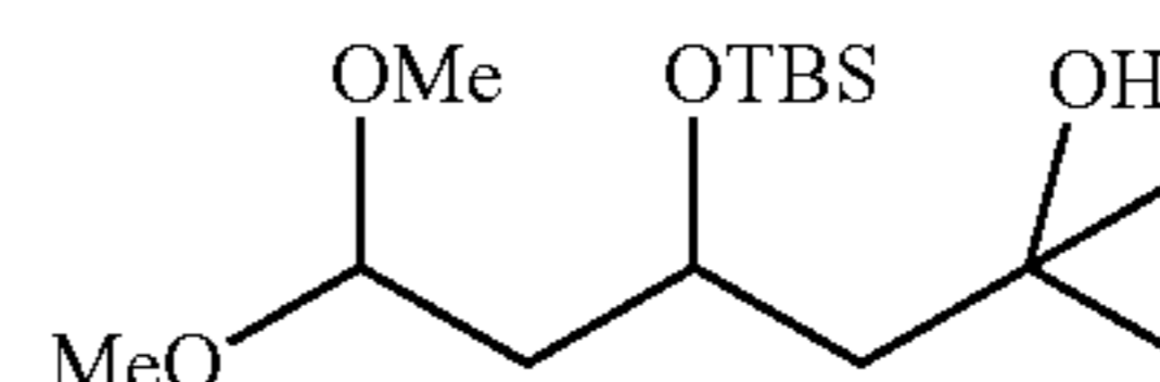
Cap 5, step e
