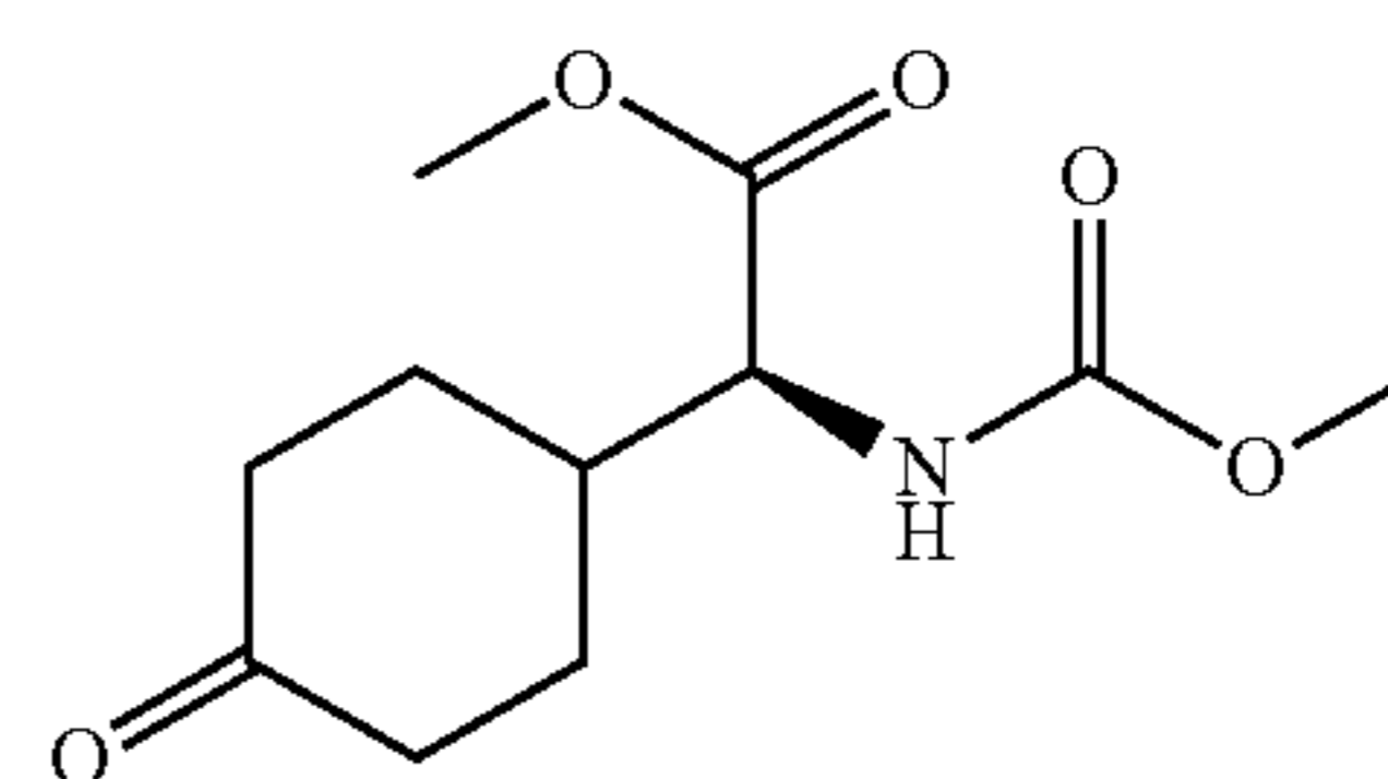
Cap-6, step e
