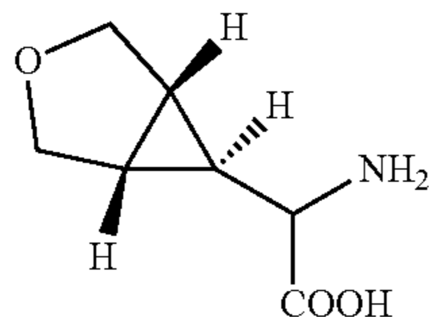
Cap-1 step e
