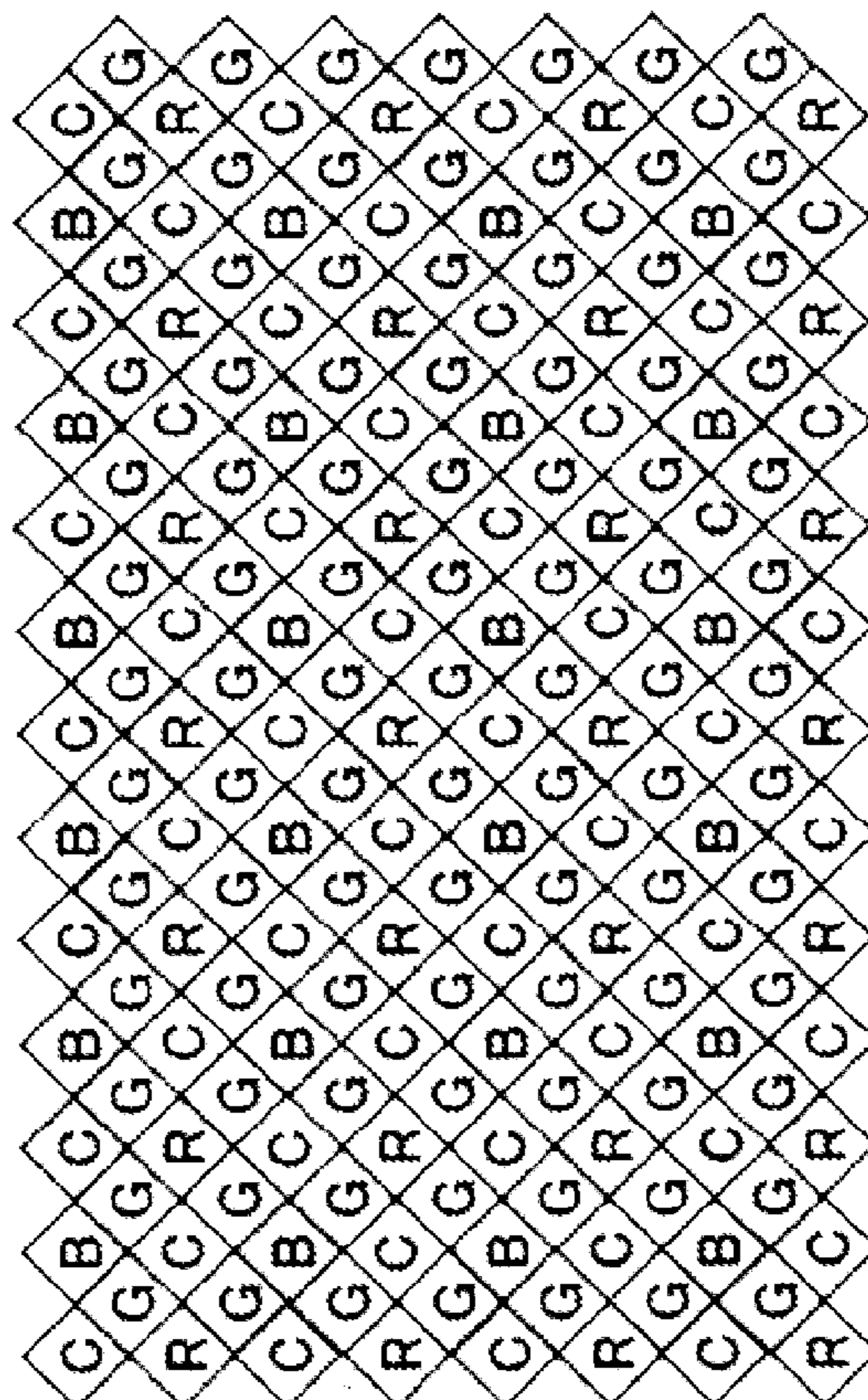
ARRAY 2 (FIG. 9)
