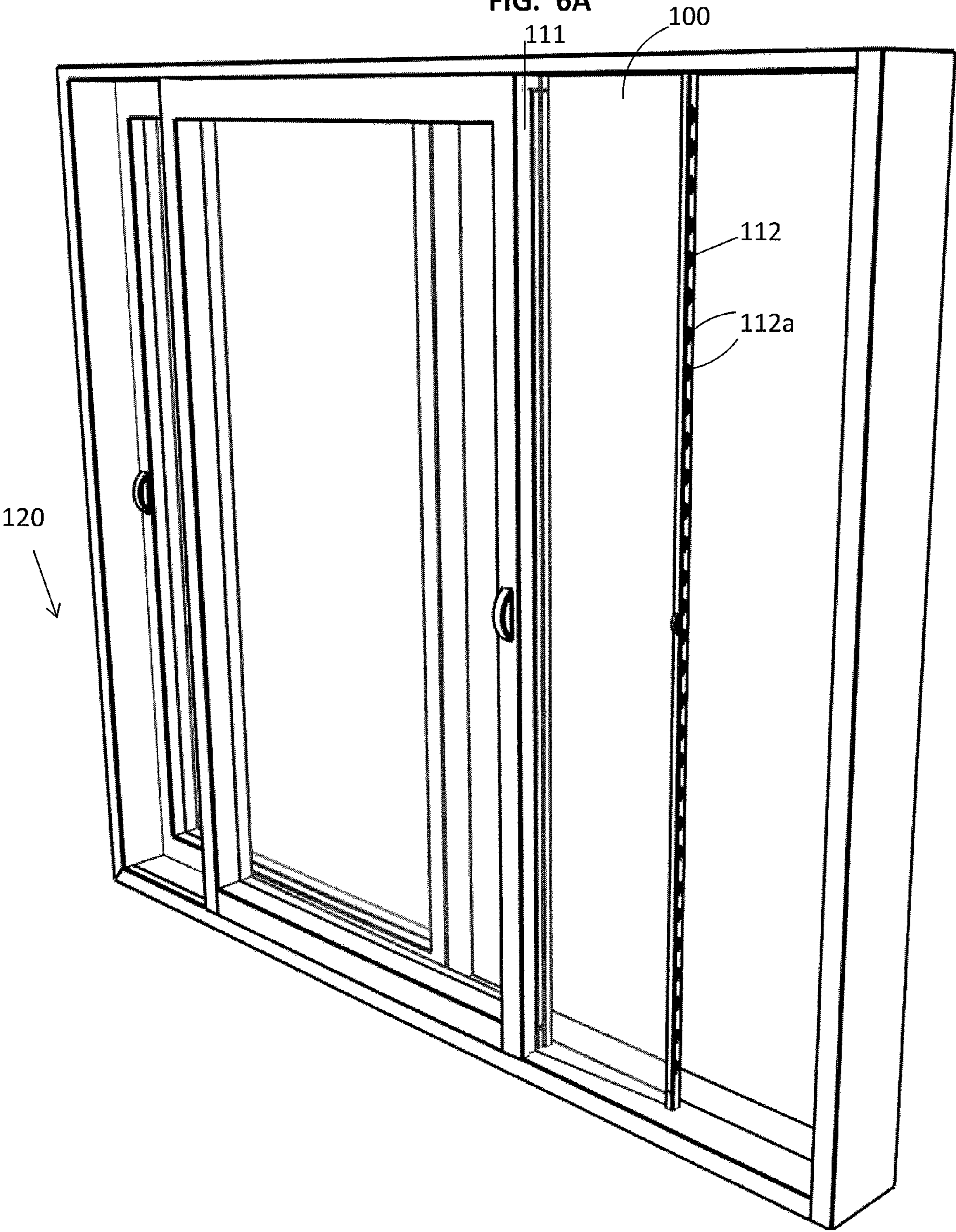
FIG. 6A
