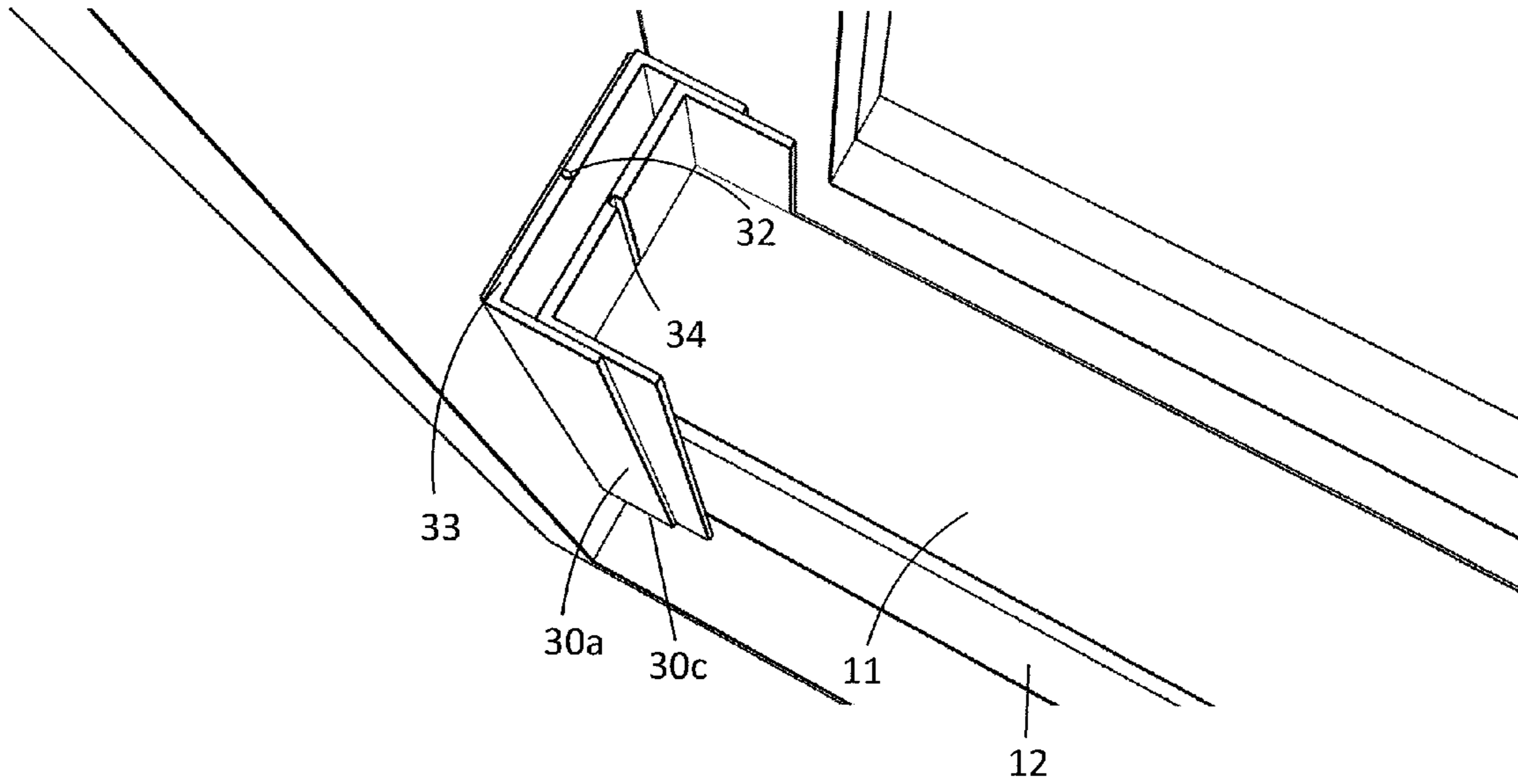
FIG. 10A
