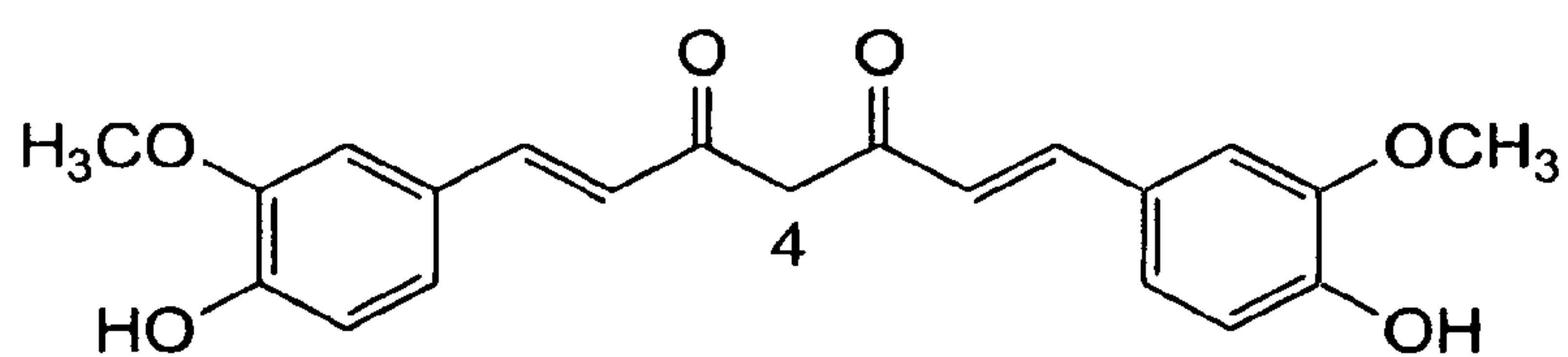
Curcumin
