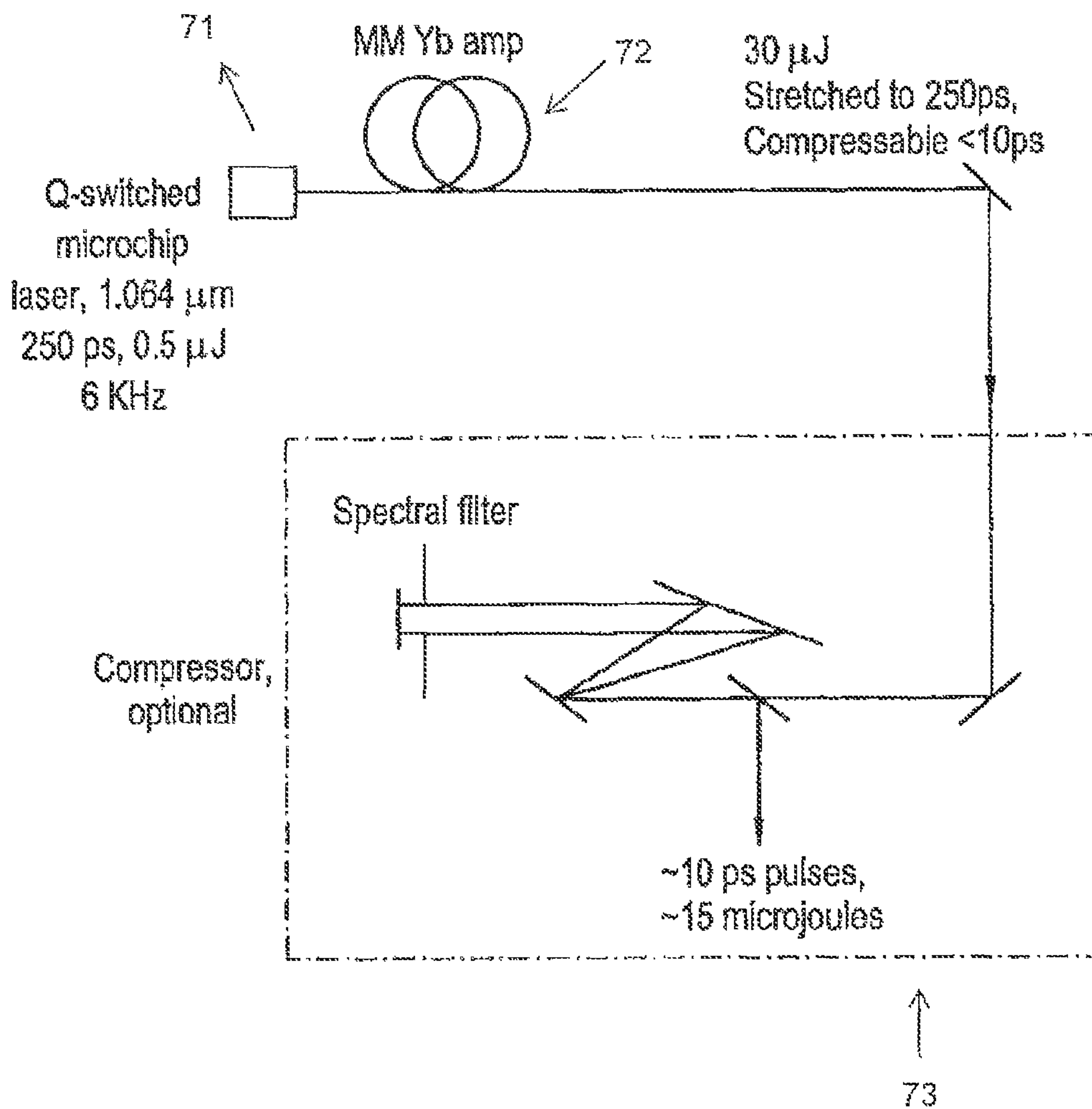
FIG. 7
