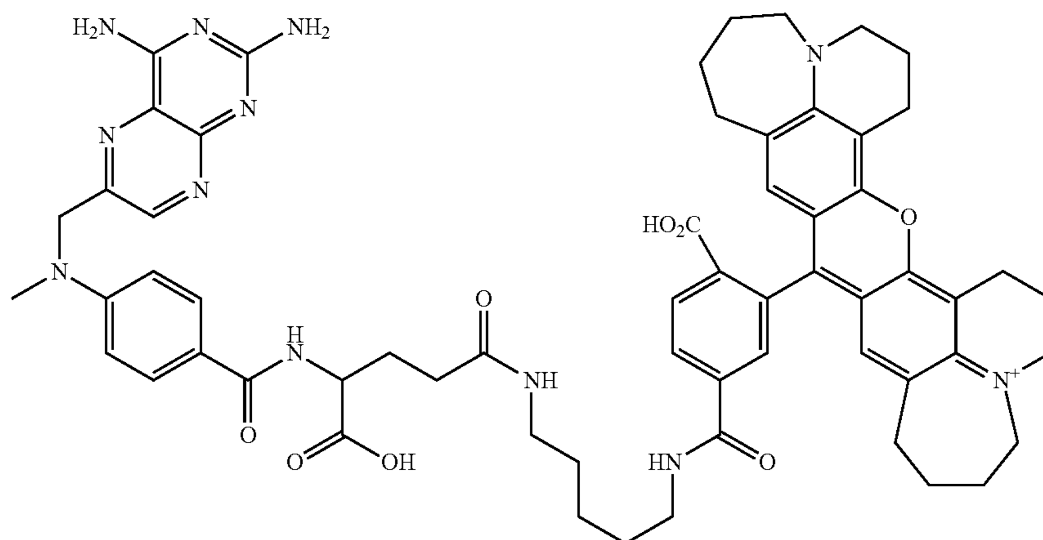
PBI-4890 Methotrexate-TOM
