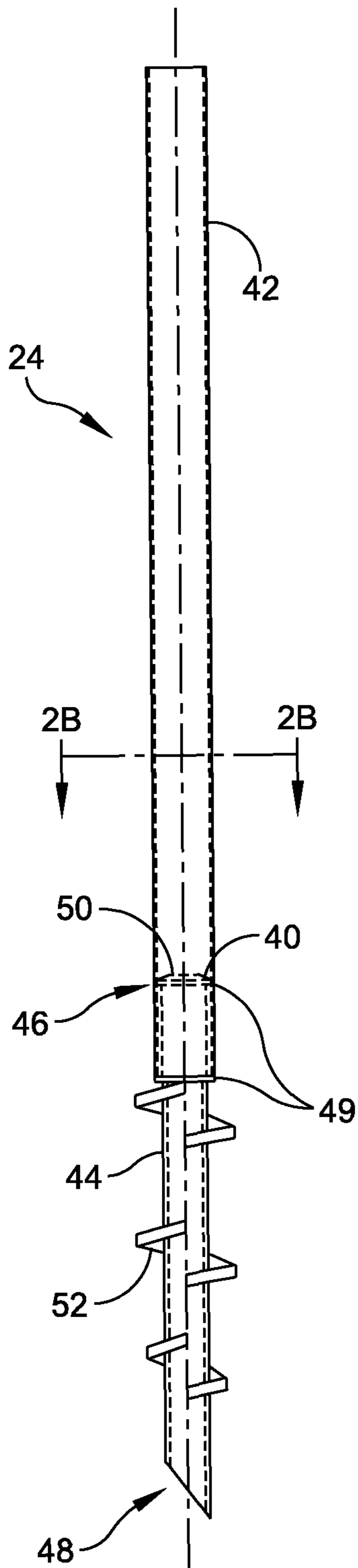
FIG. 2A
