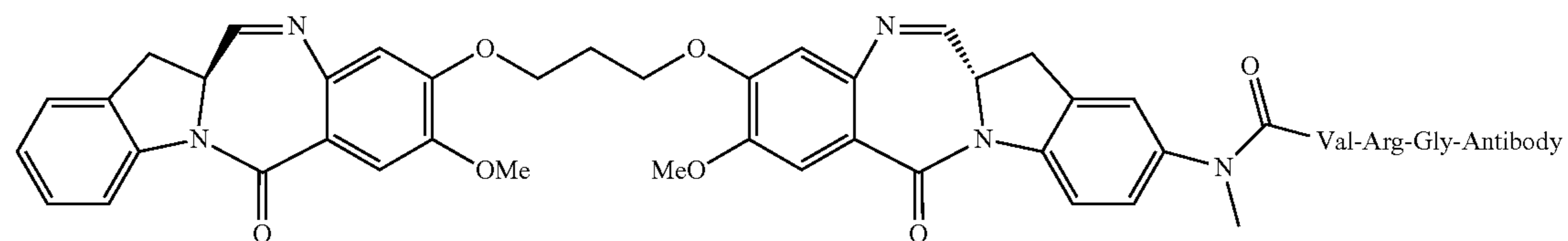
Dimer 6
