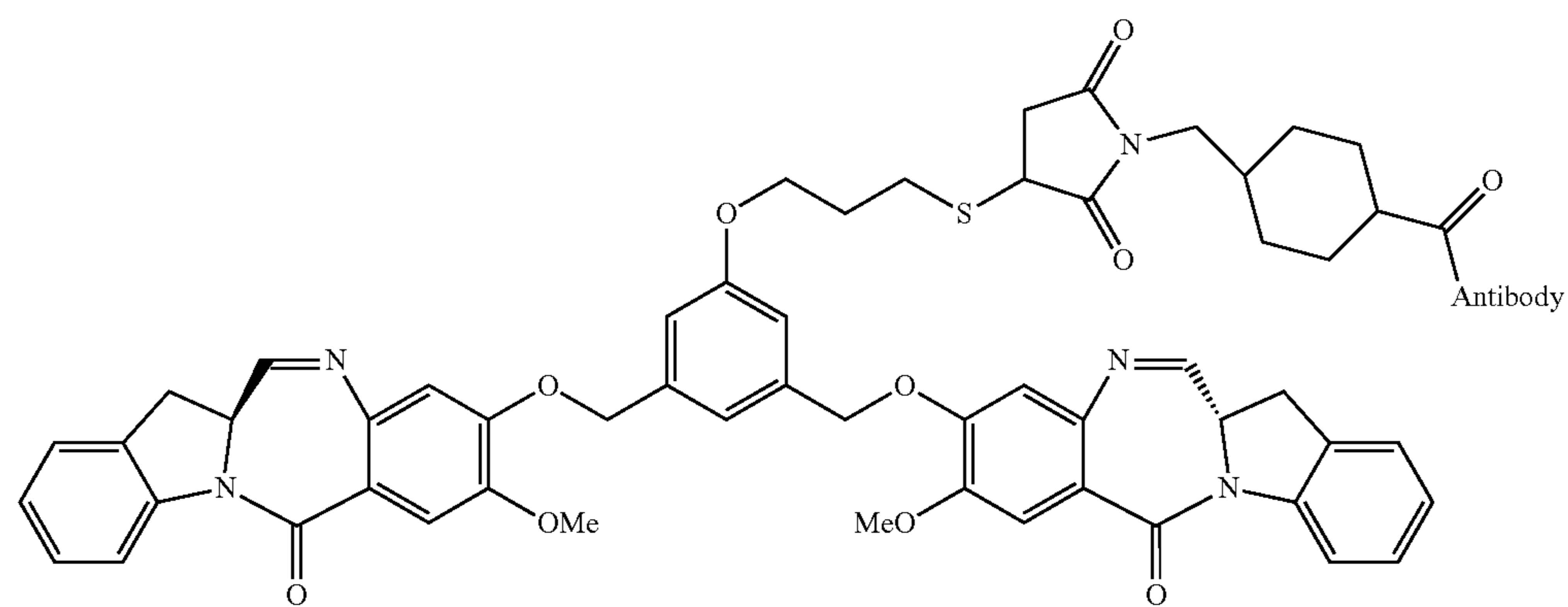
Dimer 3
