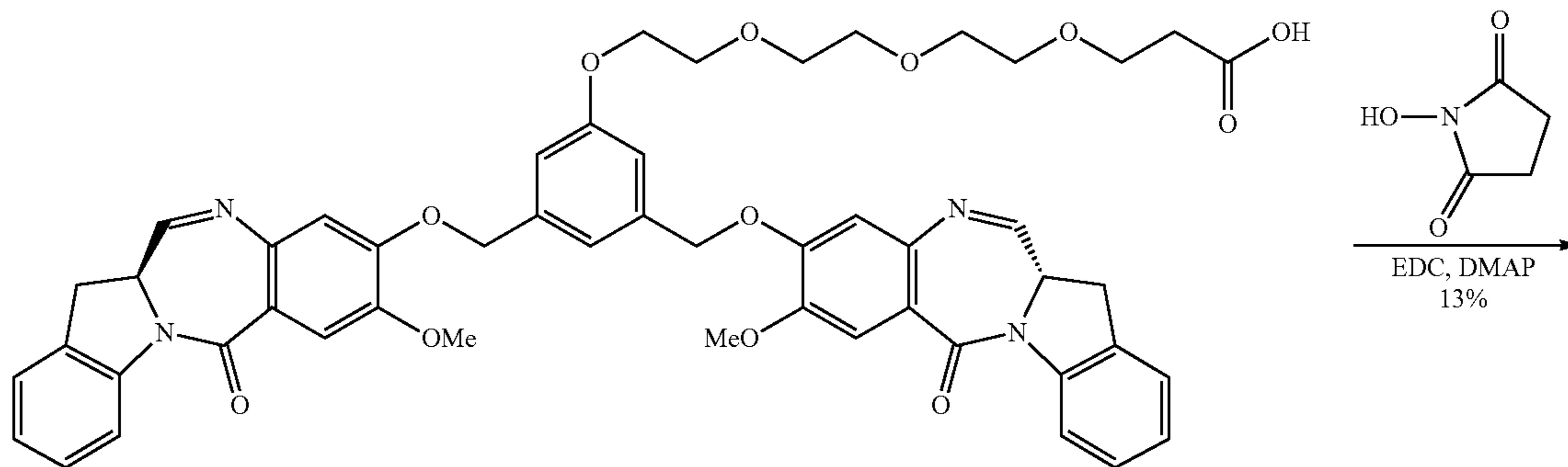
263d
