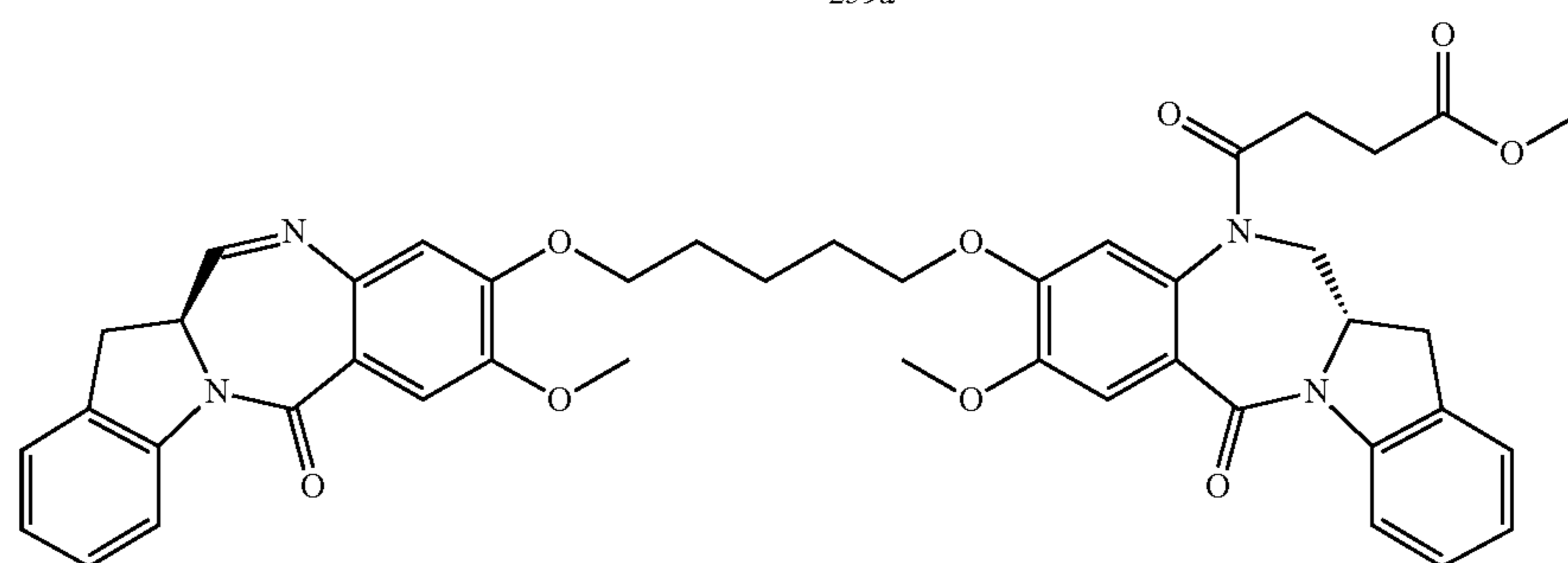
260c
