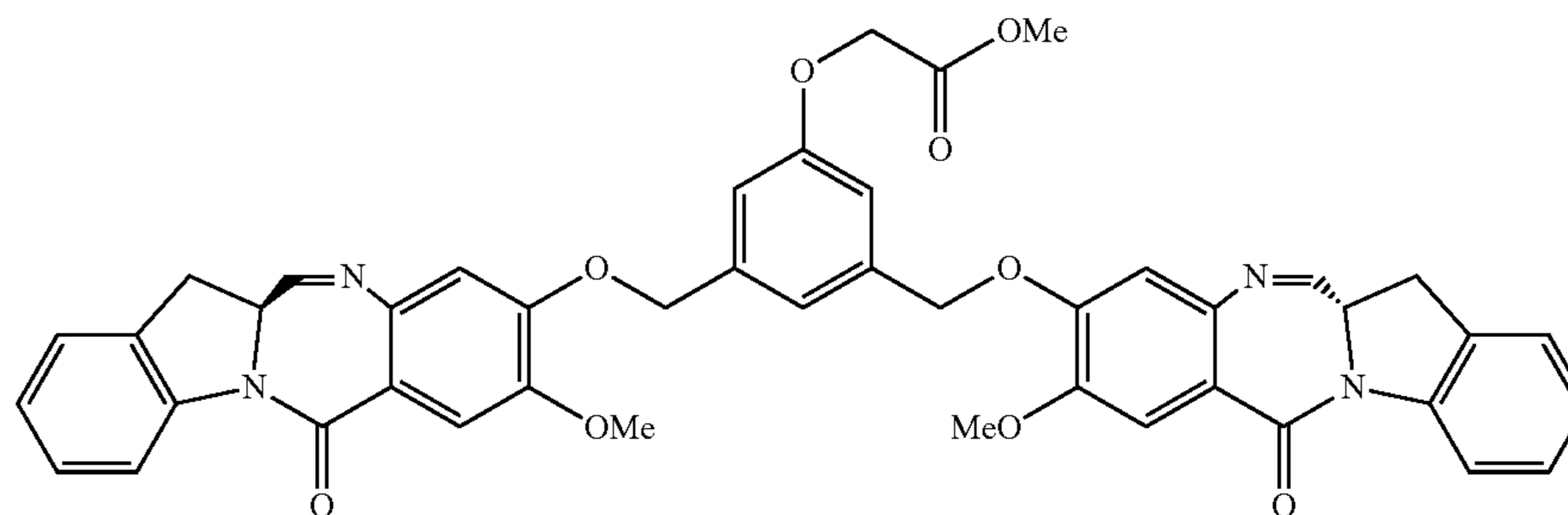
36 (IGN-05)
