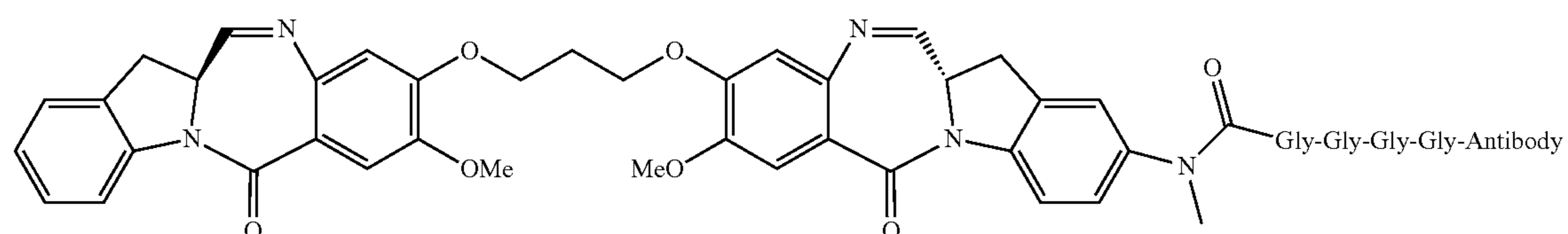
Dimer 5
