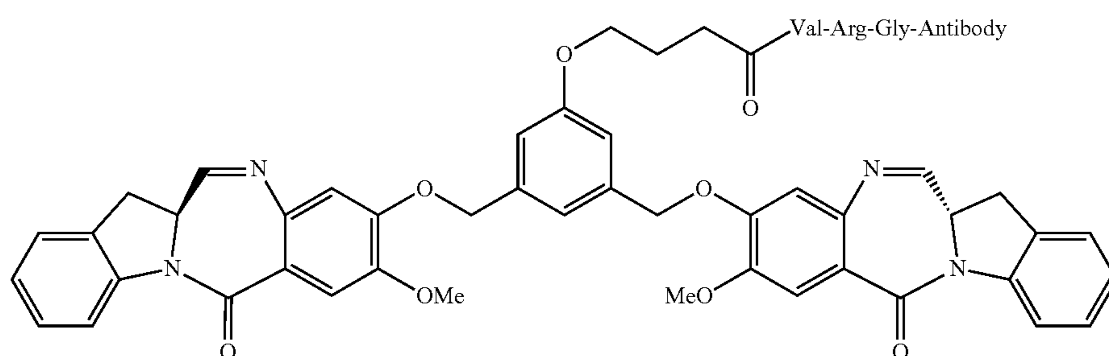
Dimer 2
