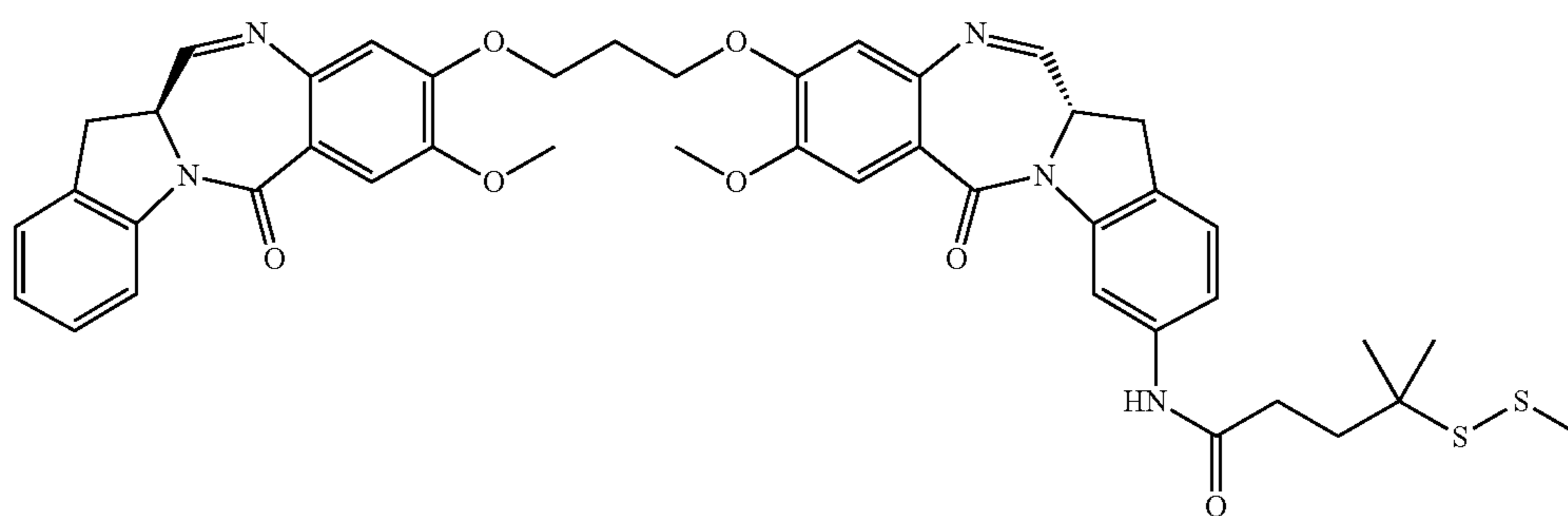
258h
