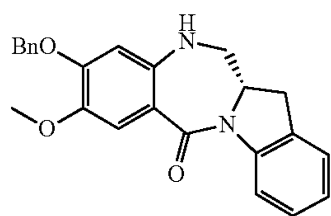
256a
