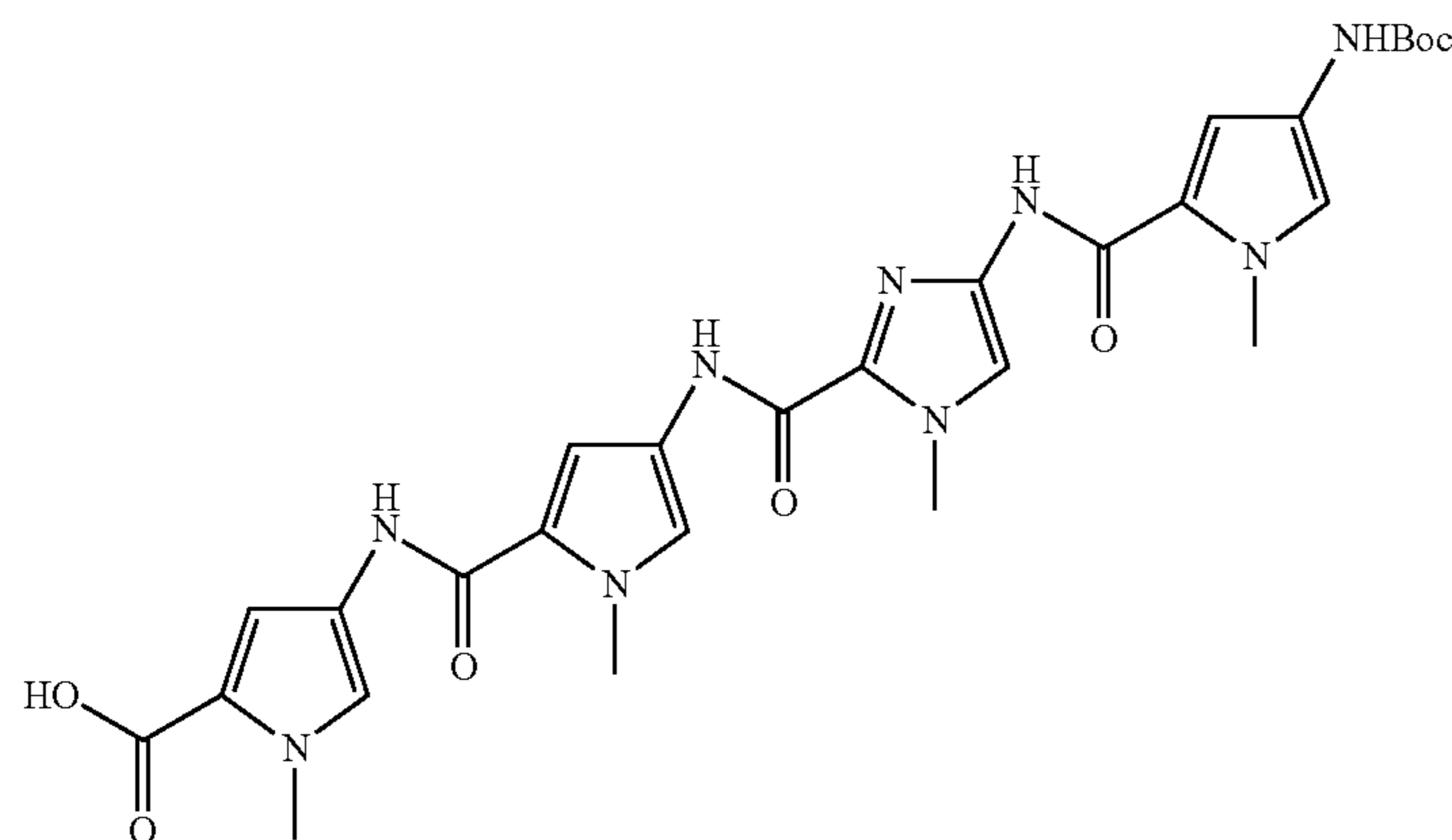
123
