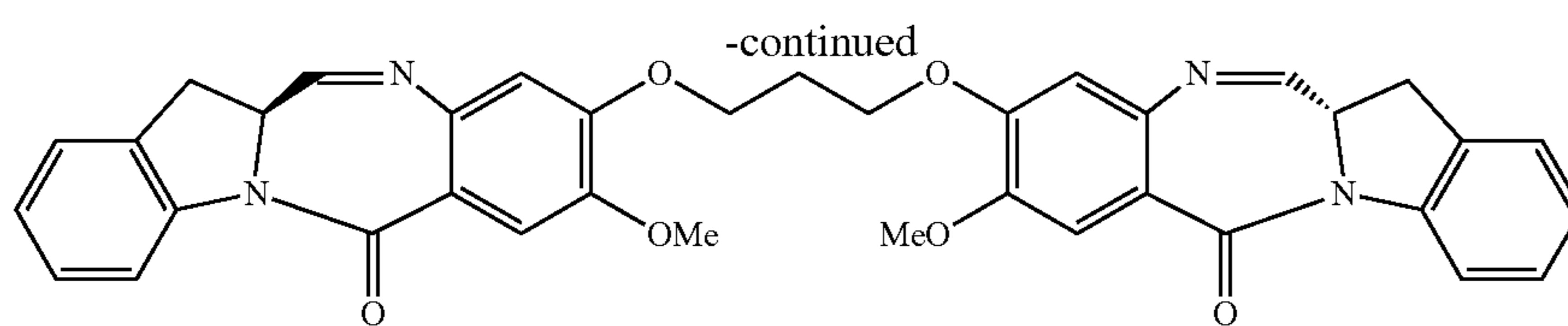
15 (IGN-09)
