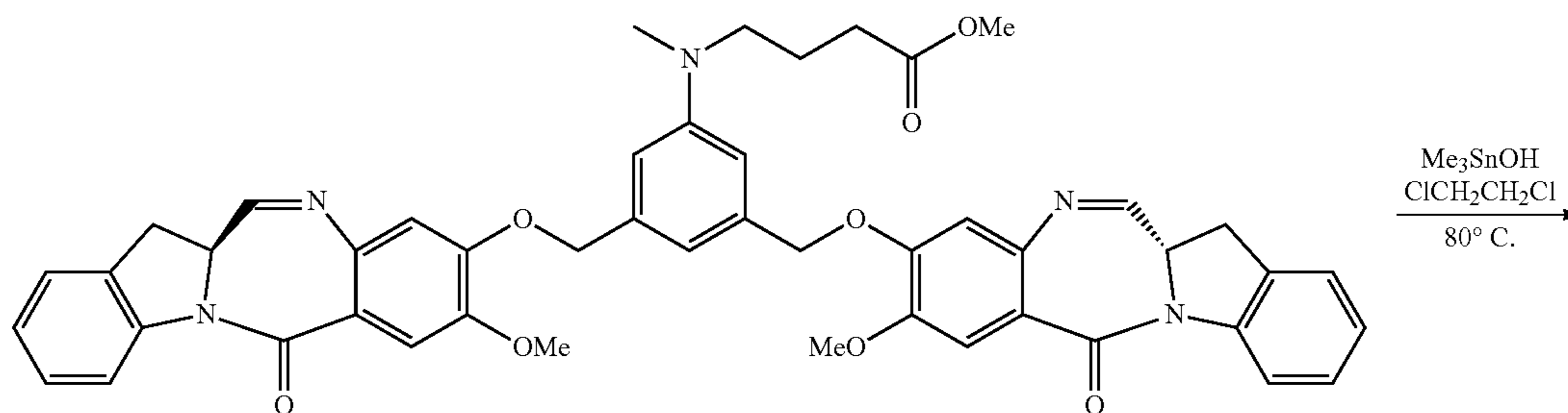
40 (IGN-07)
