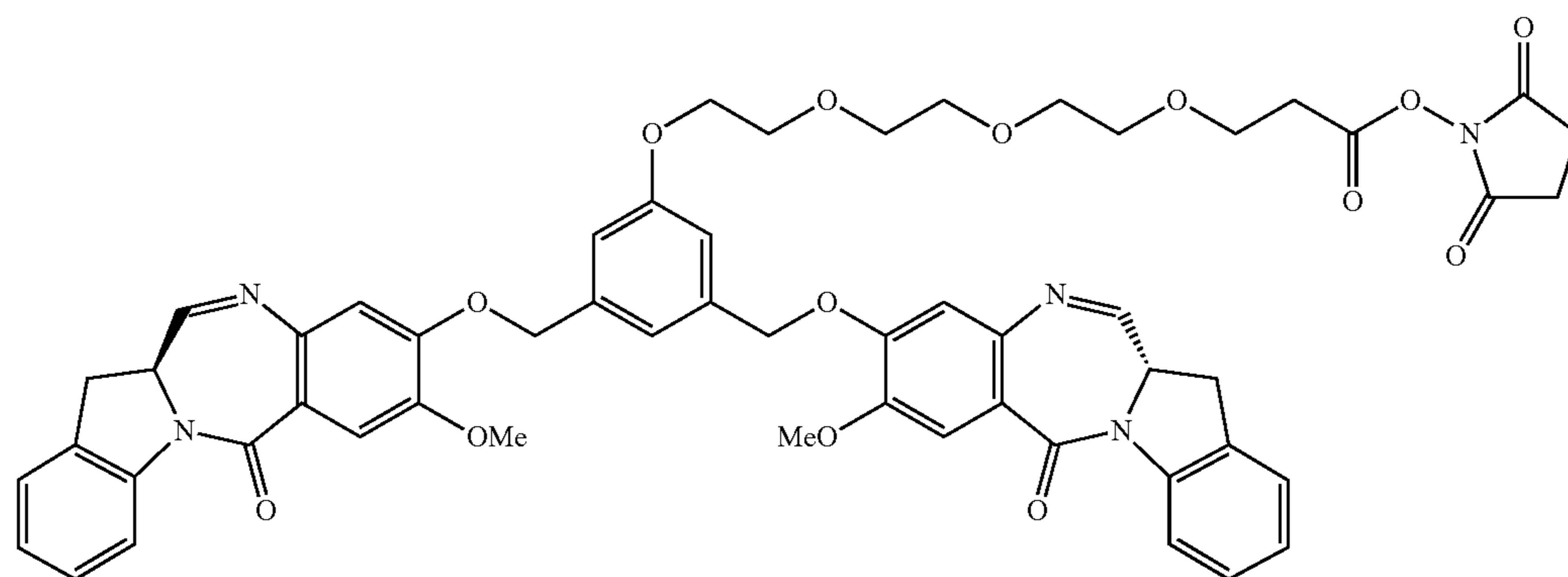
263e
