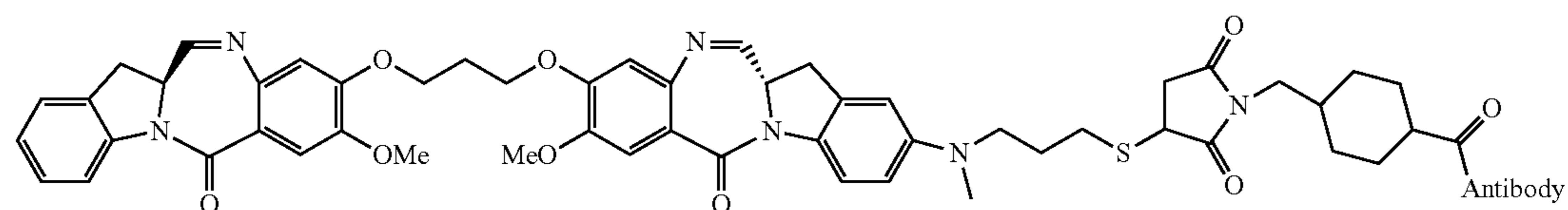
Dimer 7
