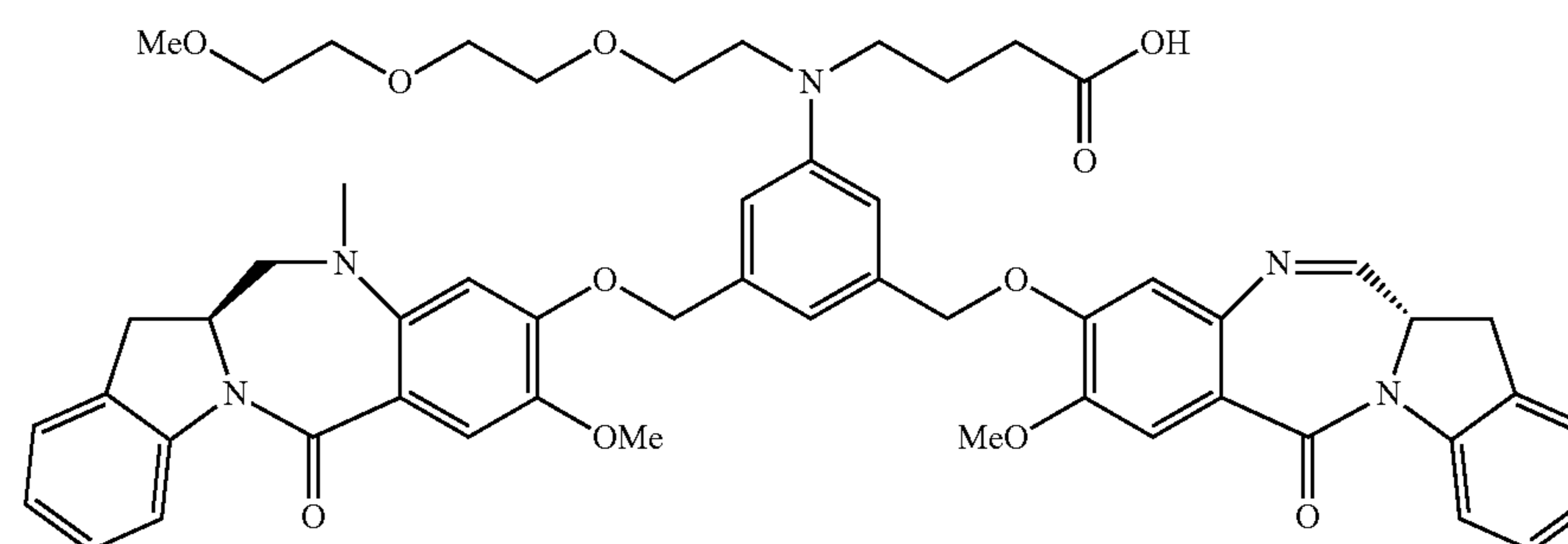
256f
