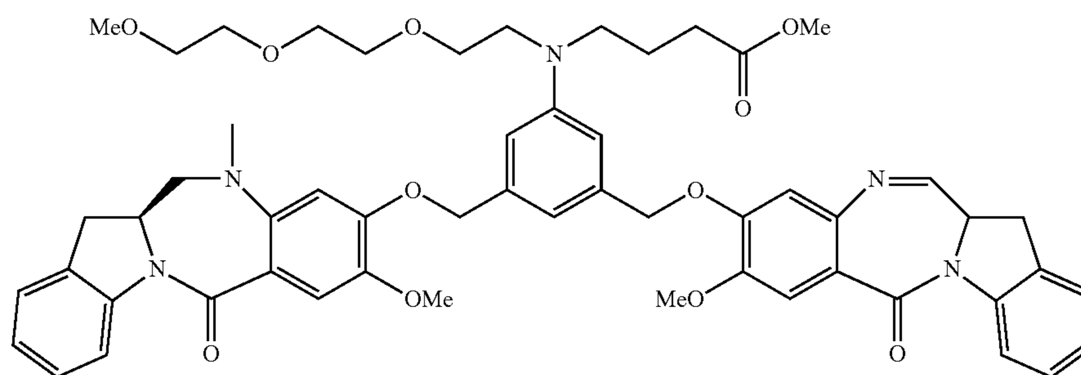
256d (IGN-29-OMe)
