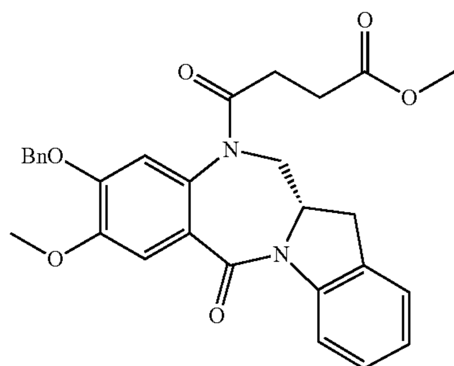
260a
