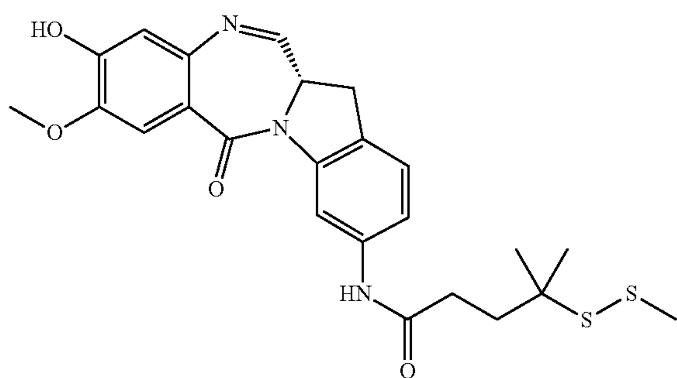
258f
