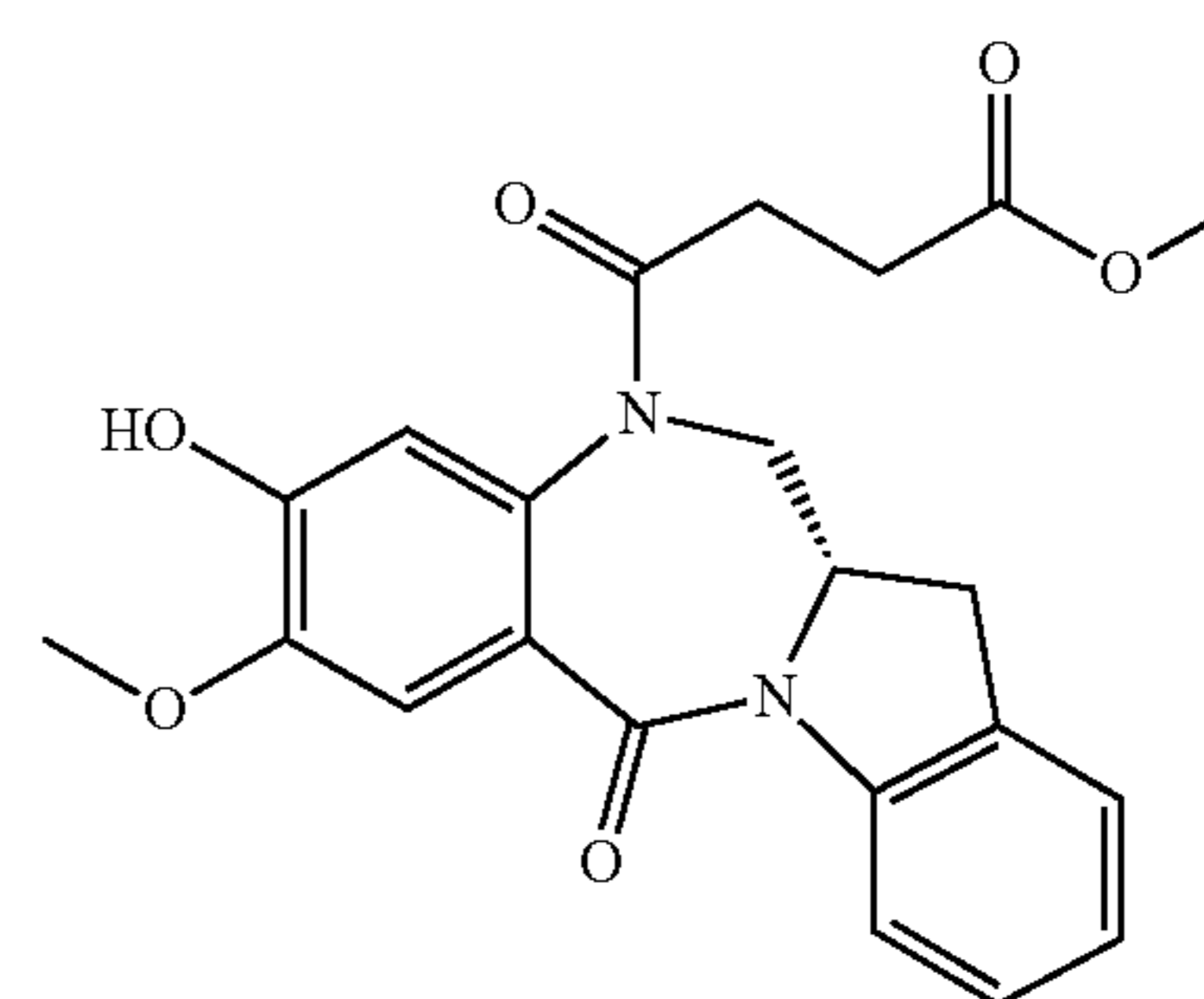
260b
