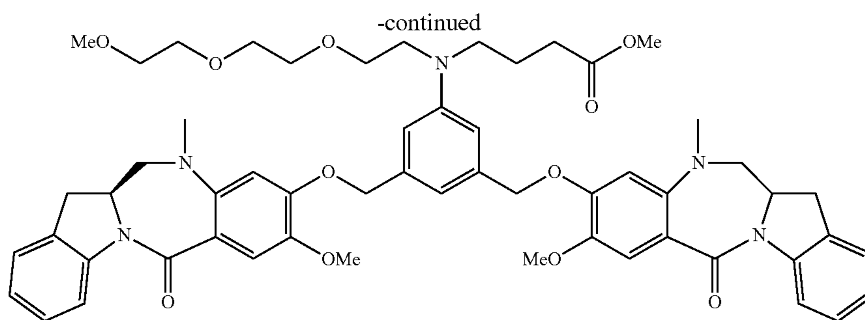
256e
