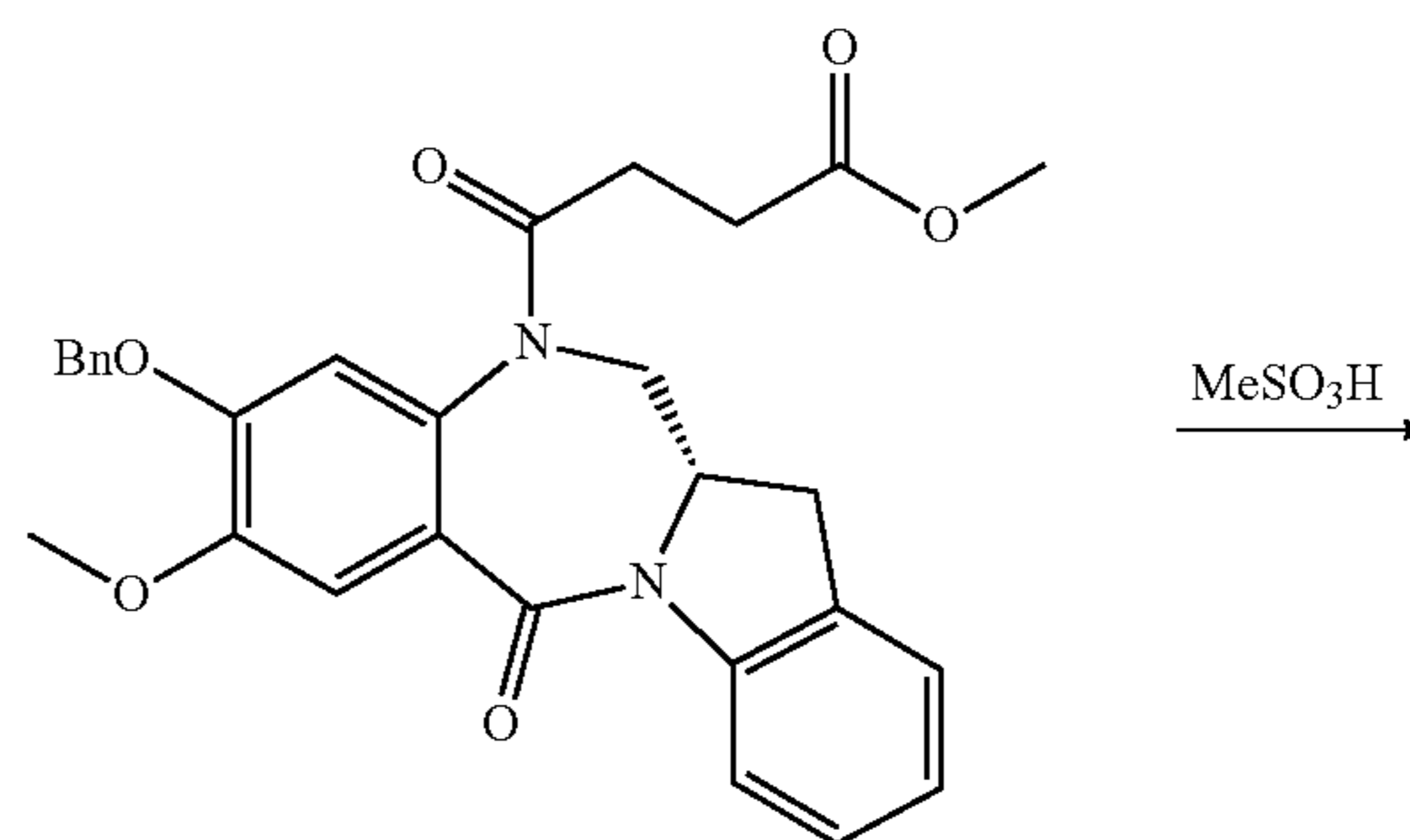
260a
