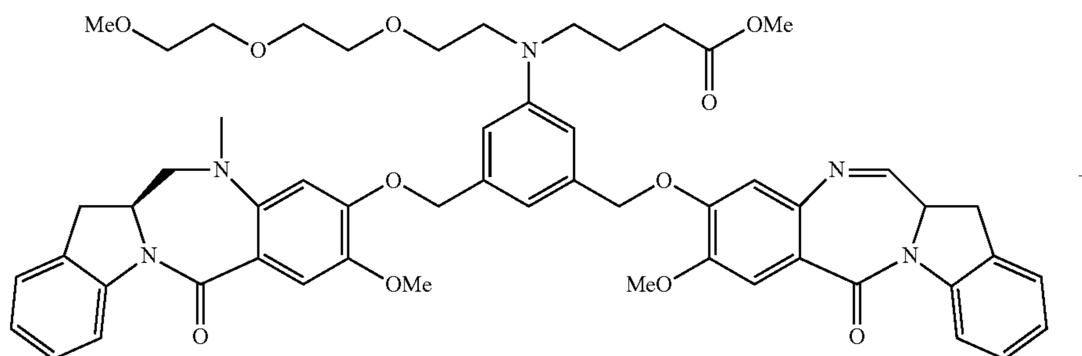
256d (IGN-29-OMe)
