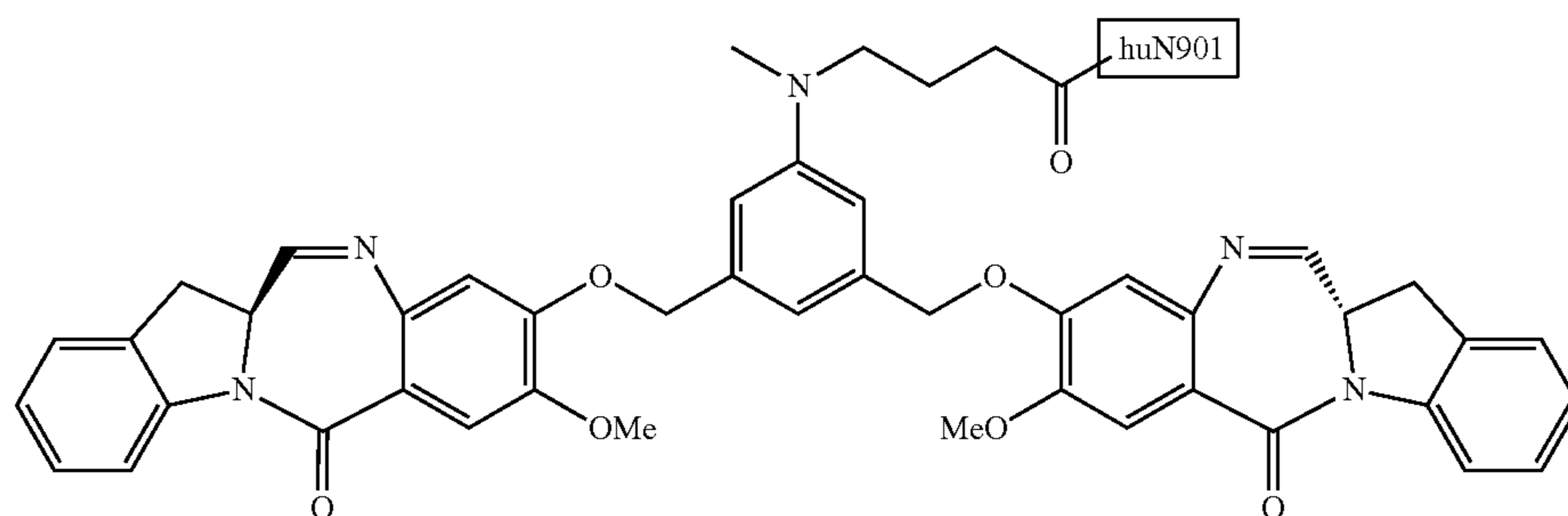
huN901-IGN-07
