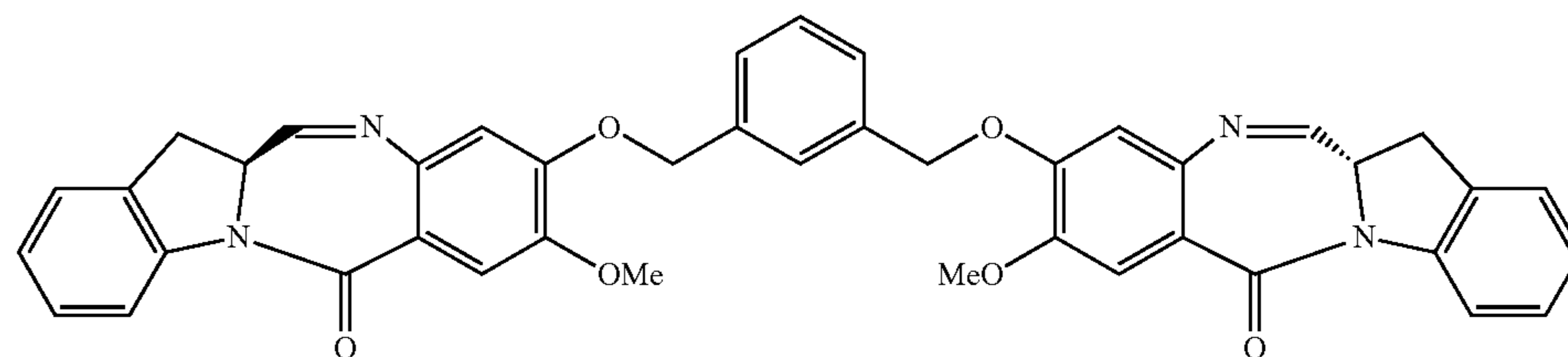
18 (IGN-01)
