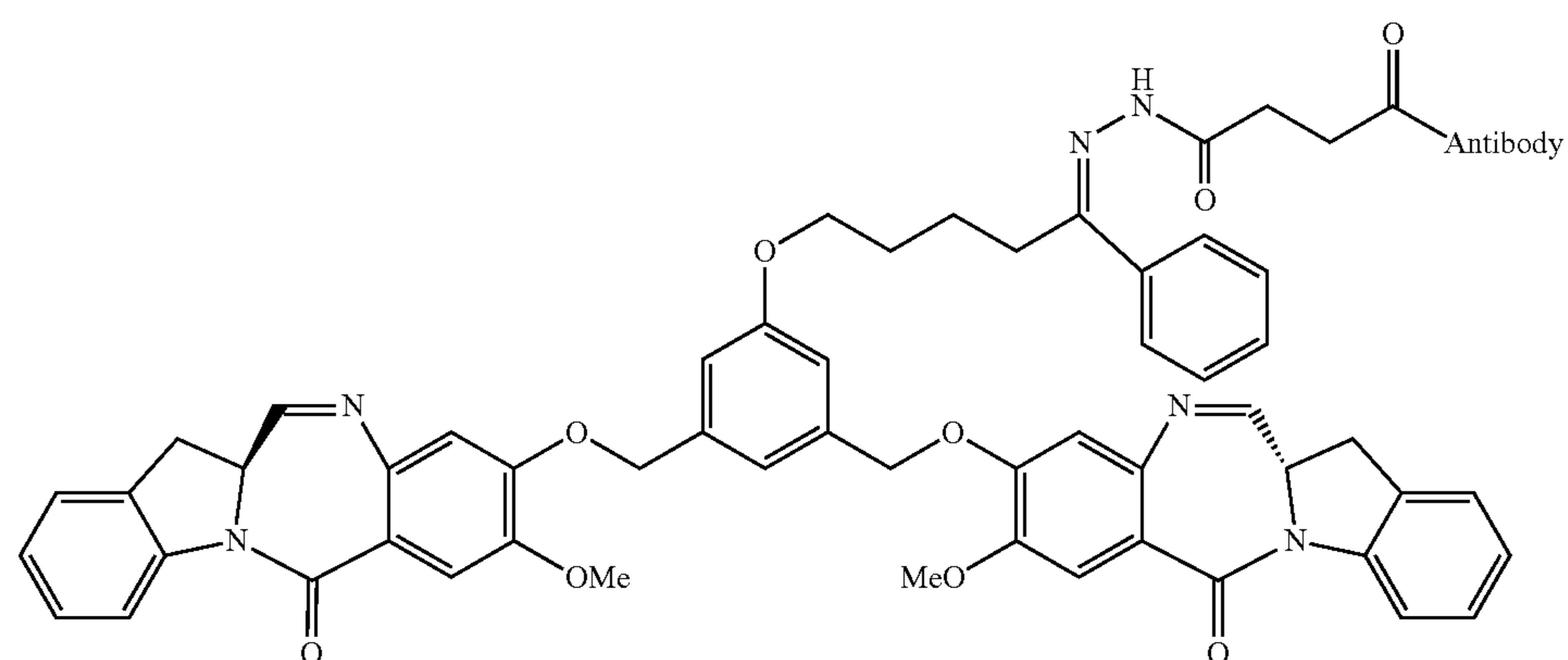
Dimer 4
