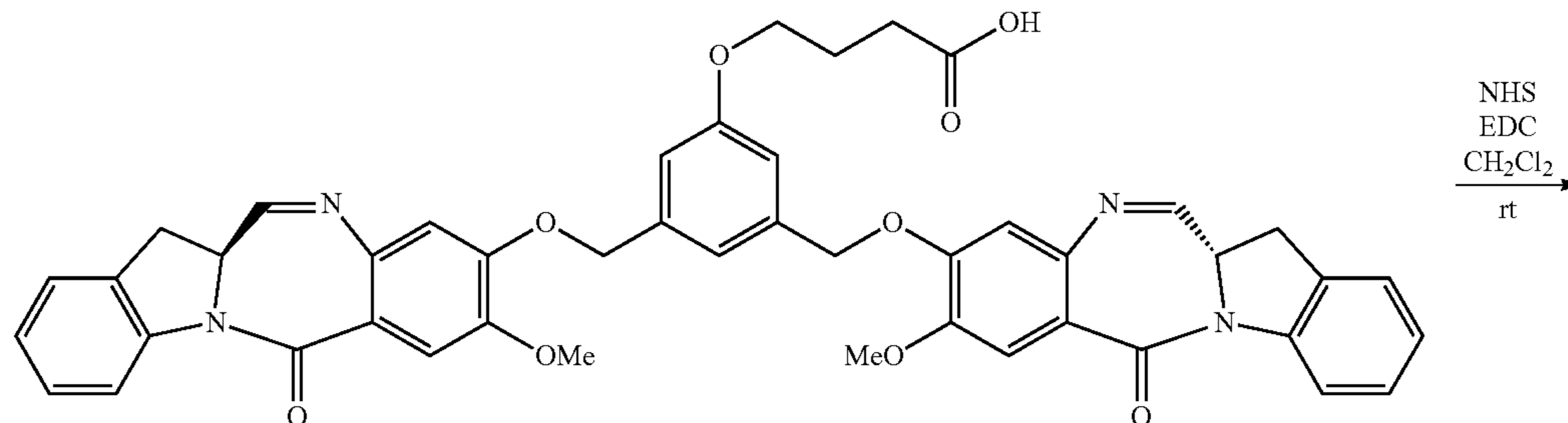
42 (IGN-04 acid)
