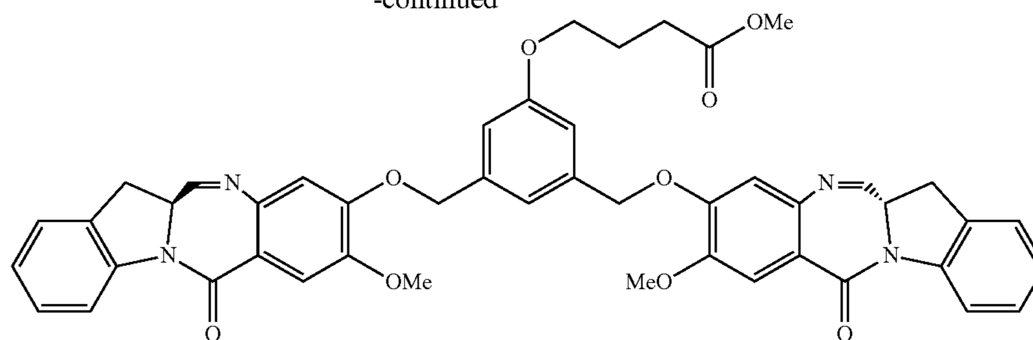
35 (IGN-04)
