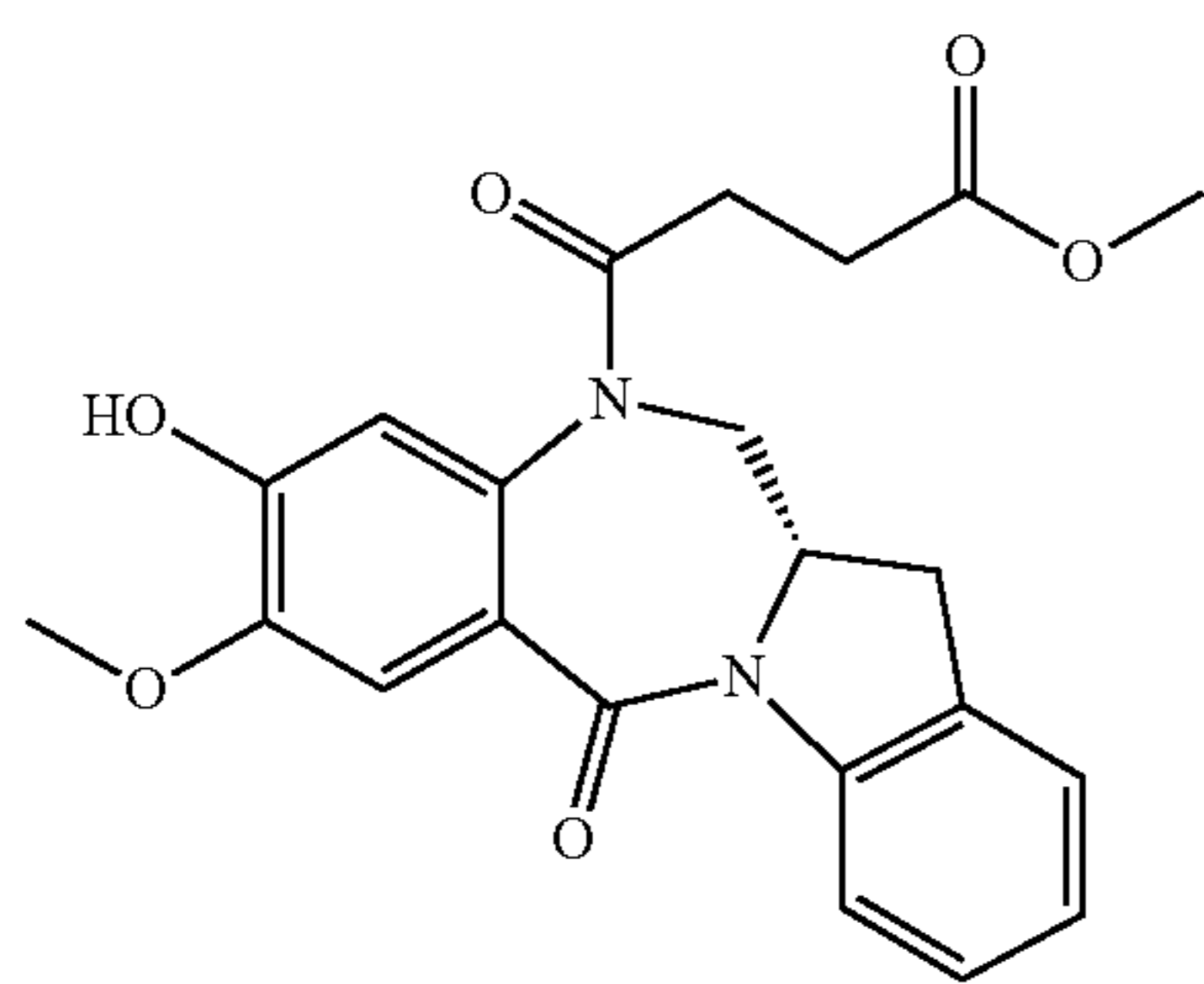
260b
