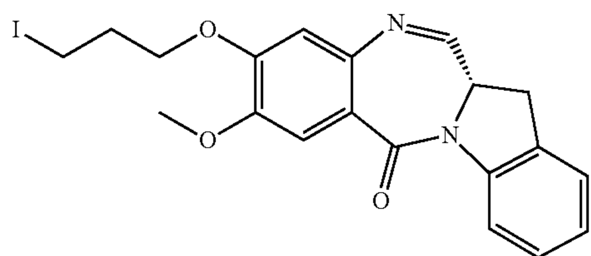
258g
