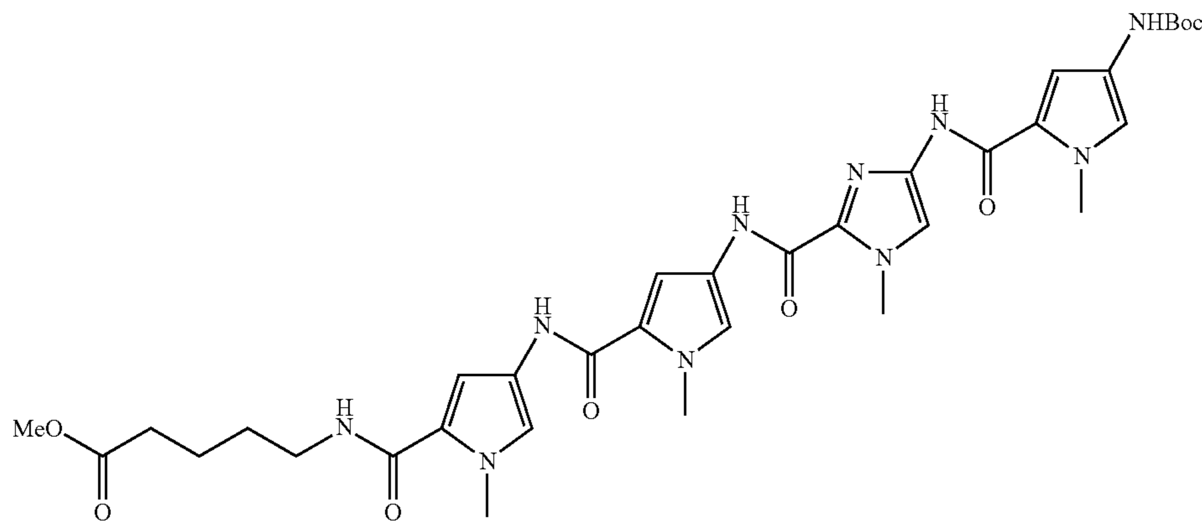
124
