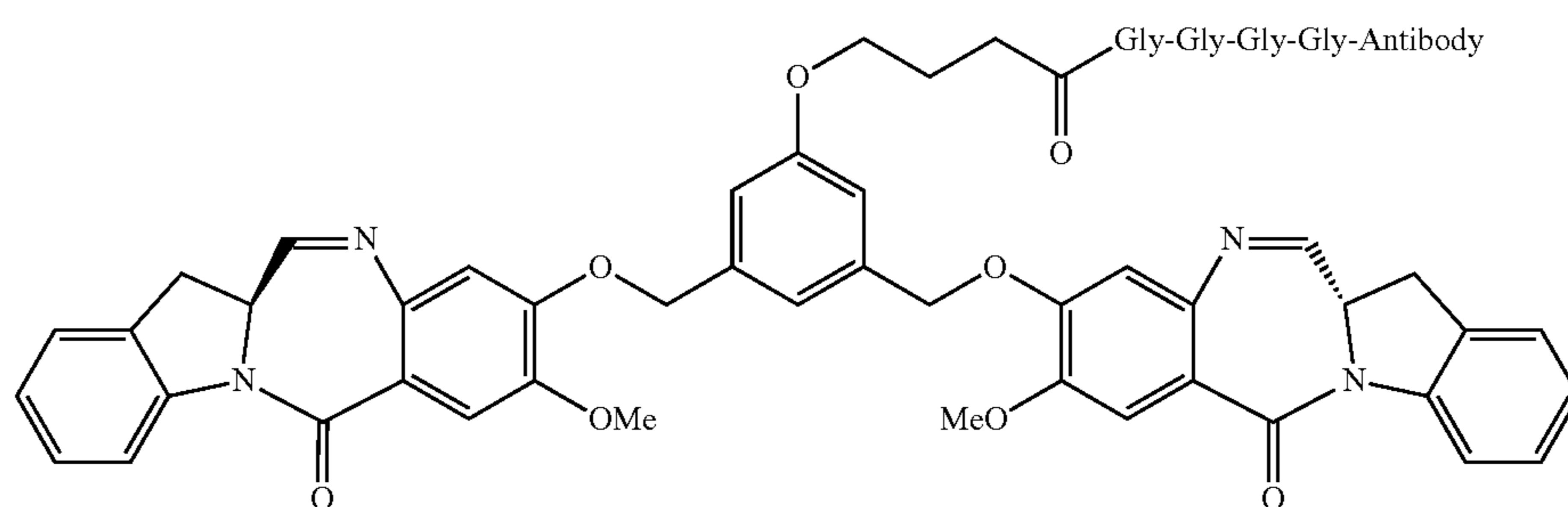
Dimer 1
