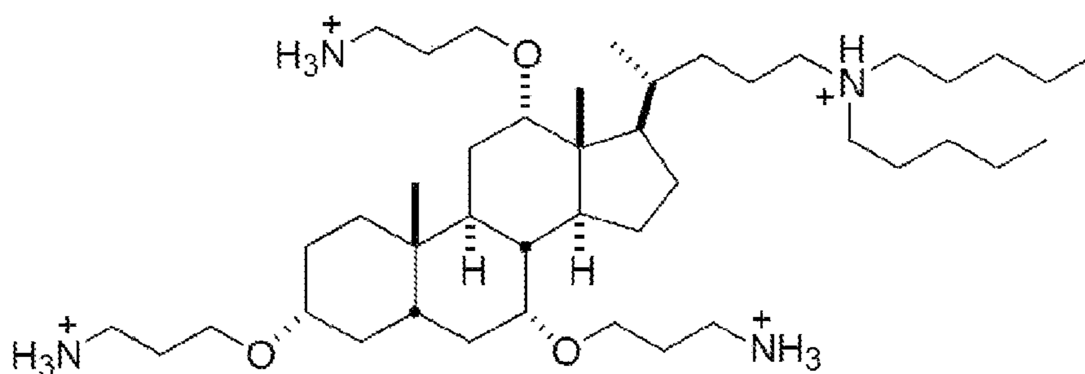
CSA-90 CLogP: 6.0858
