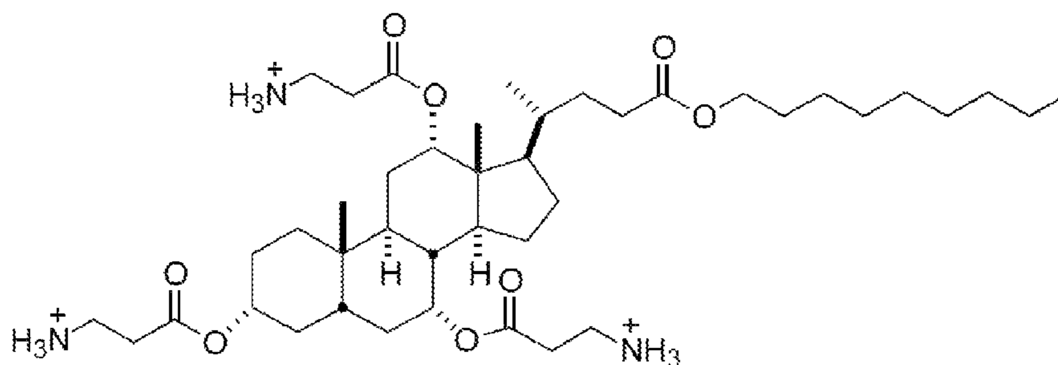
CSA-145 CLogP: 6.88
