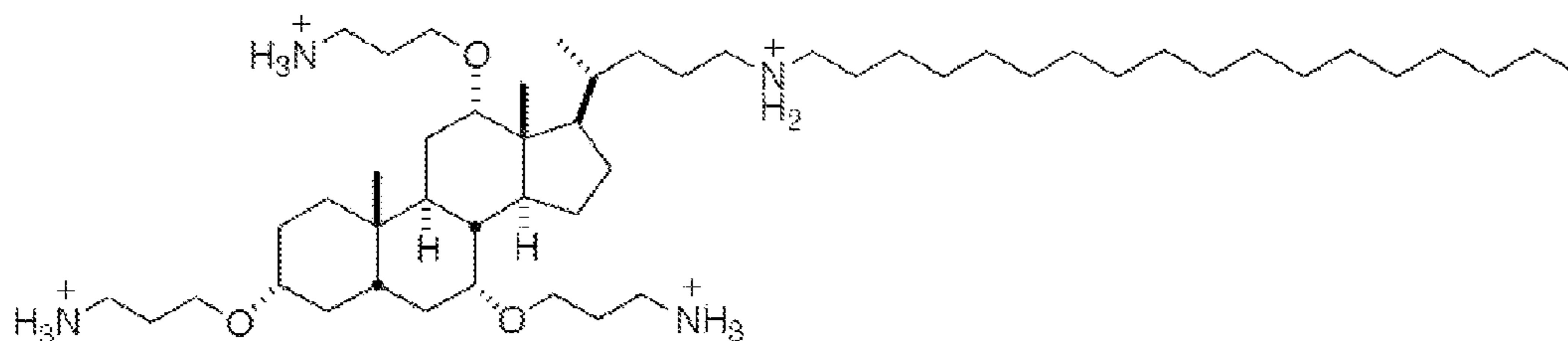
CSA-132 CLogP: 10.518
