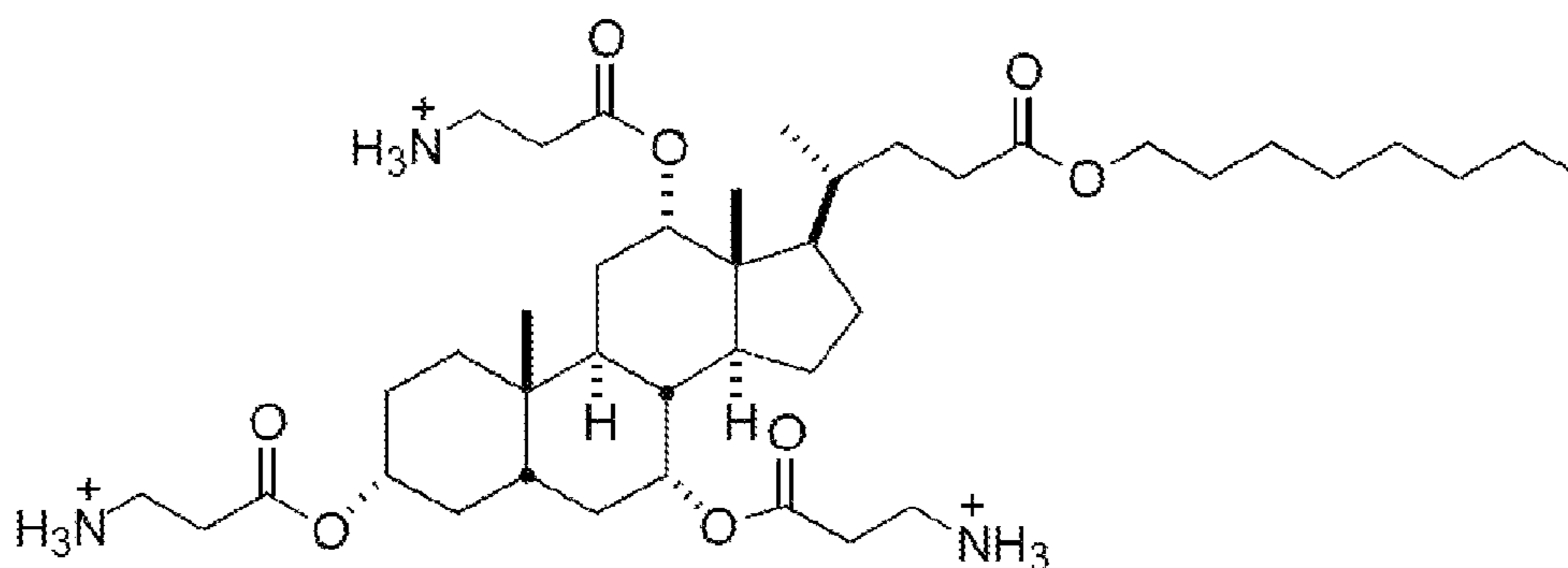
CSA-44 CLogP: 6.351
