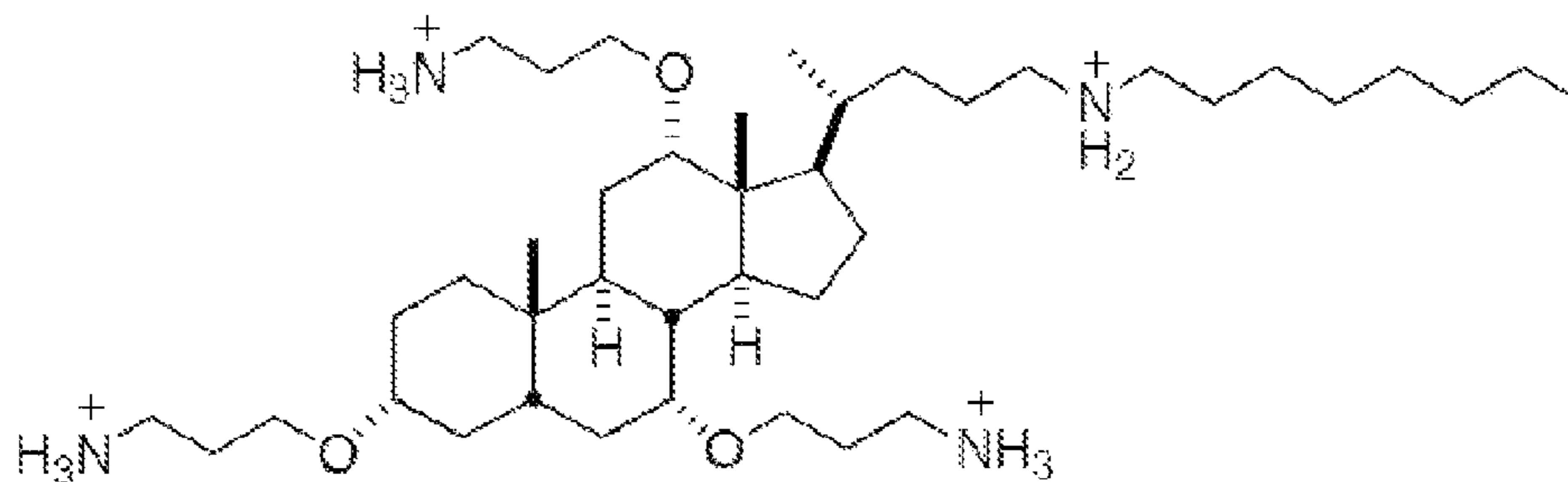
CSA-13 CLogP: 5.228
