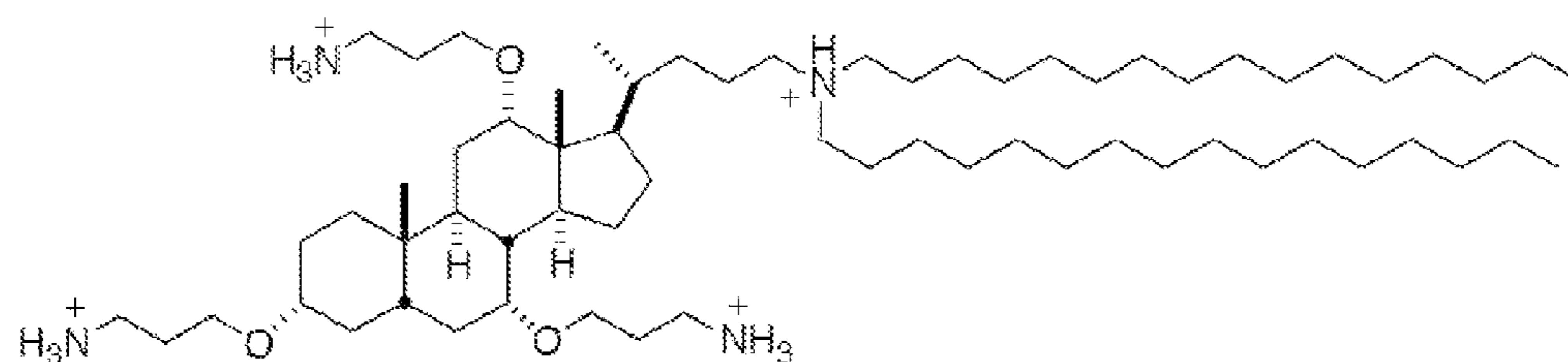
CSA-133 CLogP: 17.7238
