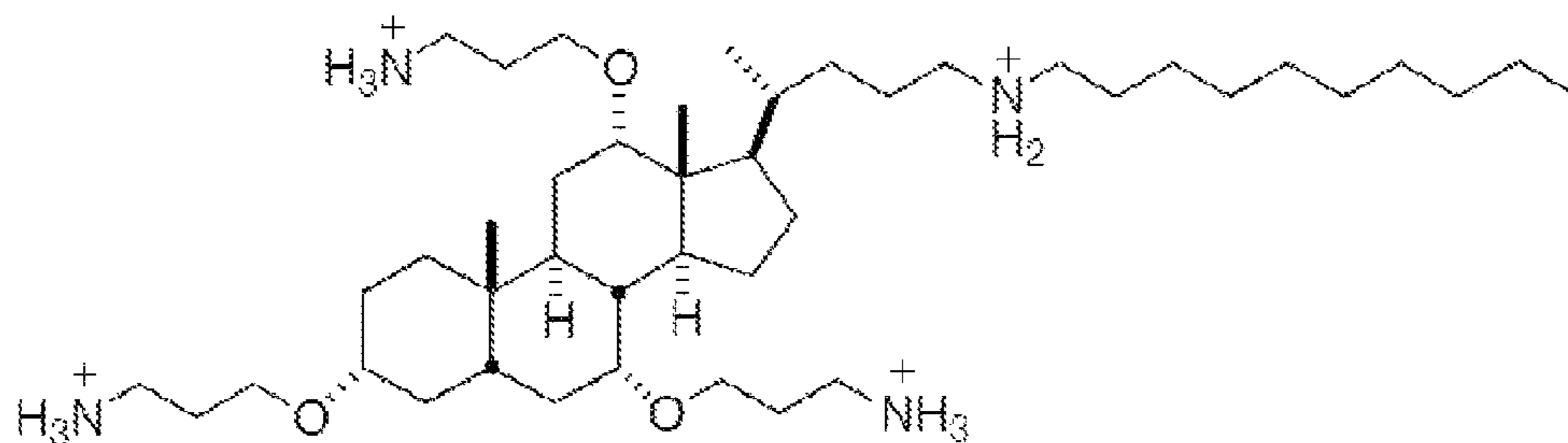
CSA-136 CLogP: 6.286
