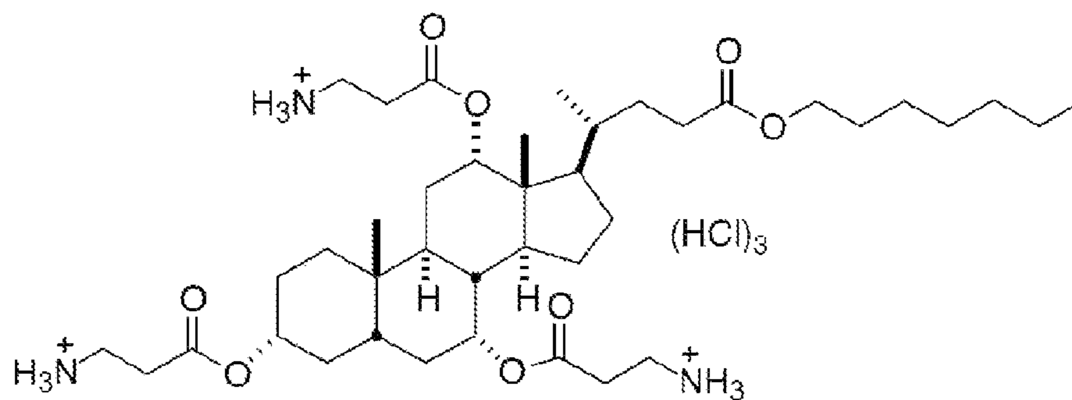
CSA-146 CLogP: 5.822
