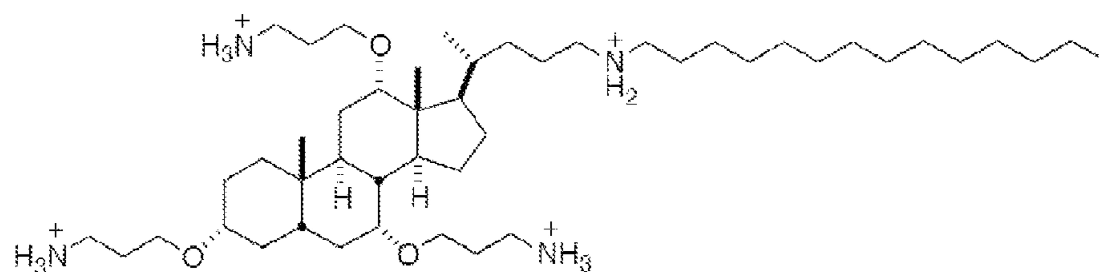
CSA-134 CLogP: 8.402
