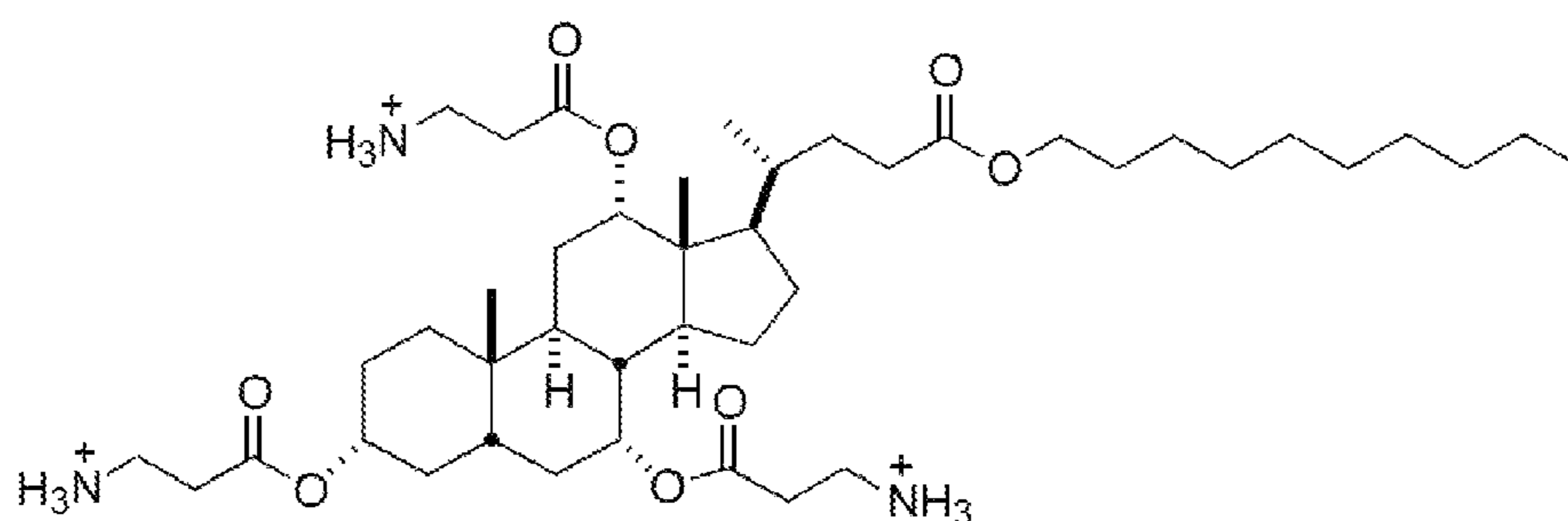
CSA-144 CLogP: 7.409
