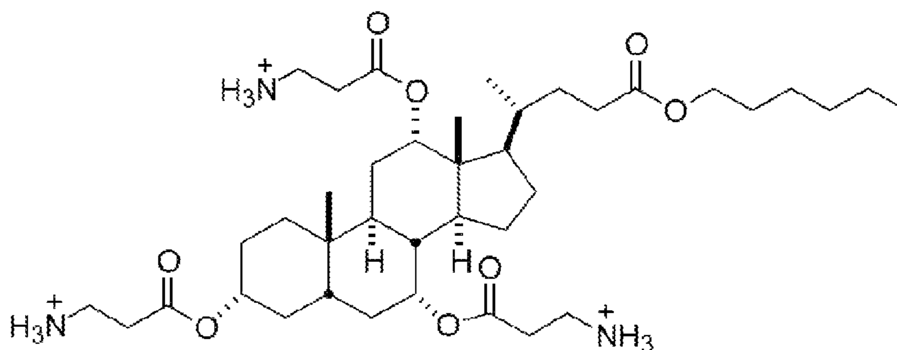
CSA-142 CLogP: 5.293
