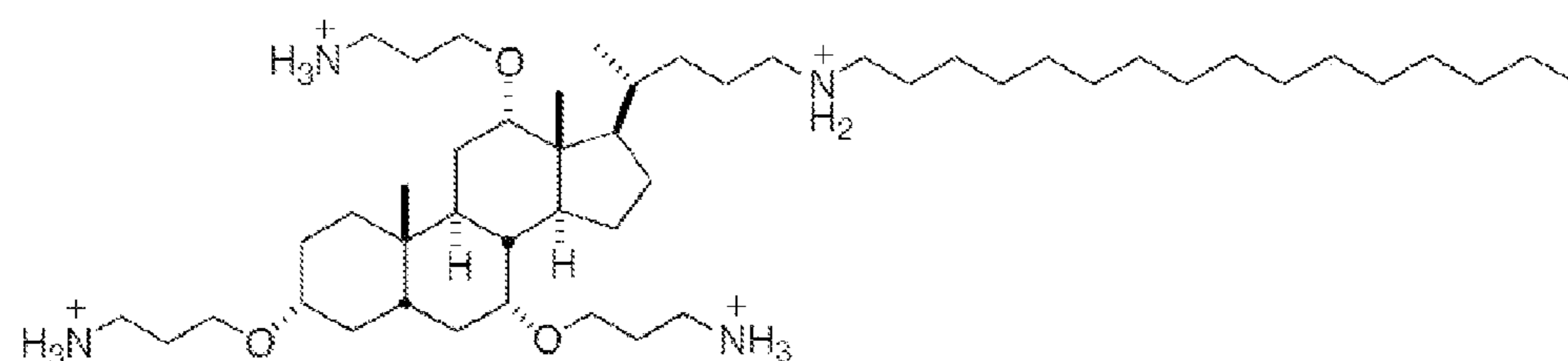
CSA-135 CLogP: 9.46
