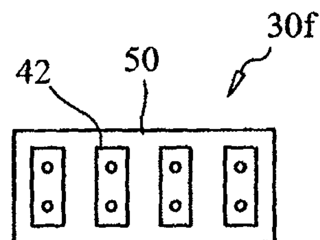
FIG. 1F
