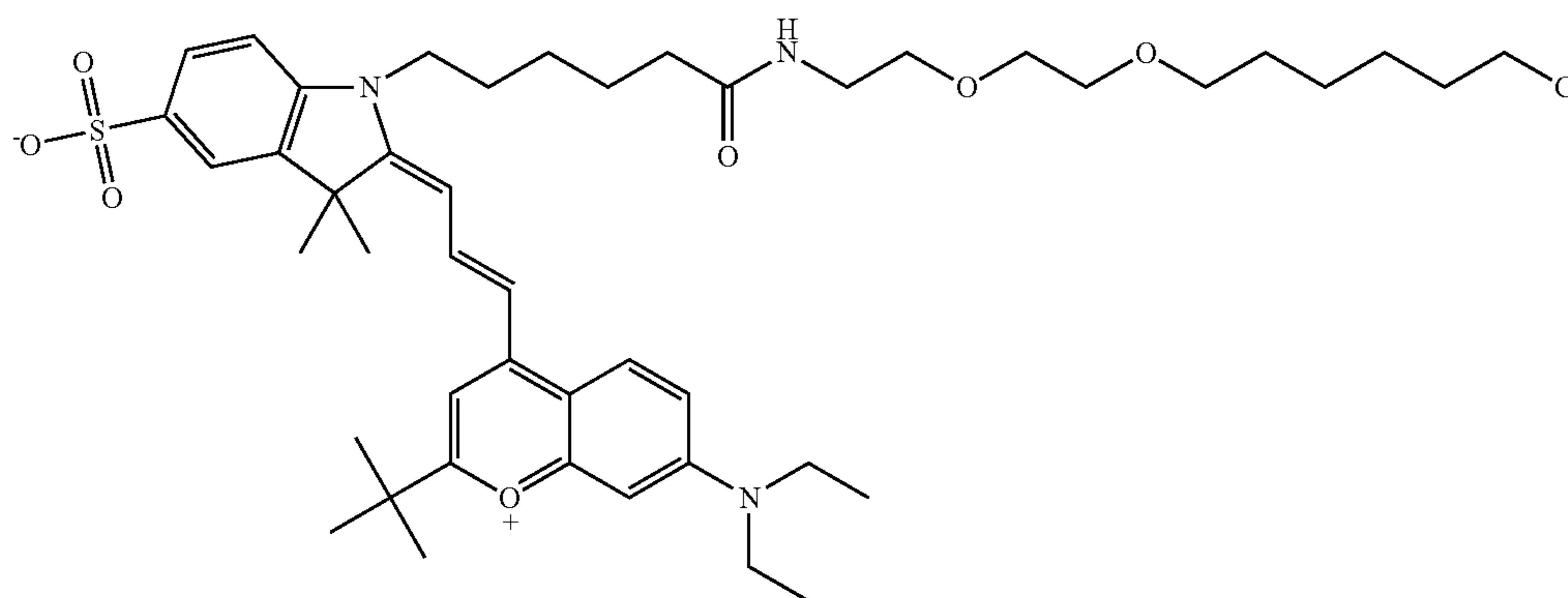
N-{2-[2-(6-Chlorohexyloxy)-ethoxy]-ethyl}-3-{4-[5-(4-dimethylamino-phenyl)-oxazol-2-yl]-benzene-sulfonylamino}-propionamide
