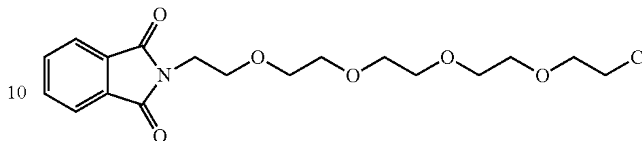
2-{2-[2-(2-{2-[2-(2-Chloroethoxy)-ethoxy]-ethoxy]-ethoxy}-ethyl)-isoindole-1,3-dione
