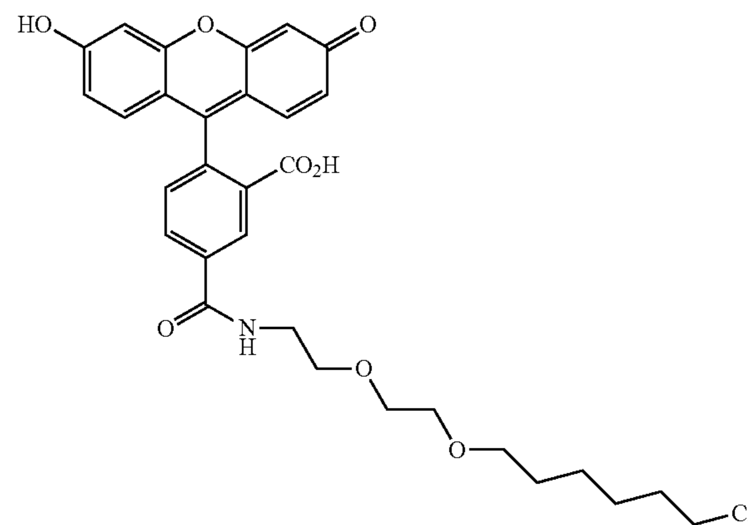
N-{2-[2-(6-Chlorohexyloxy)-ethoxy]-ethyl}-biotin-amide
