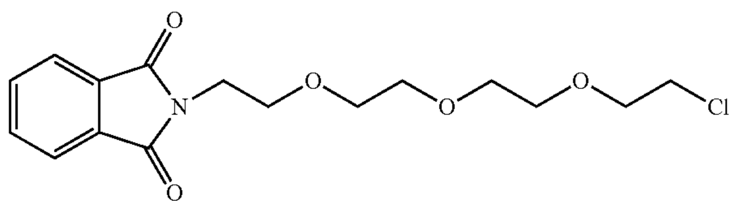
2-[2-(2-{2-[2-(2-Chloroethoxy)-ethoxy]-ethoxy}-ethyl)-isoindole-1,3-dione
