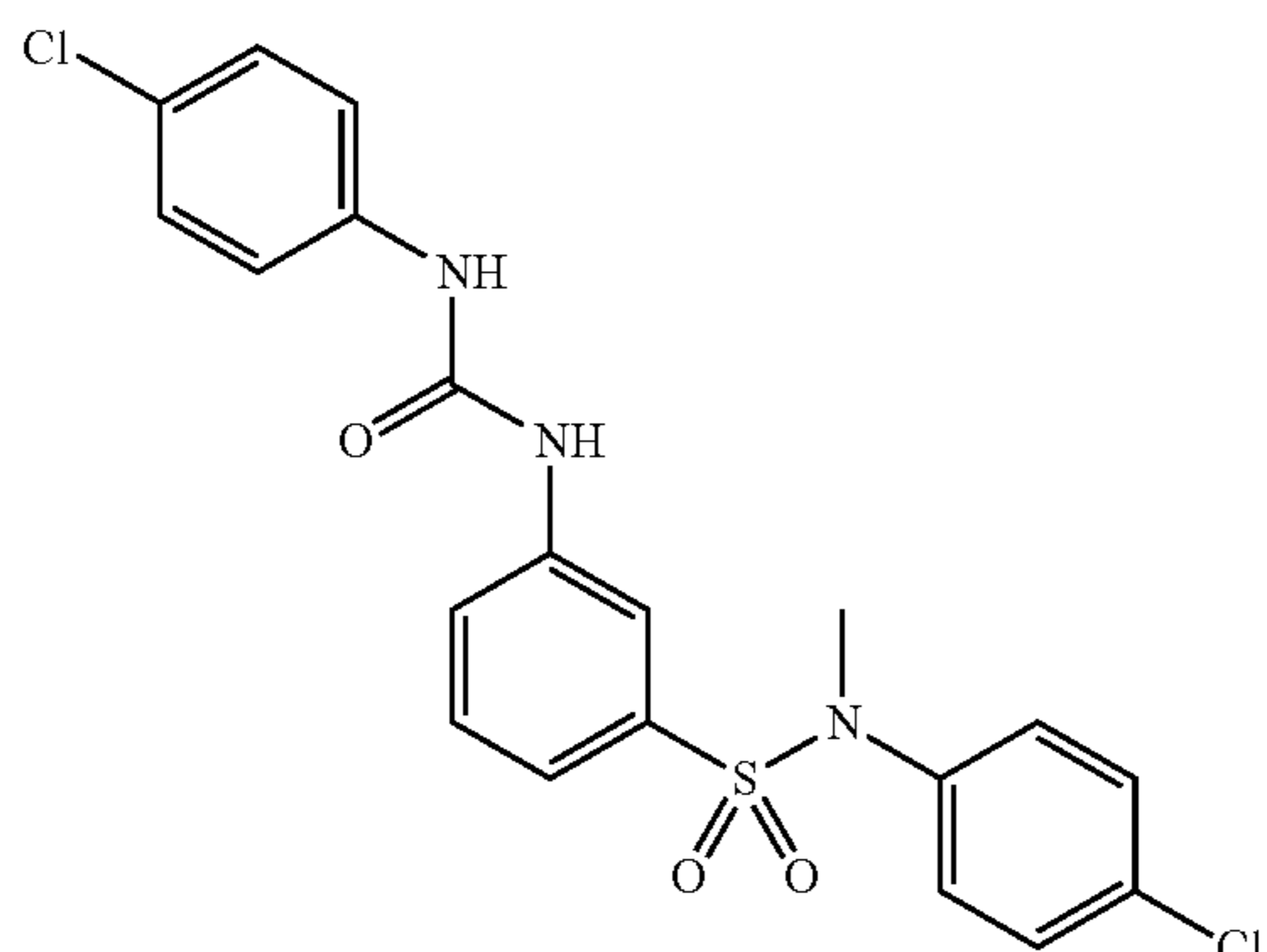
N-(4-chlorophenyl)-3-(3-(4-chlorophenyl)ureido)-N-methylbenzenesulfonamide (233a)
