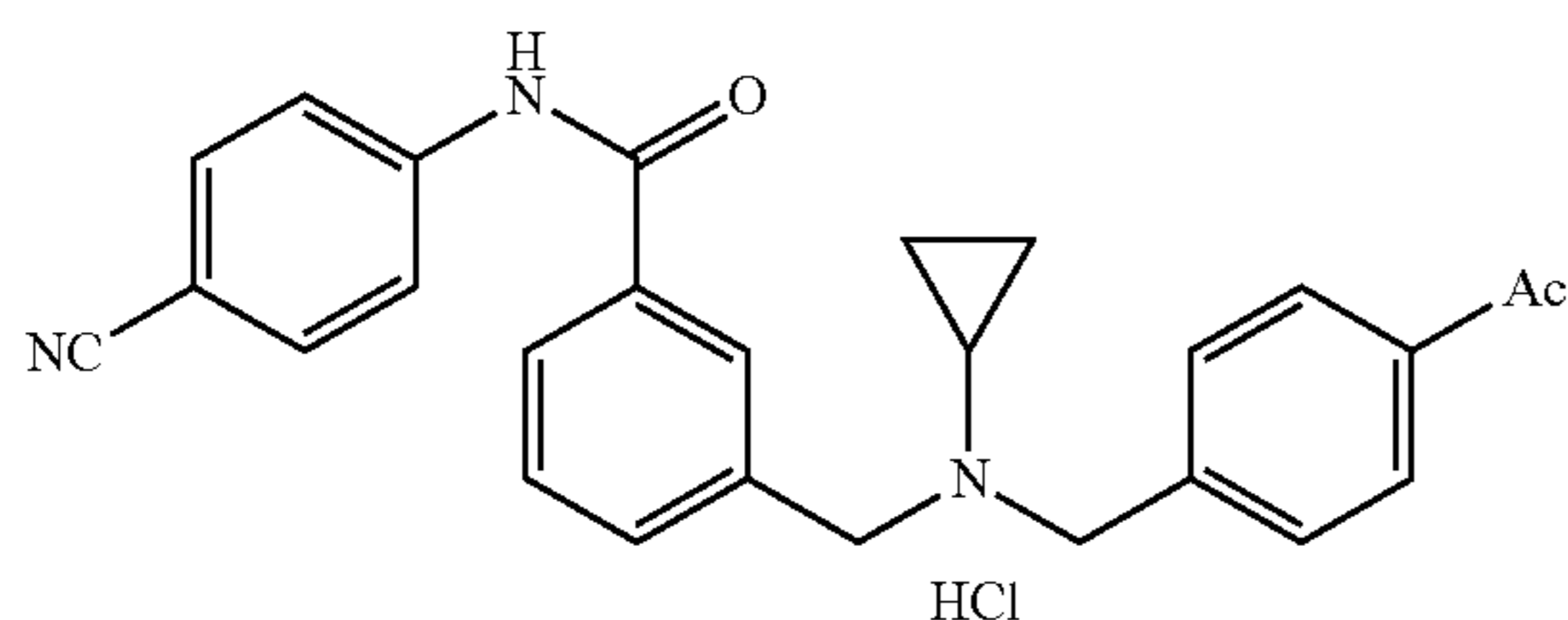
3-(((4-acetylbenzyl)(cyclopropyl)amino)methyl)-N-(4-cyanophenyl)benzamide hydrochloride (225x)
