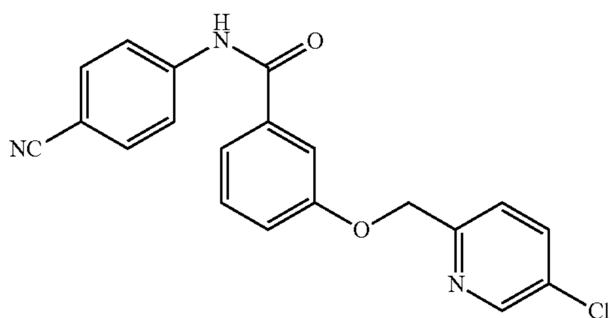
3-((5-chloropyridin-2-yl)methoxy)-N-(4-cyanophenyl)benzamide (216n)
