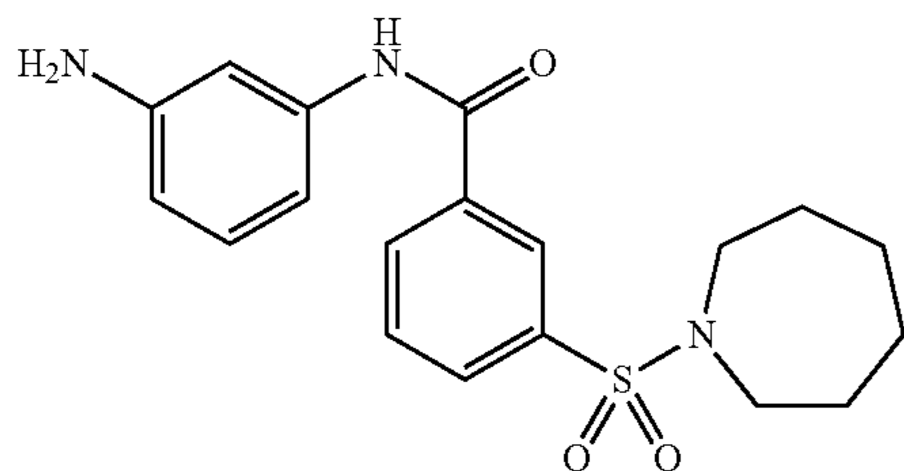
N-(3-aminophenyl)-3-(azepan-1-ylsulfonyl)benzamide (203i)
