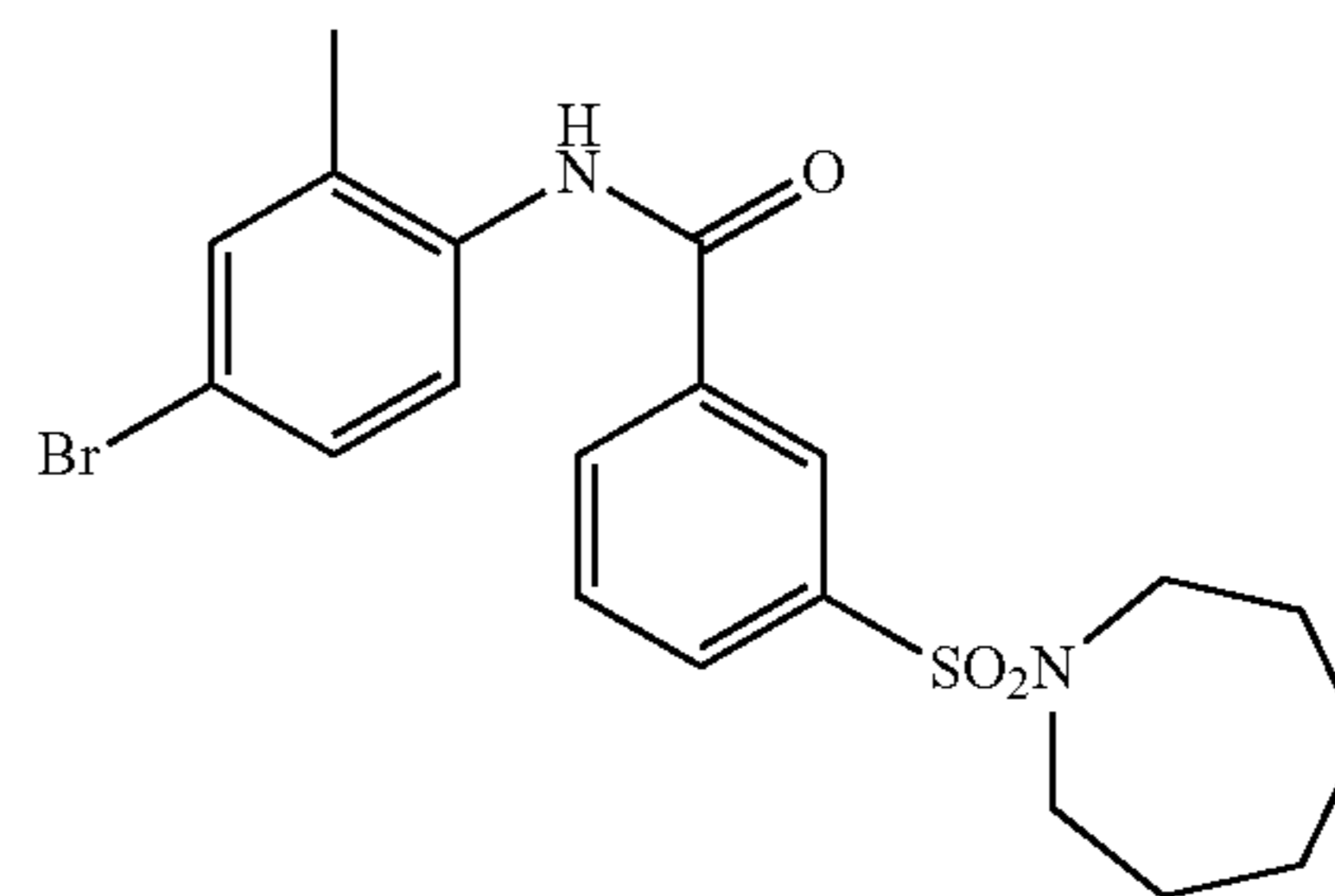
3-(azepan-1-ylsulfonyl)-N-(4-bromo-2-methylphenyl)benzamide (203b)
