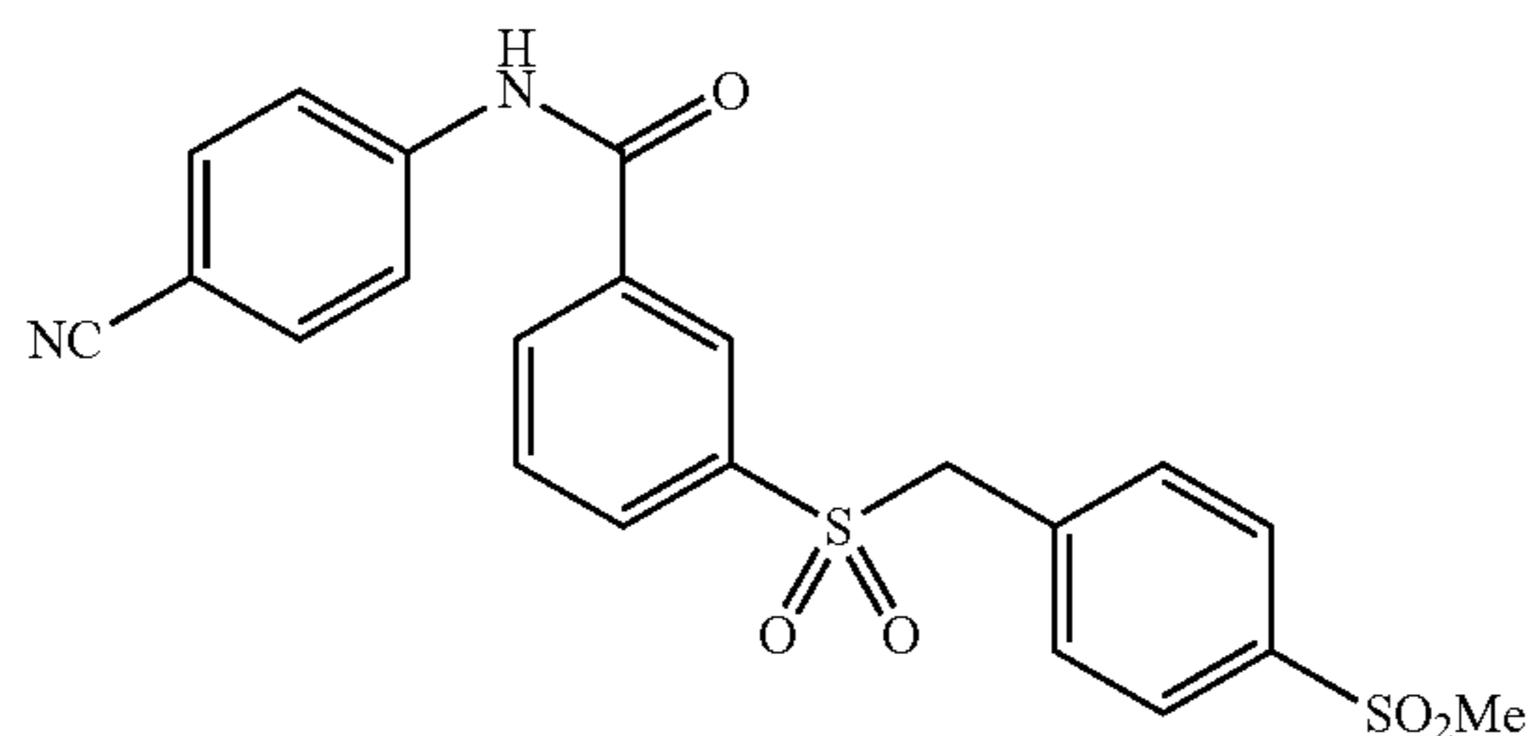
N-(4-cyanophenyl)-3-((4-(methylsulfonyl)benzyl)sulfonyl)benzamide (212a)
