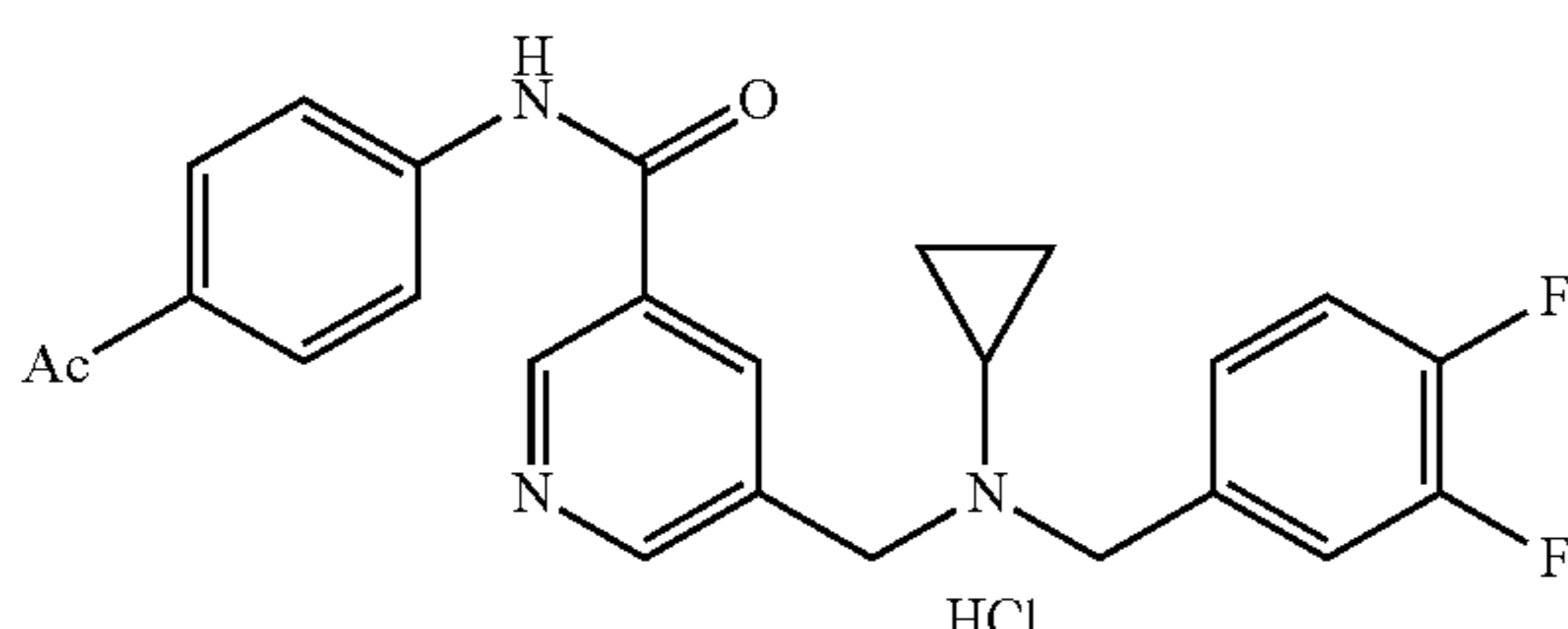
N-(4-acetylphenyl)-5-((cyclopropyl(3,4-difluorobenzyl)amino)methyl)nicotinamide hydrochloride (225u)
