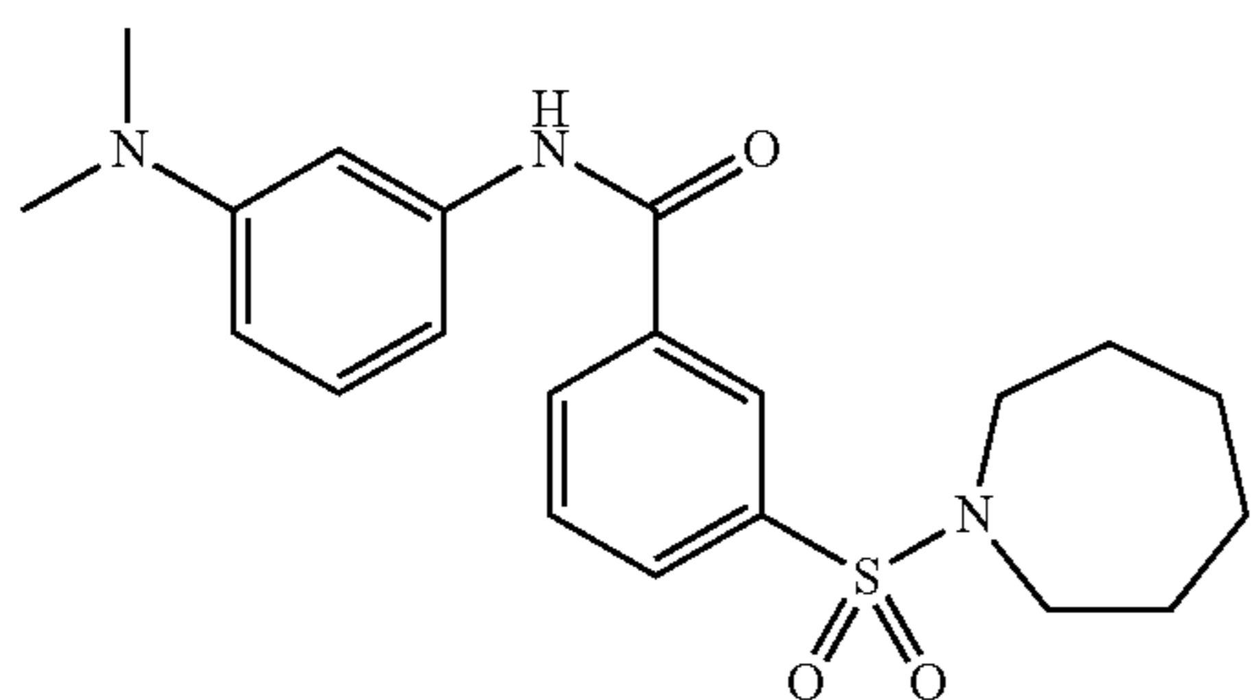
3-(azepan-1-ylsulfonyl)-N-(3-(dimethylamino)phenyl)benzamide (203j)
