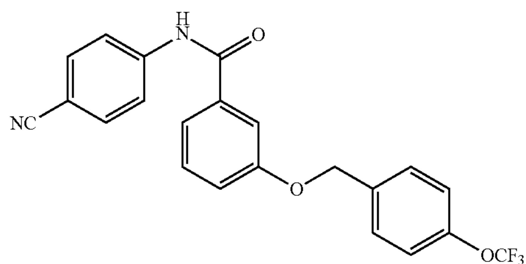
N-(4-cyanophenyl)-3-((4-(trifluoromethoxy)benzyl)oxy)benzamide (216m)
