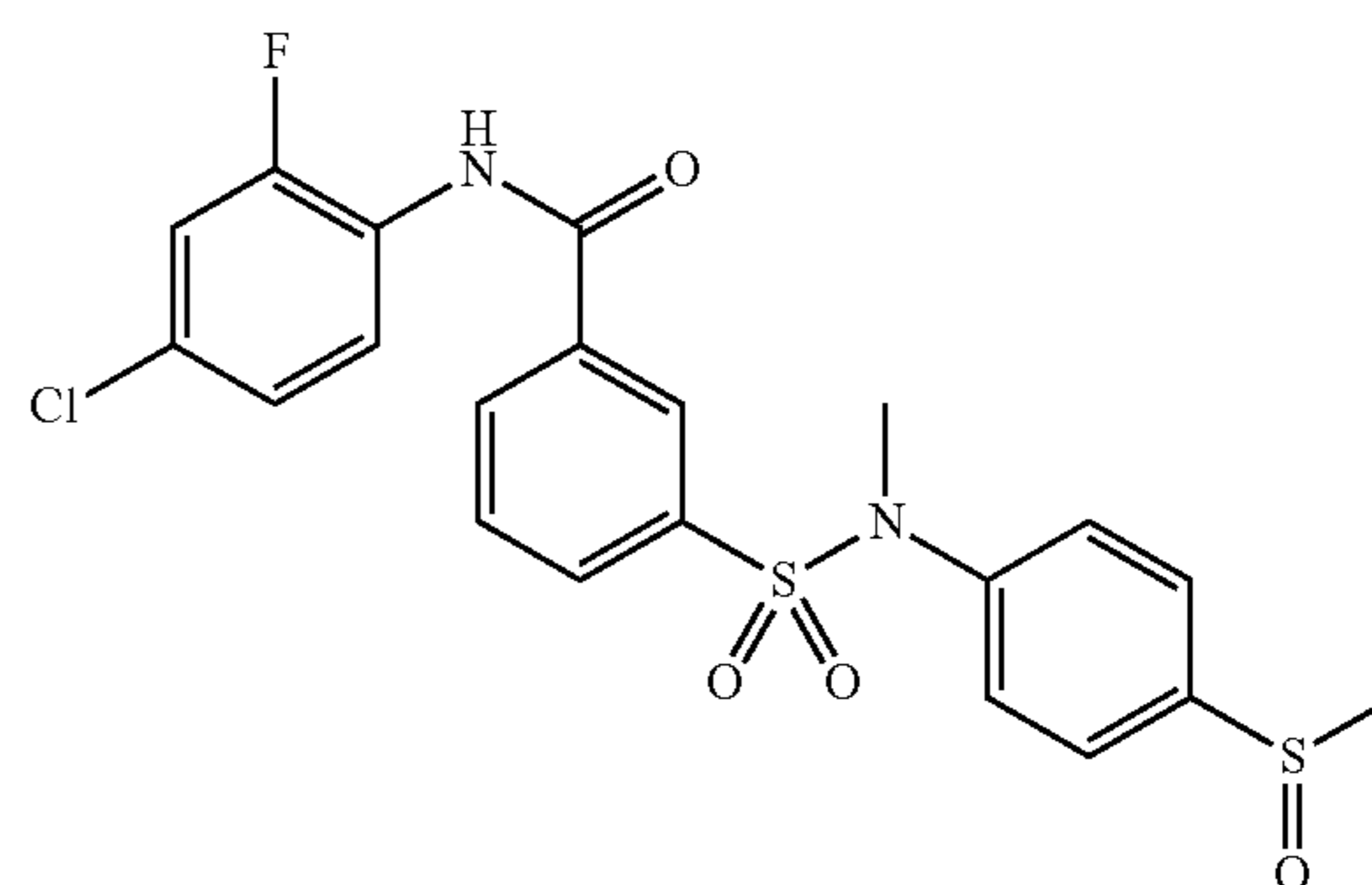
N-(4-chloro-2-fluorophenyl)-3-(N-methyl-N-(4-(methylsulfinyl)phenyl)sulfamoyl)benzamide (203Ad)
