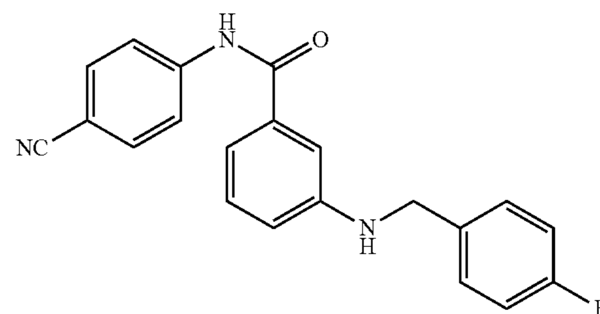
N-(4-cyanophenyl)-3-((4-fluorobenzyl)amino)benzamide (221a)
