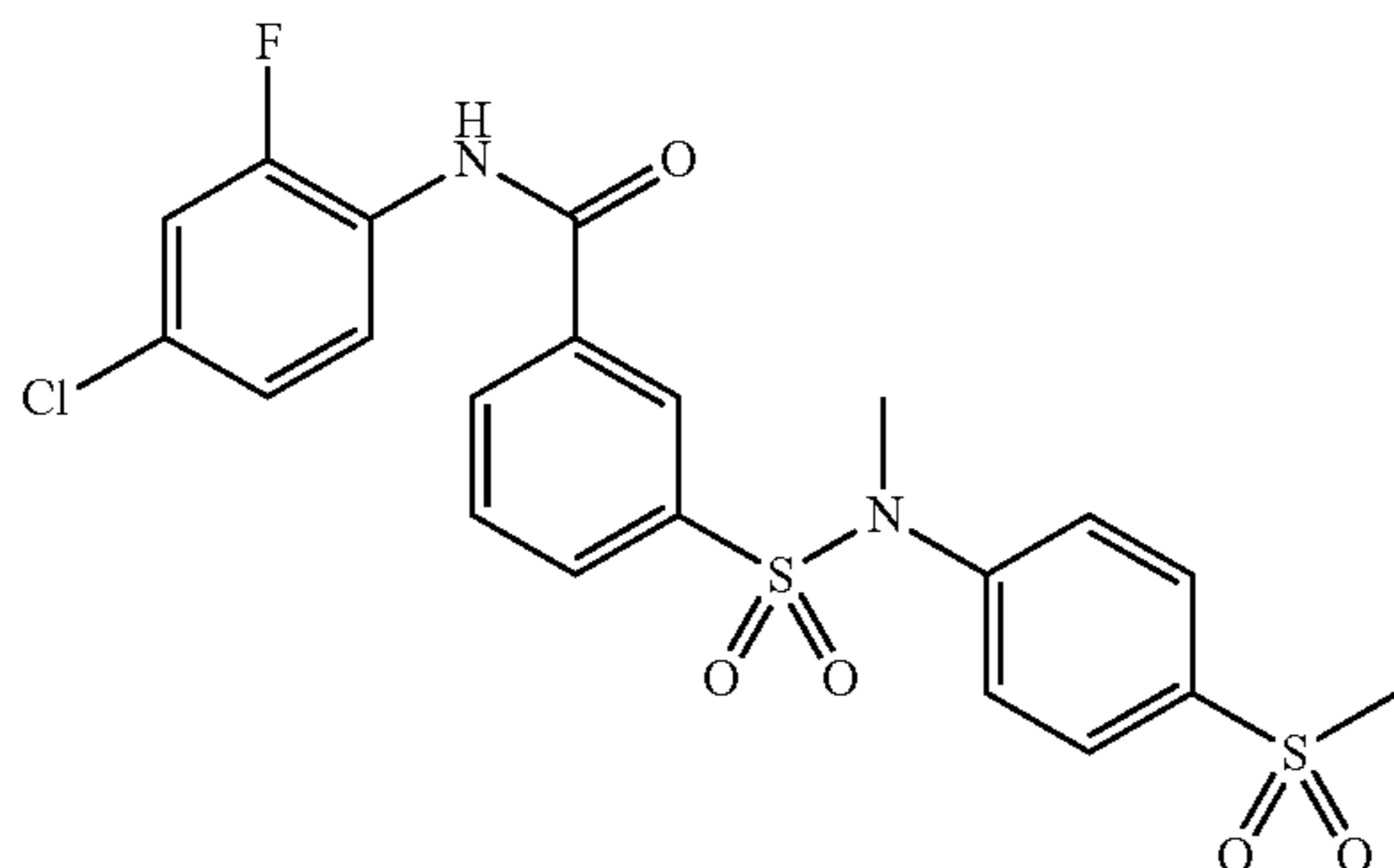
N-(4-chloro-2-fluorophenyl)-3-(N-methyl-N-(4-(methylsulfonyl)phenyl)sulfamoyl)-benzamide (203Ae)
