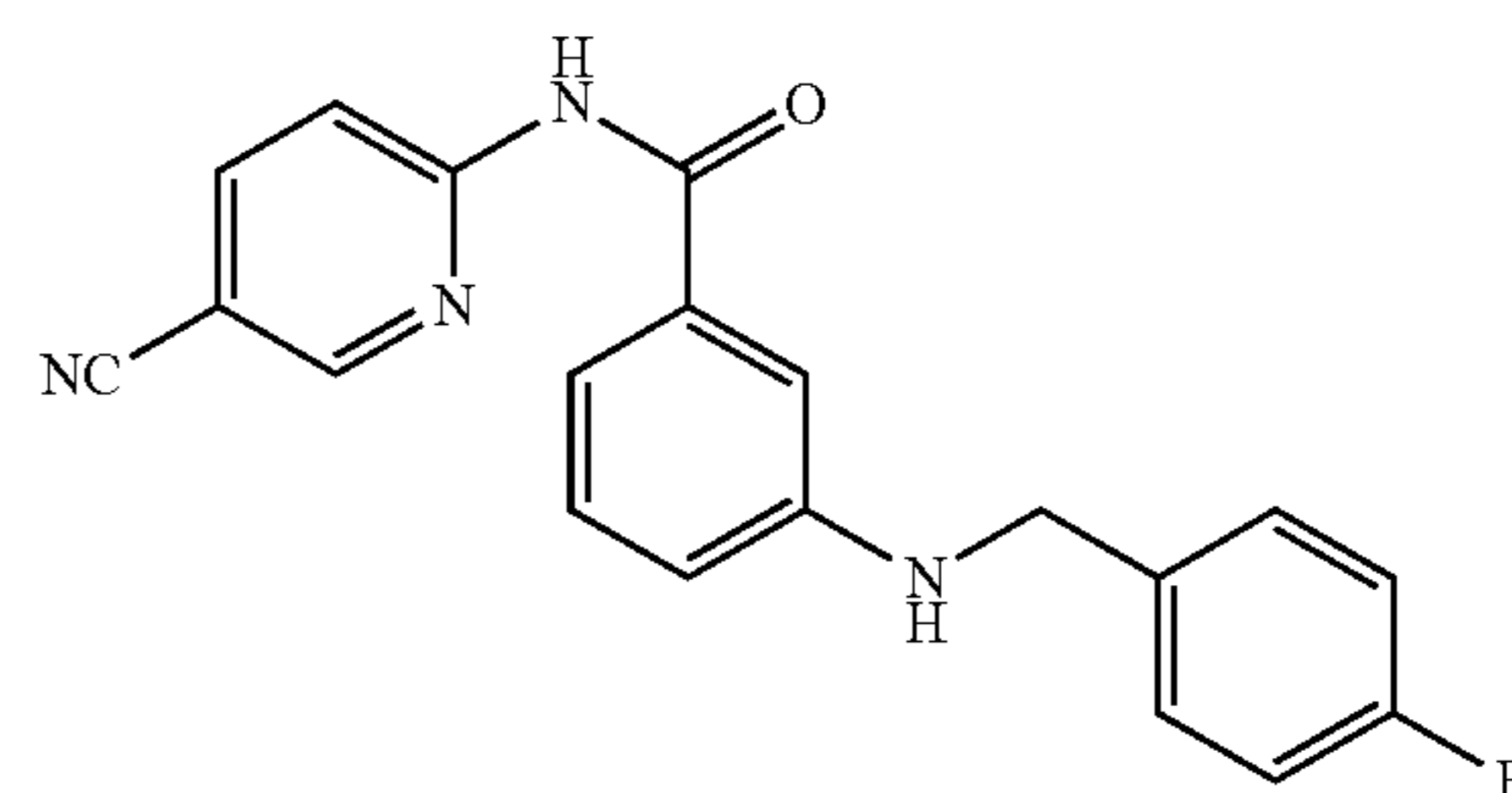
N-(5-cyanopyridin-2-yl)-3-((4-fluorobenzyl)amino)benzamide (221b)
