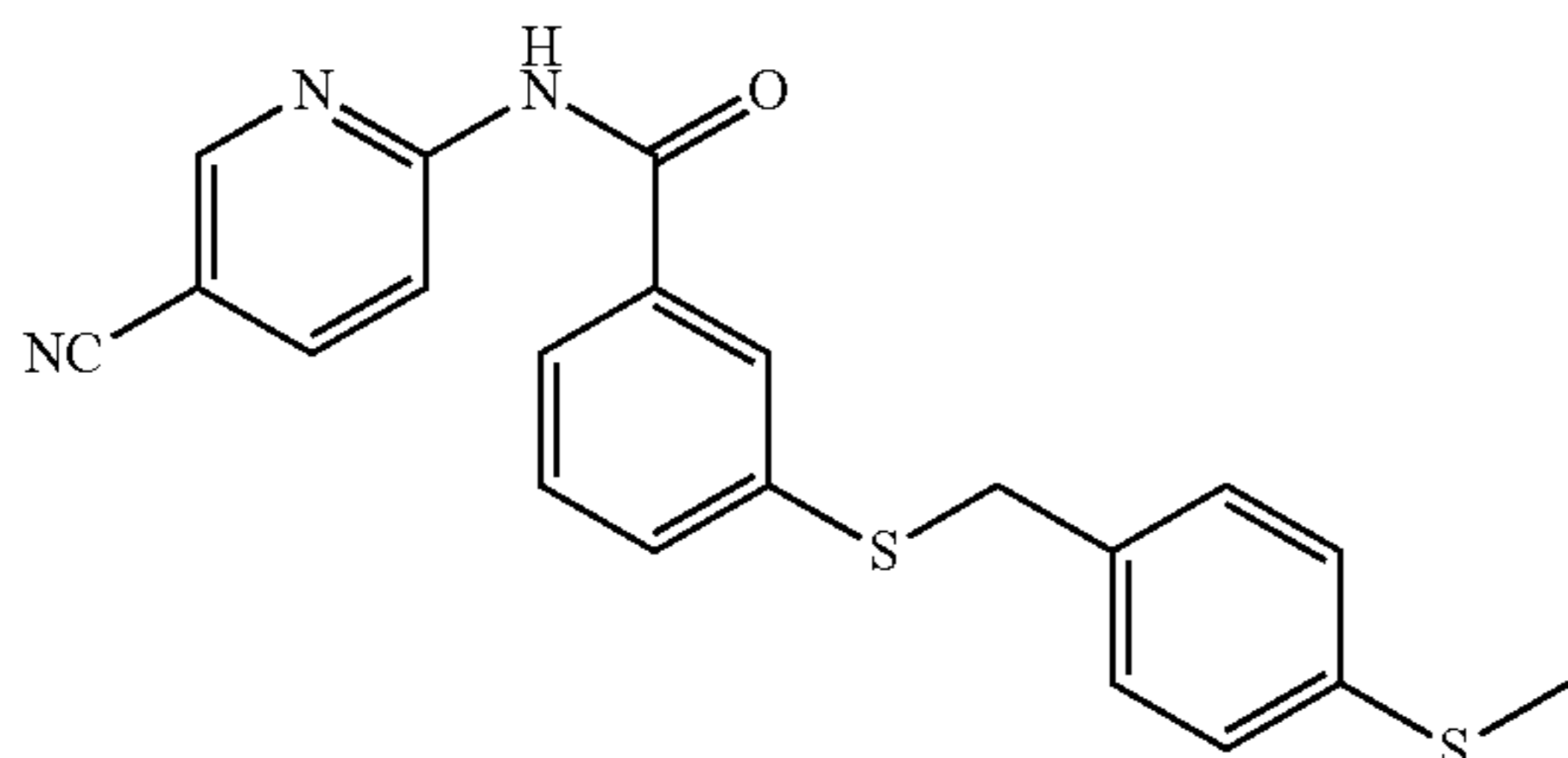
N-(5-cyanopyridin-2-yl)-3-((4-(methylthio)benzyl)thio)benzamide (211a)
