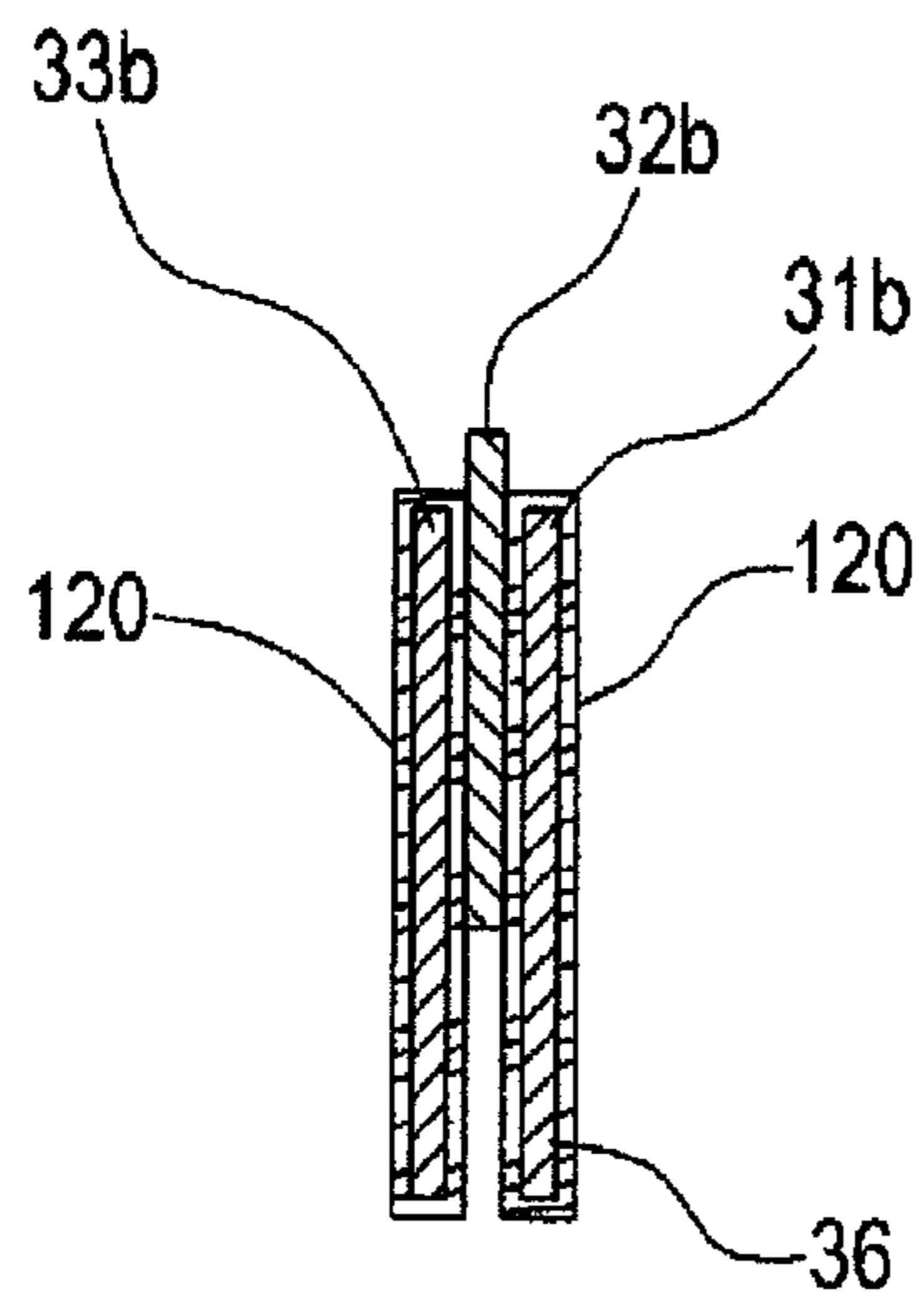
VIEW A-A
