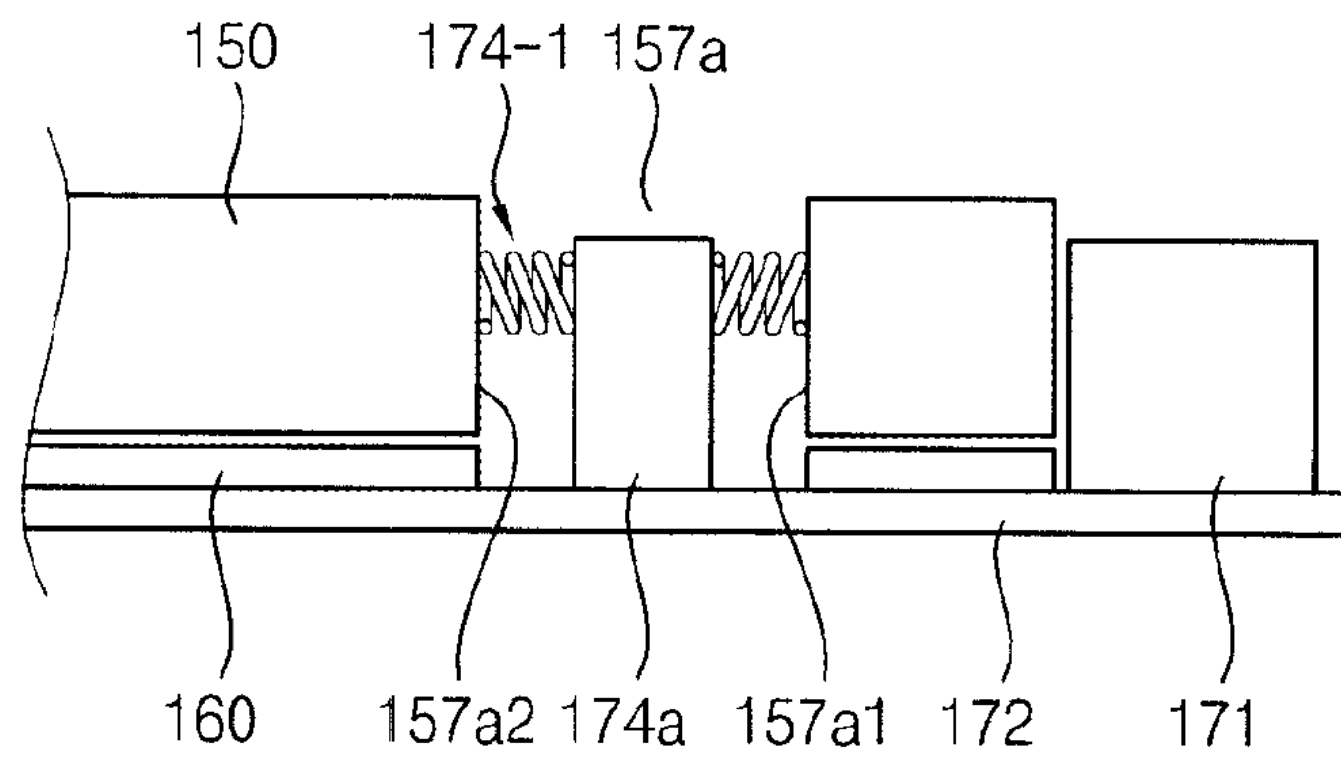
FIG. 7B
