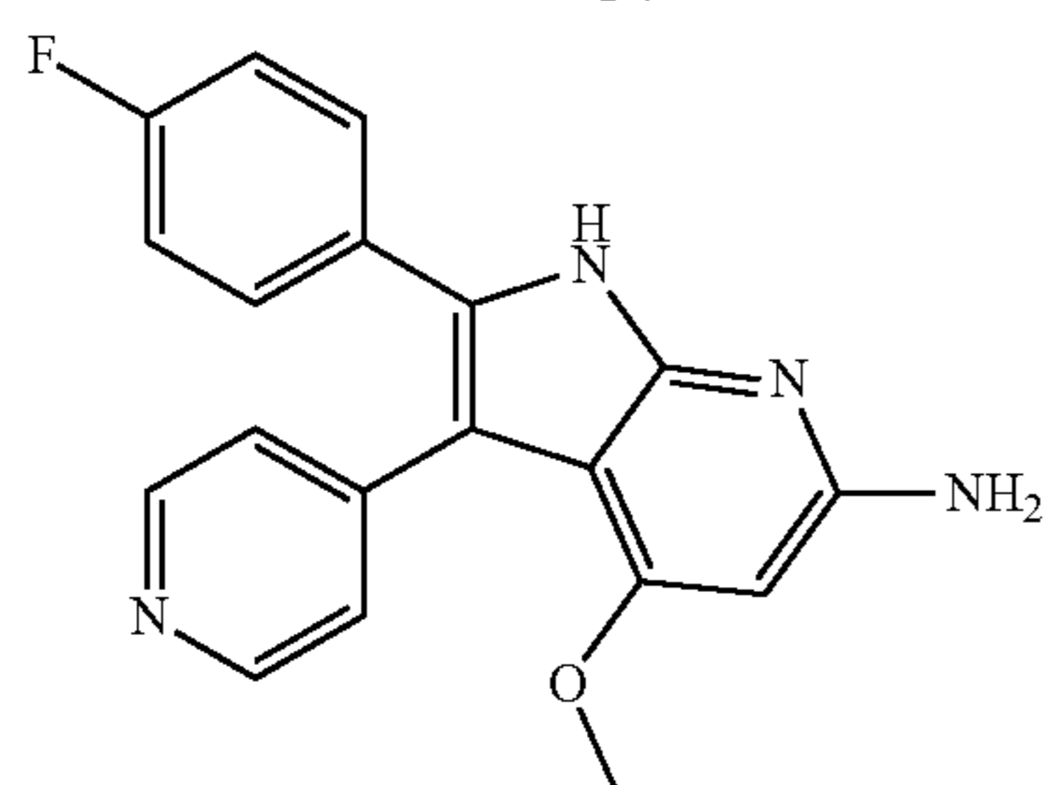
P5 RWJ 68354
