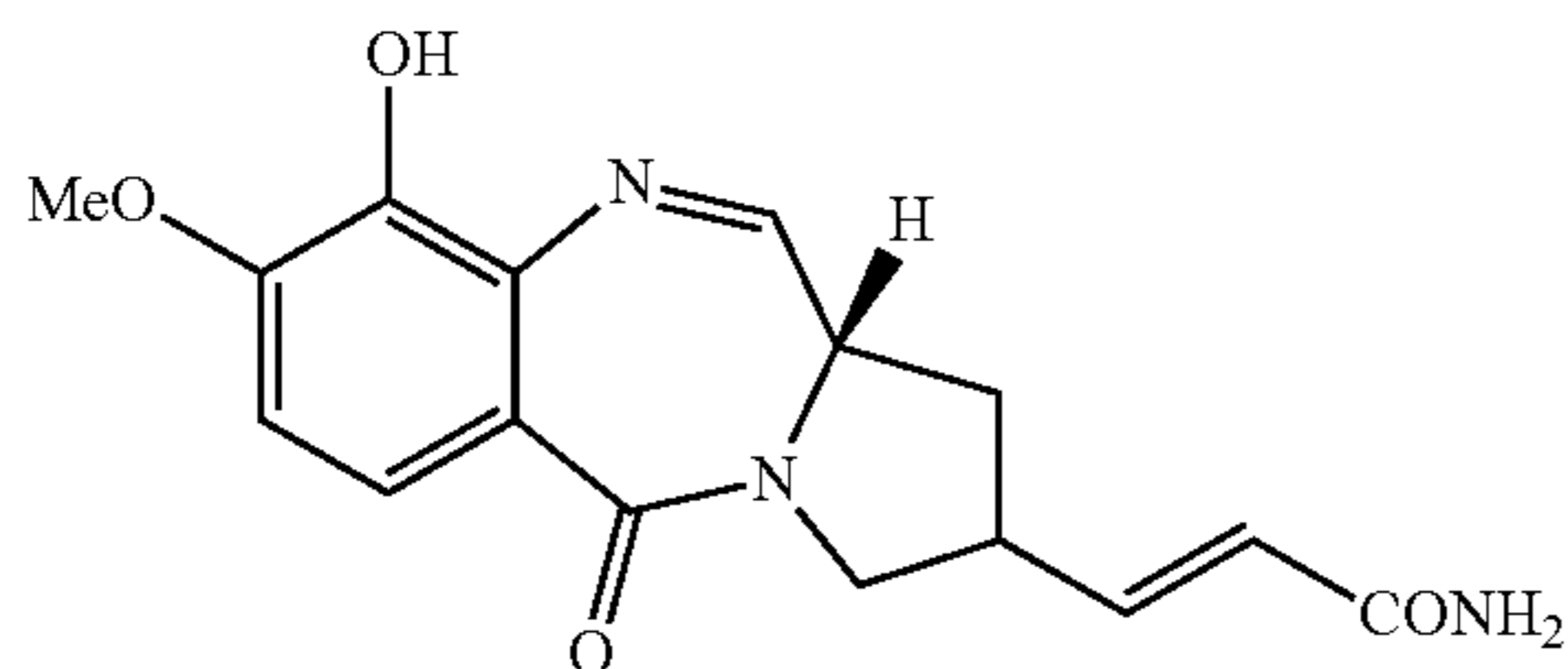
Tomaymycin
