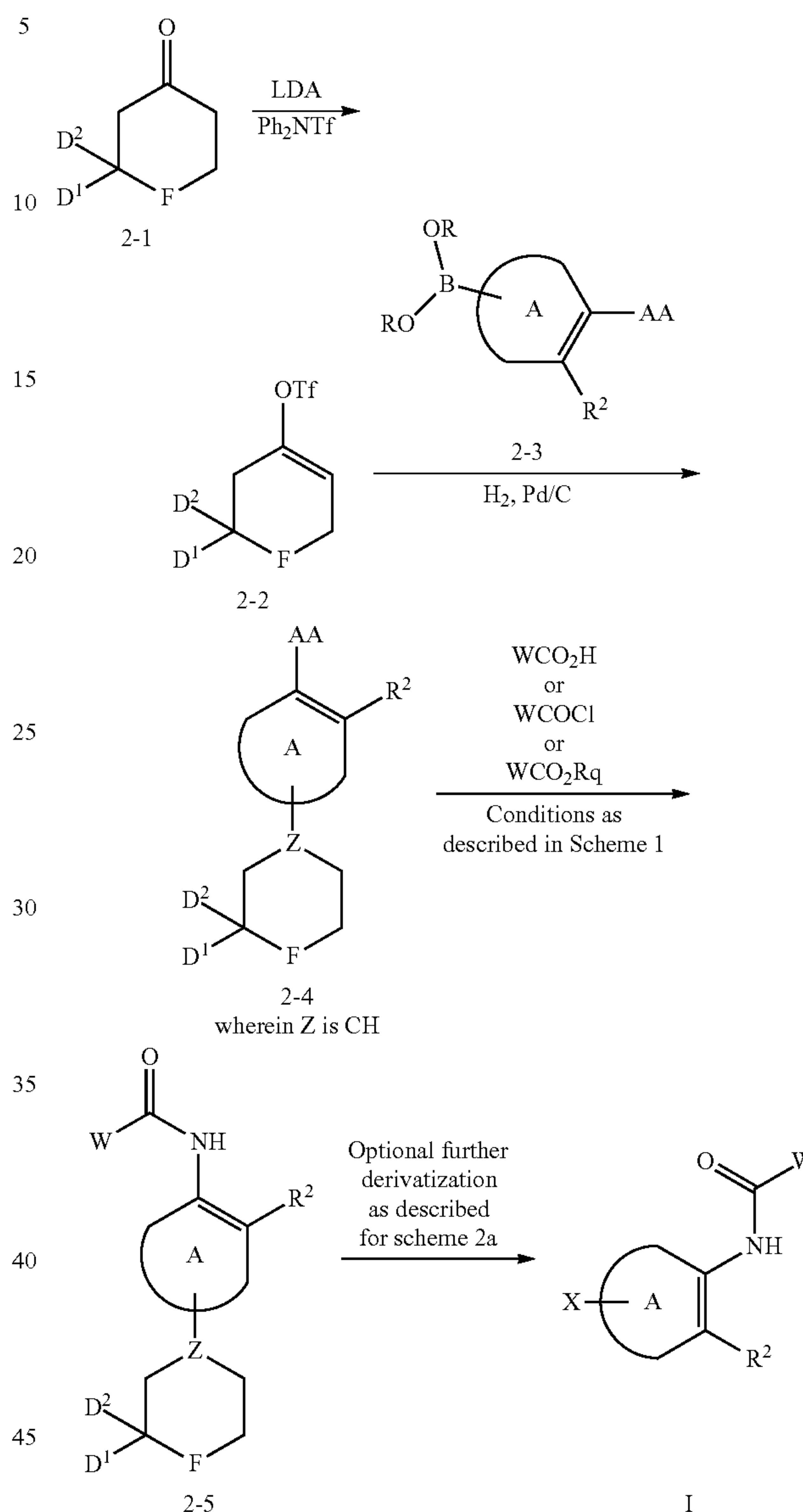
Scheme 2a
