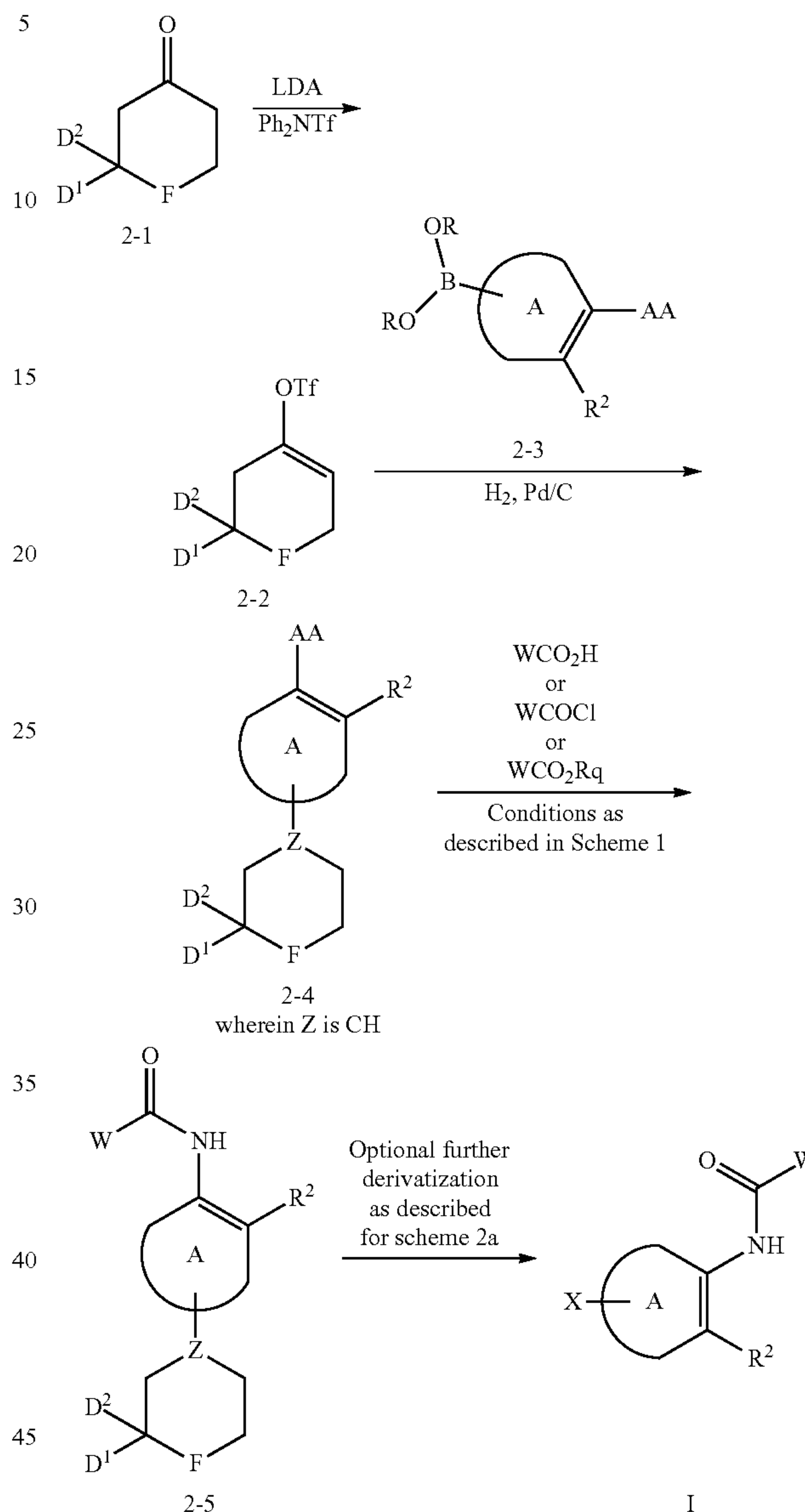
Scheme 2a
