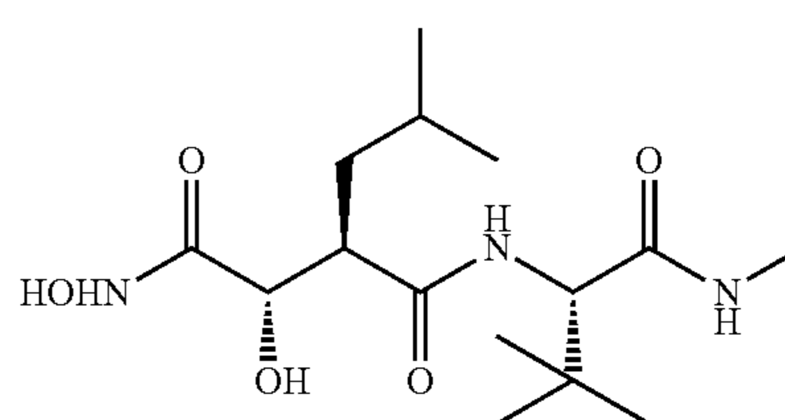
Marimastat
