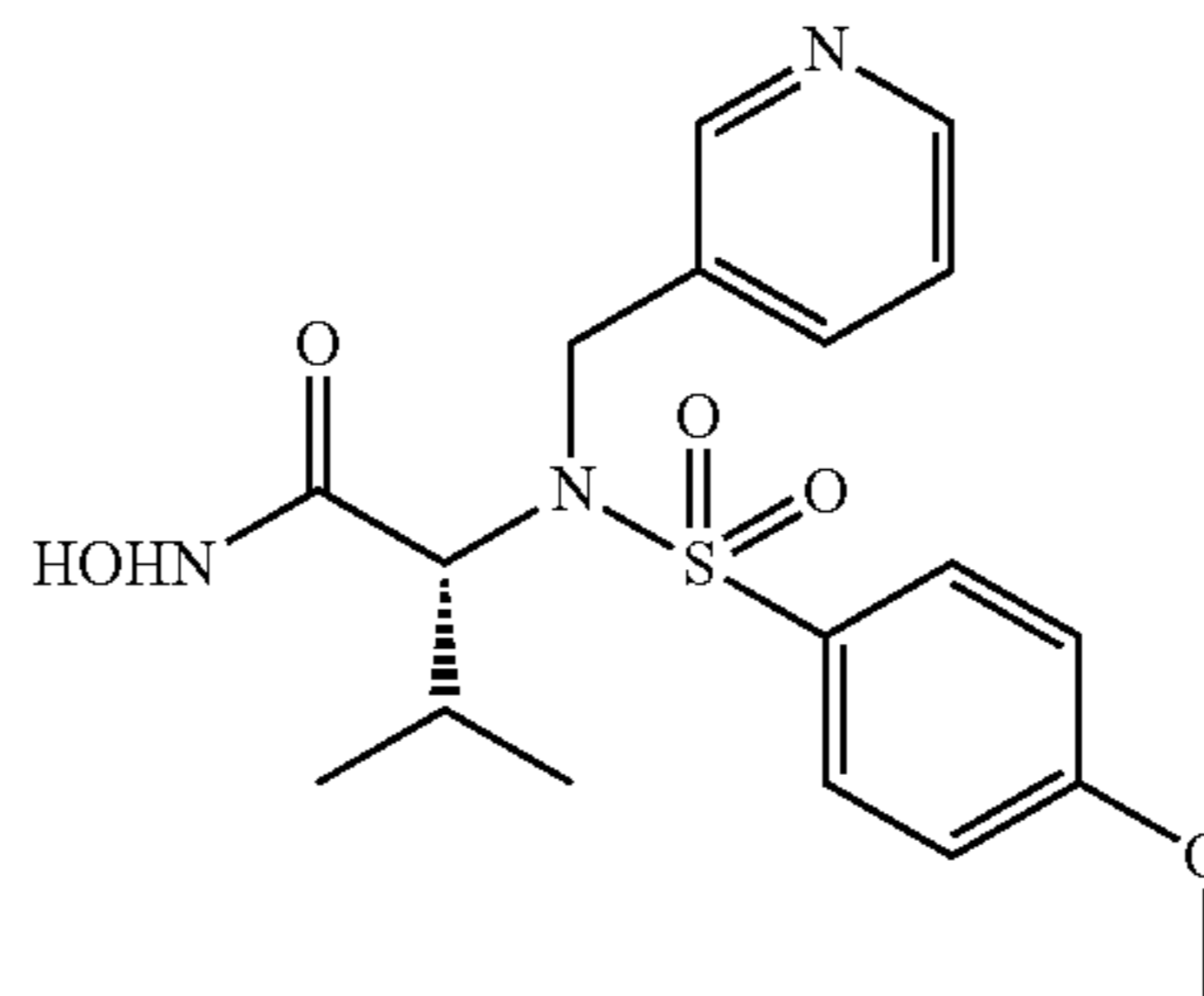
CGS-27023
