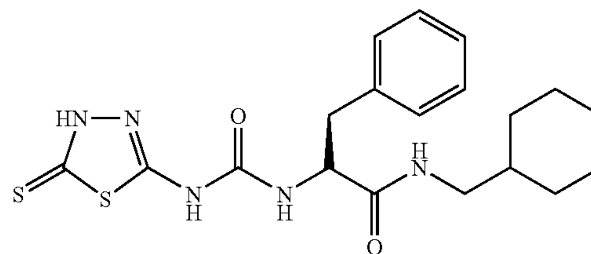
-[[[4,5-Dihydro-5-thioxo-1,3,4-thiadiazol-2-yl]amino]carbonyl]amino]-N-(cyclohexylmethyl)-(S)-benzenepropanamide
