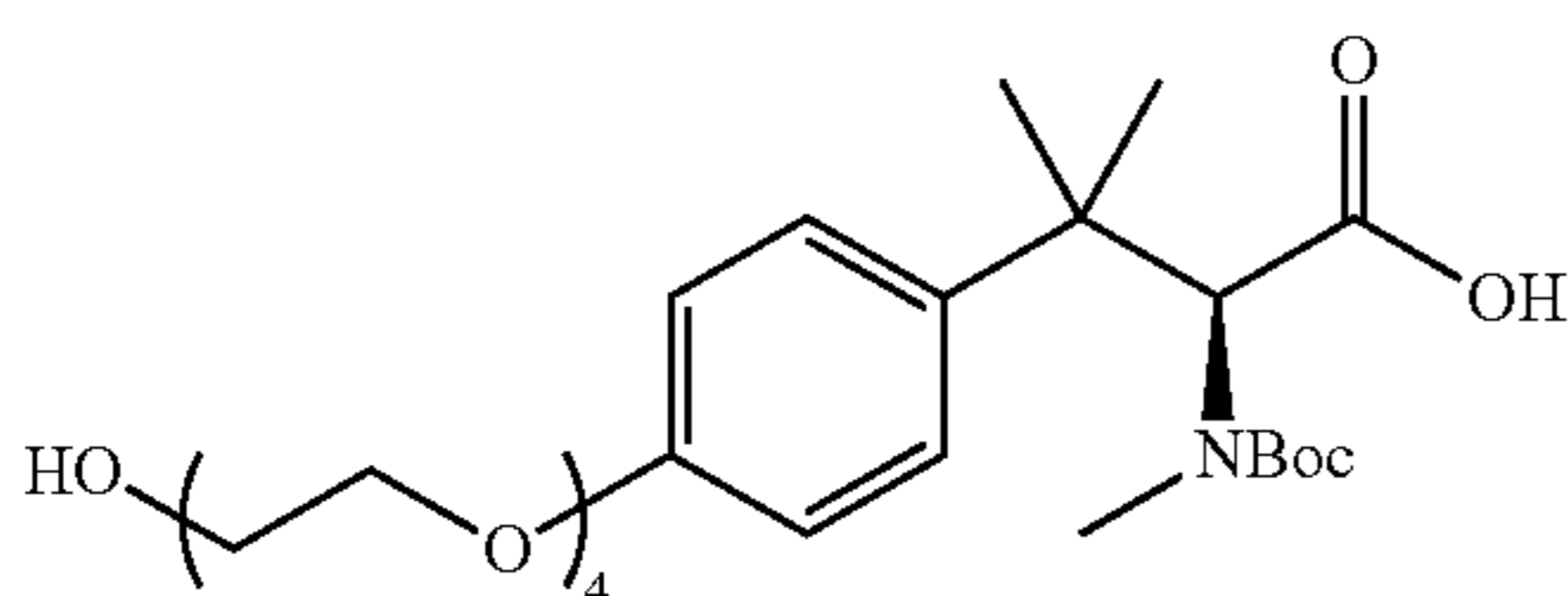
(S)-2-(((tert-butoxycarbonyl)(methyl)amino)-3-(2-(2-hydroxyethoxy)ethoxy)ethoxy)phenyl)-3-methylbutanoic acid
