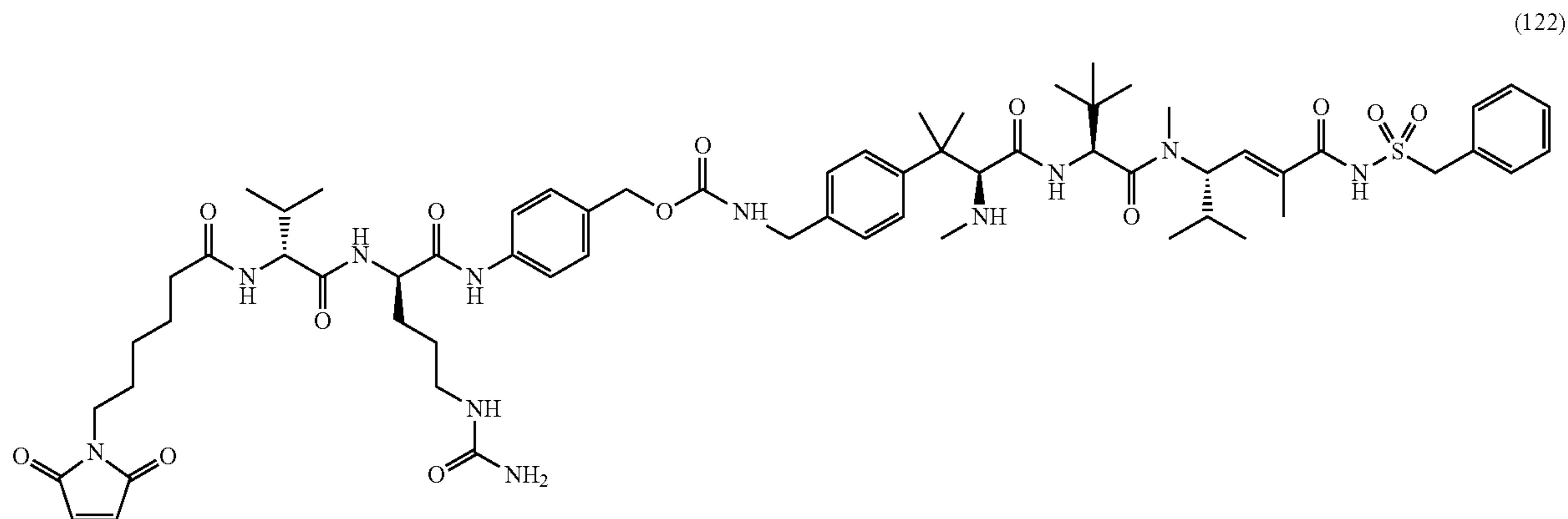
MC-VC-PABC-41
