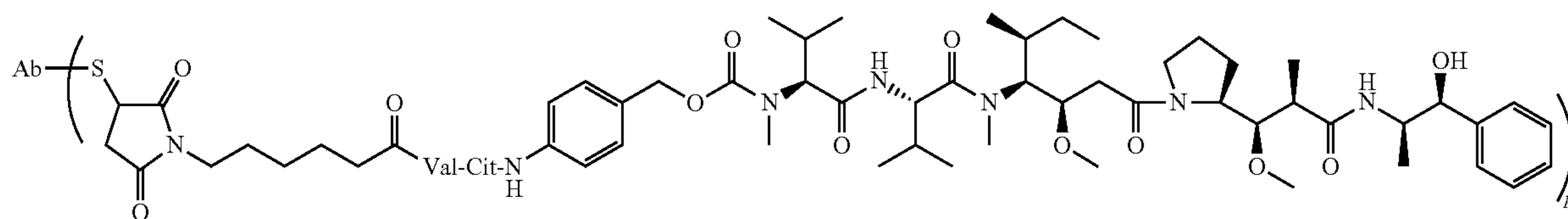
Ab-MC-vc-PAB-MMAE
