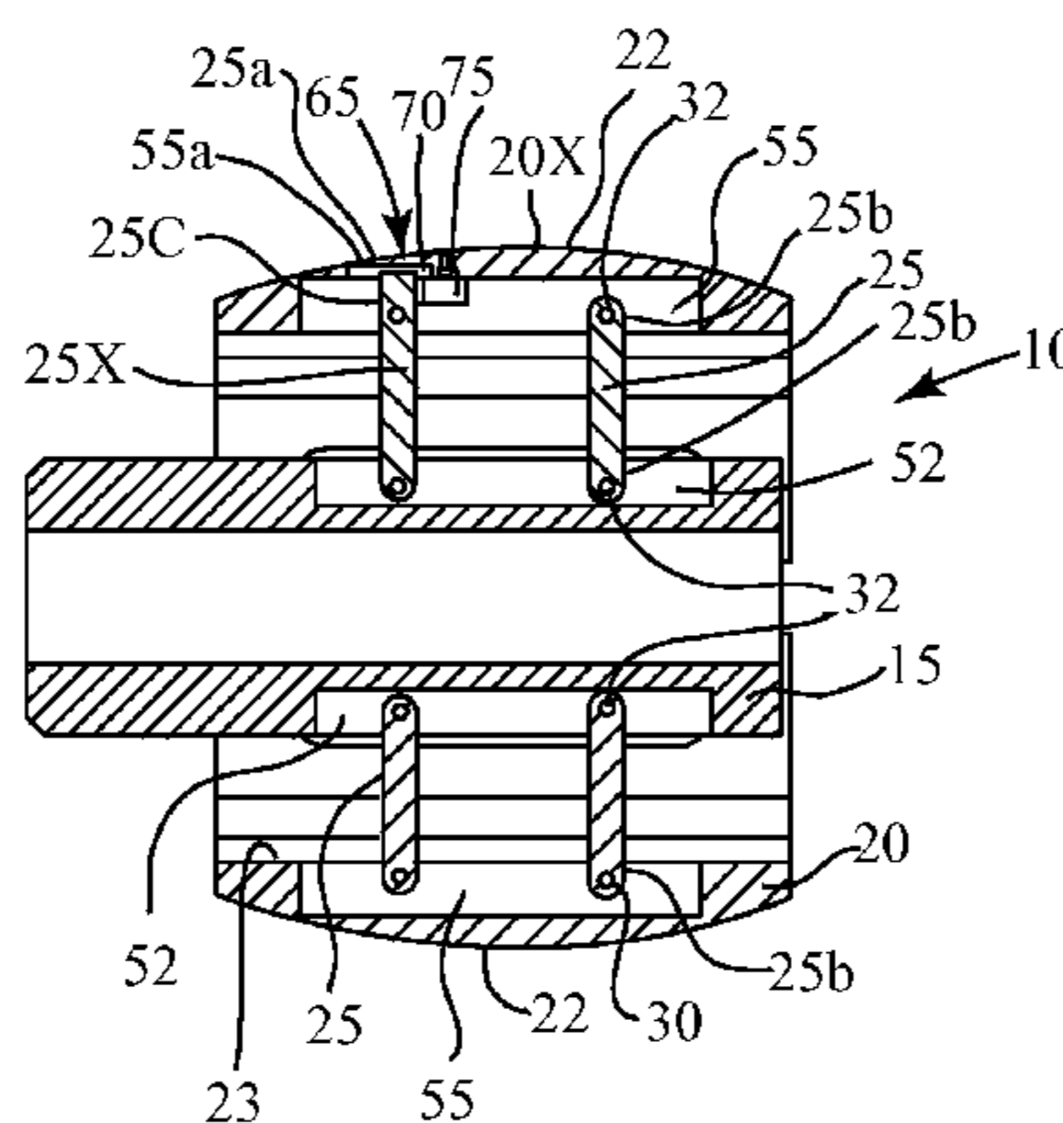
Section A-A
