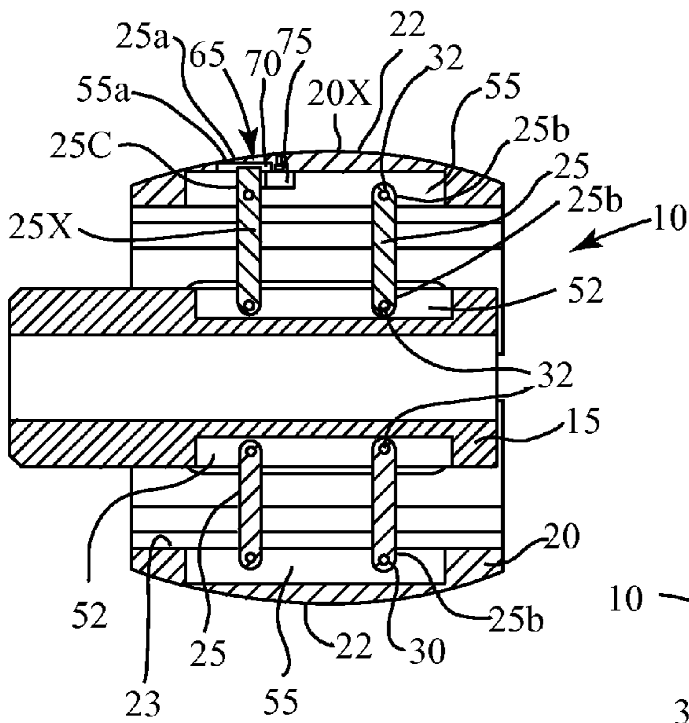
Fig. 3 Section A-A
