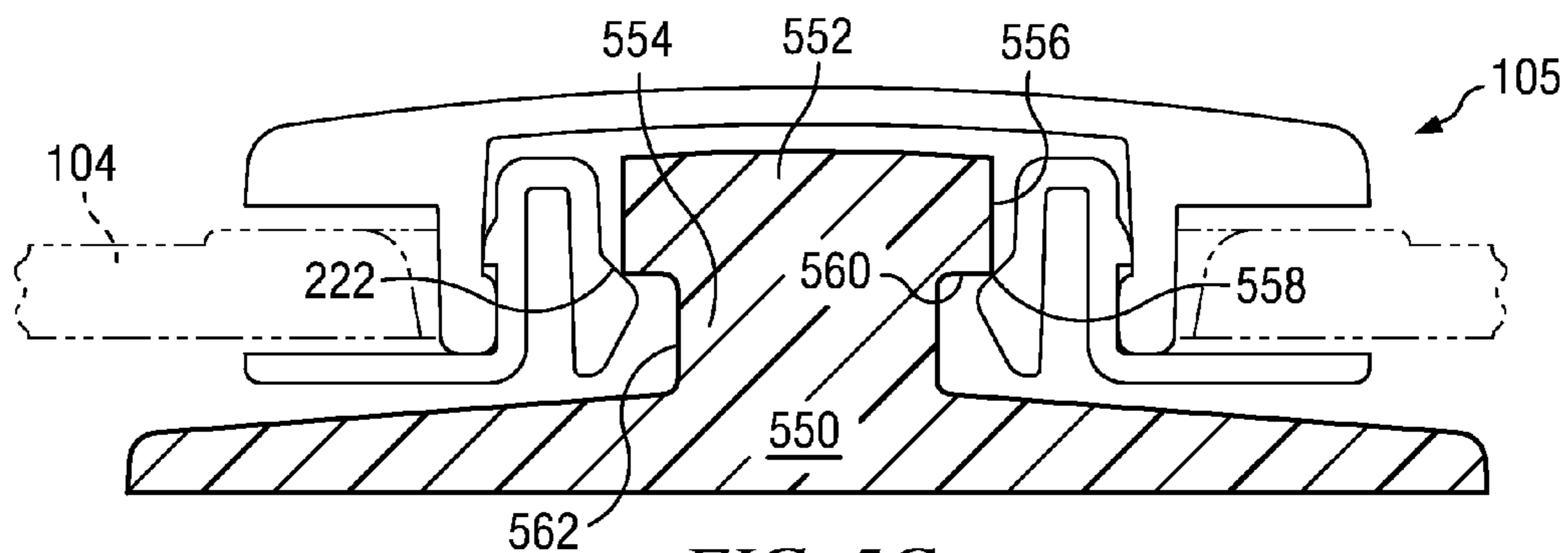
FIG. 5C
