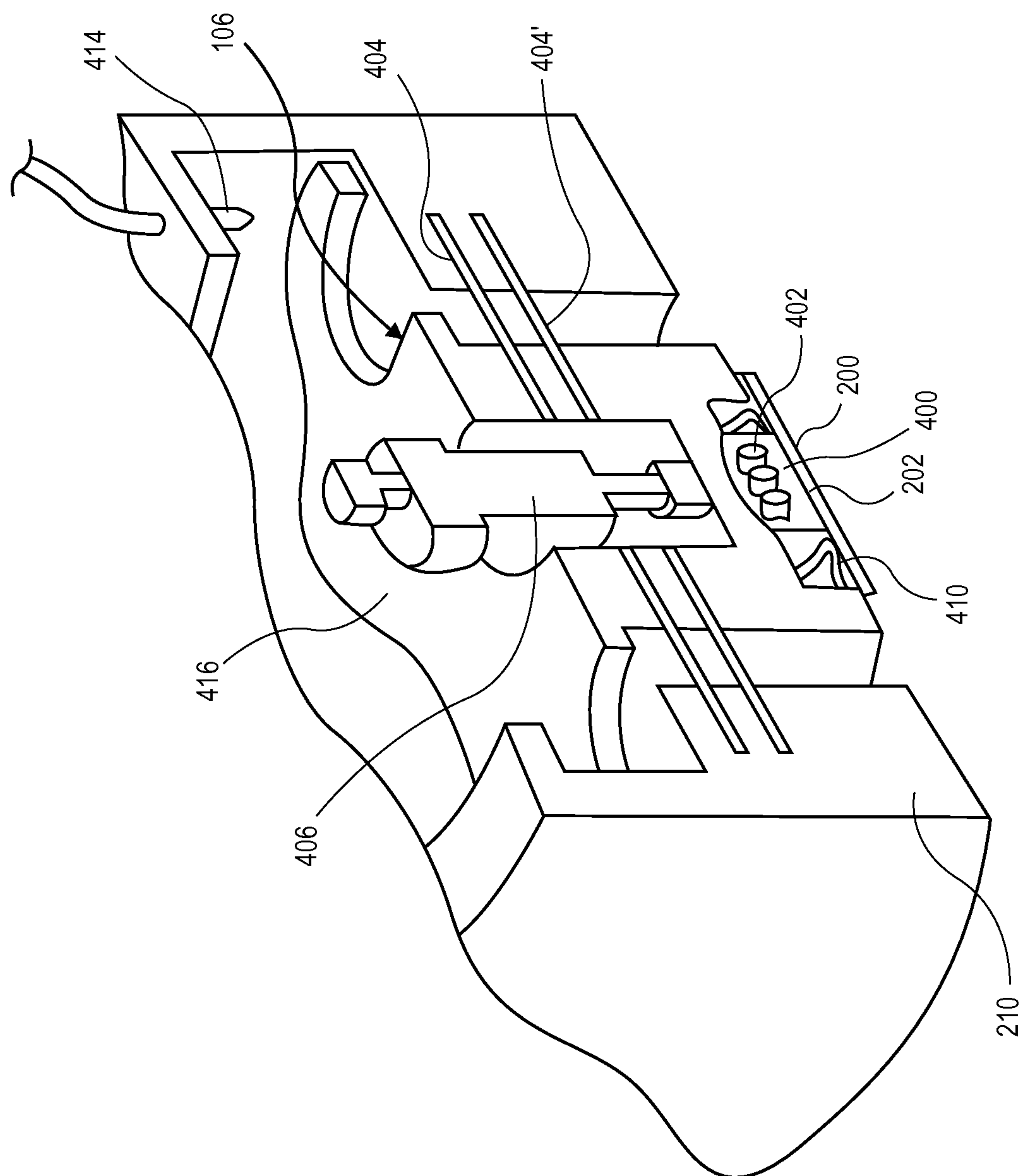
SECTION A-A
