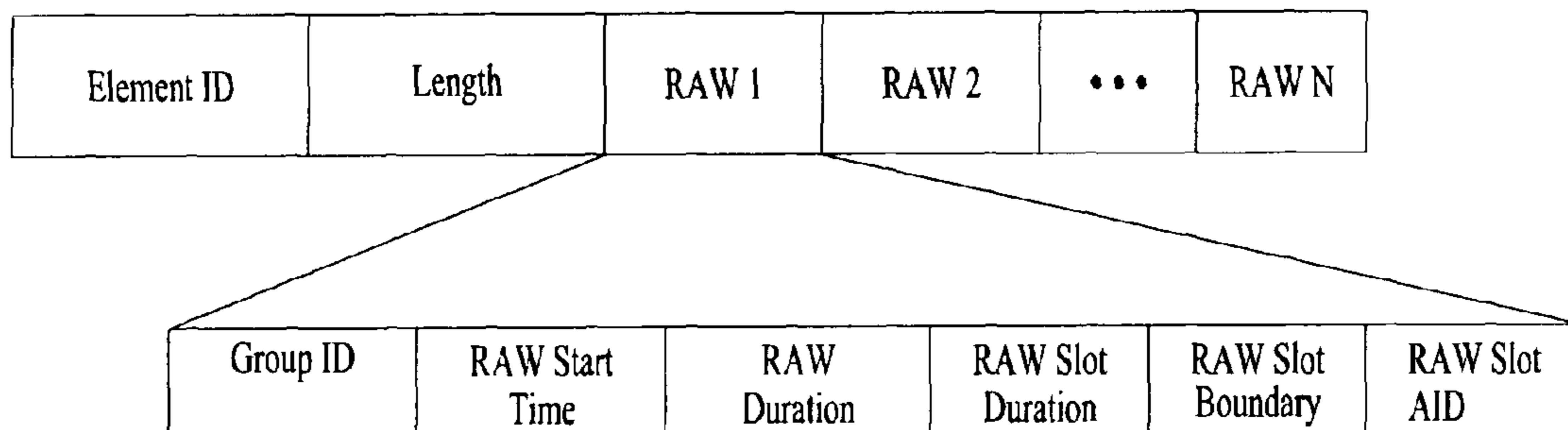
FIG. 16
