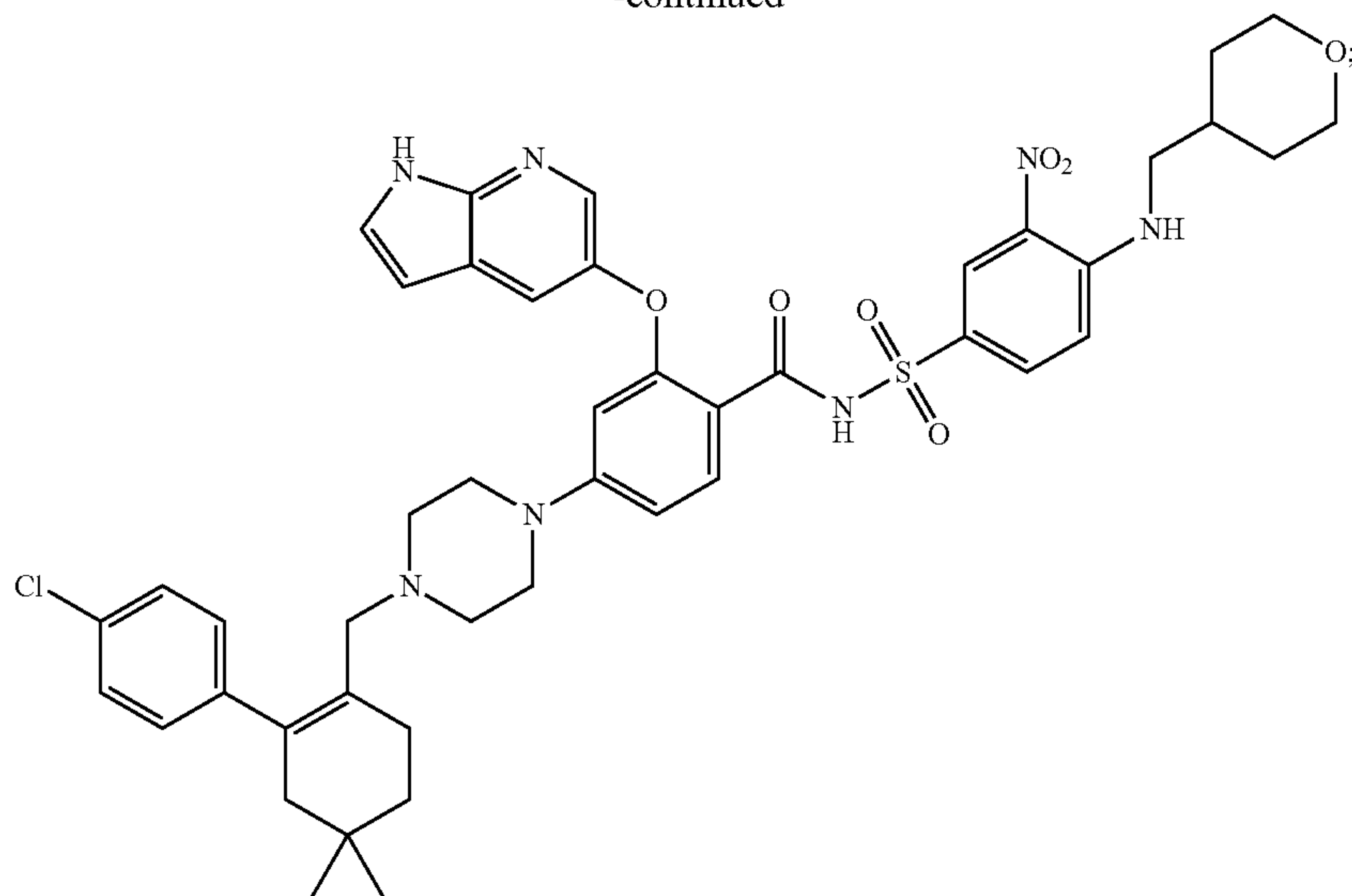
(ABT-199, GDC-0199)
