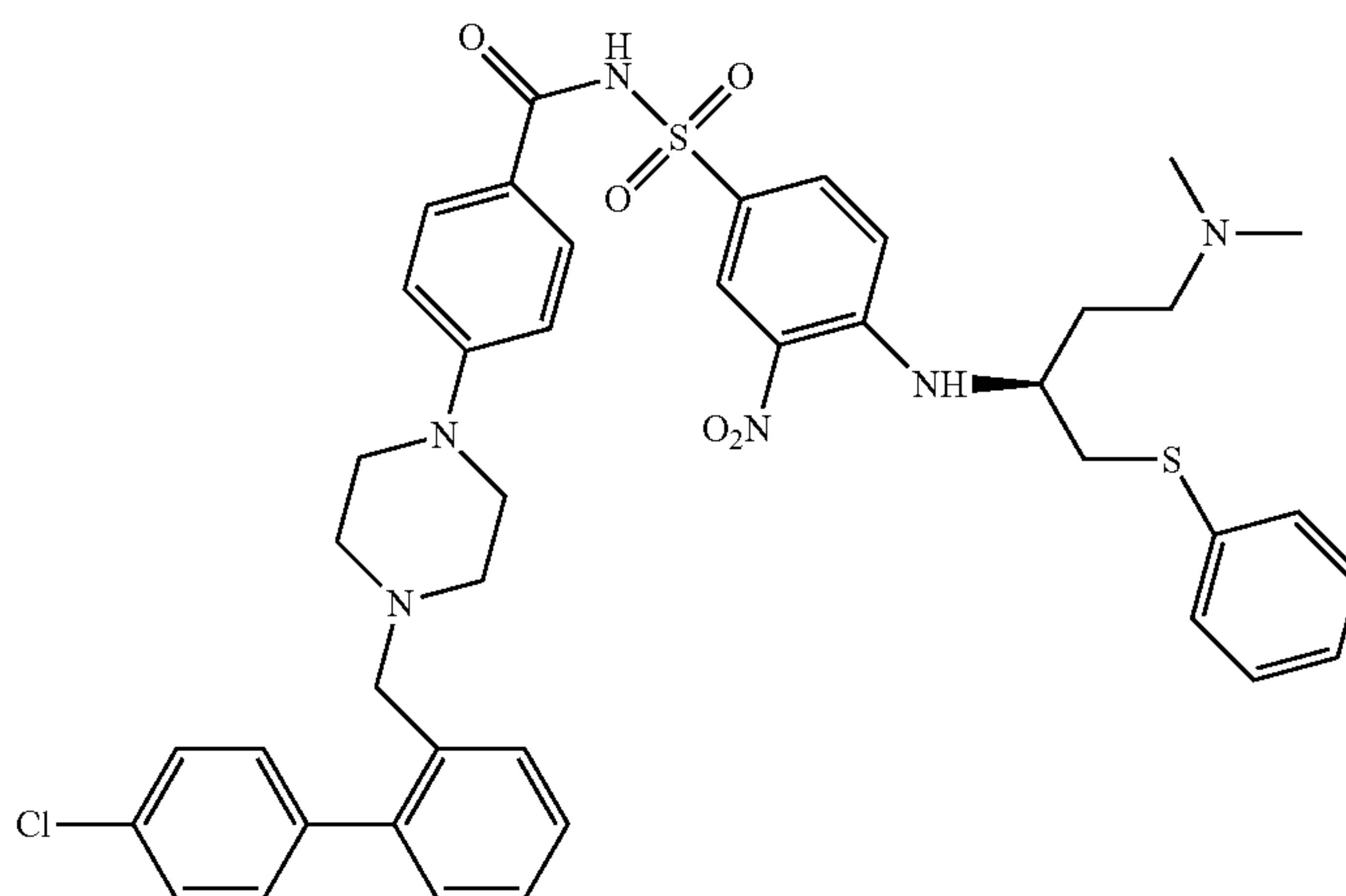
(ABT-737)
