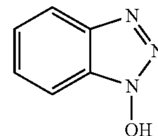
HOBT
