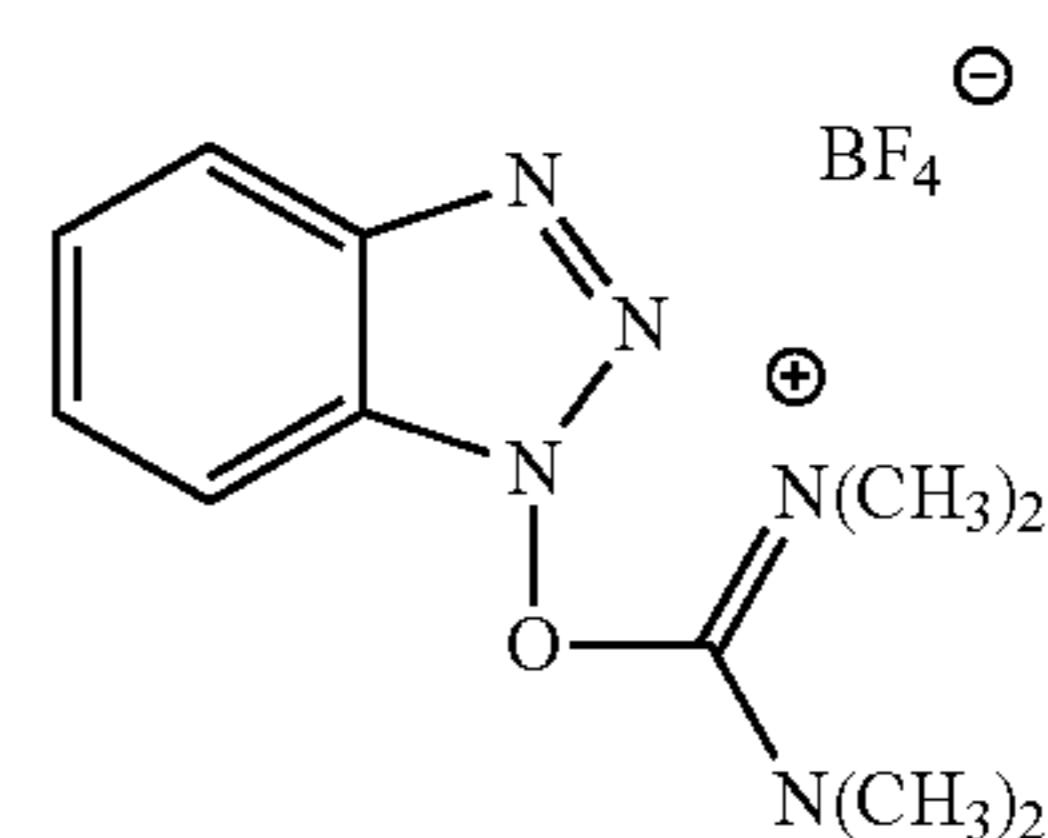
TBTU
