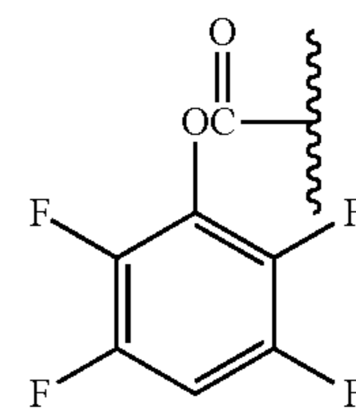
TFP
