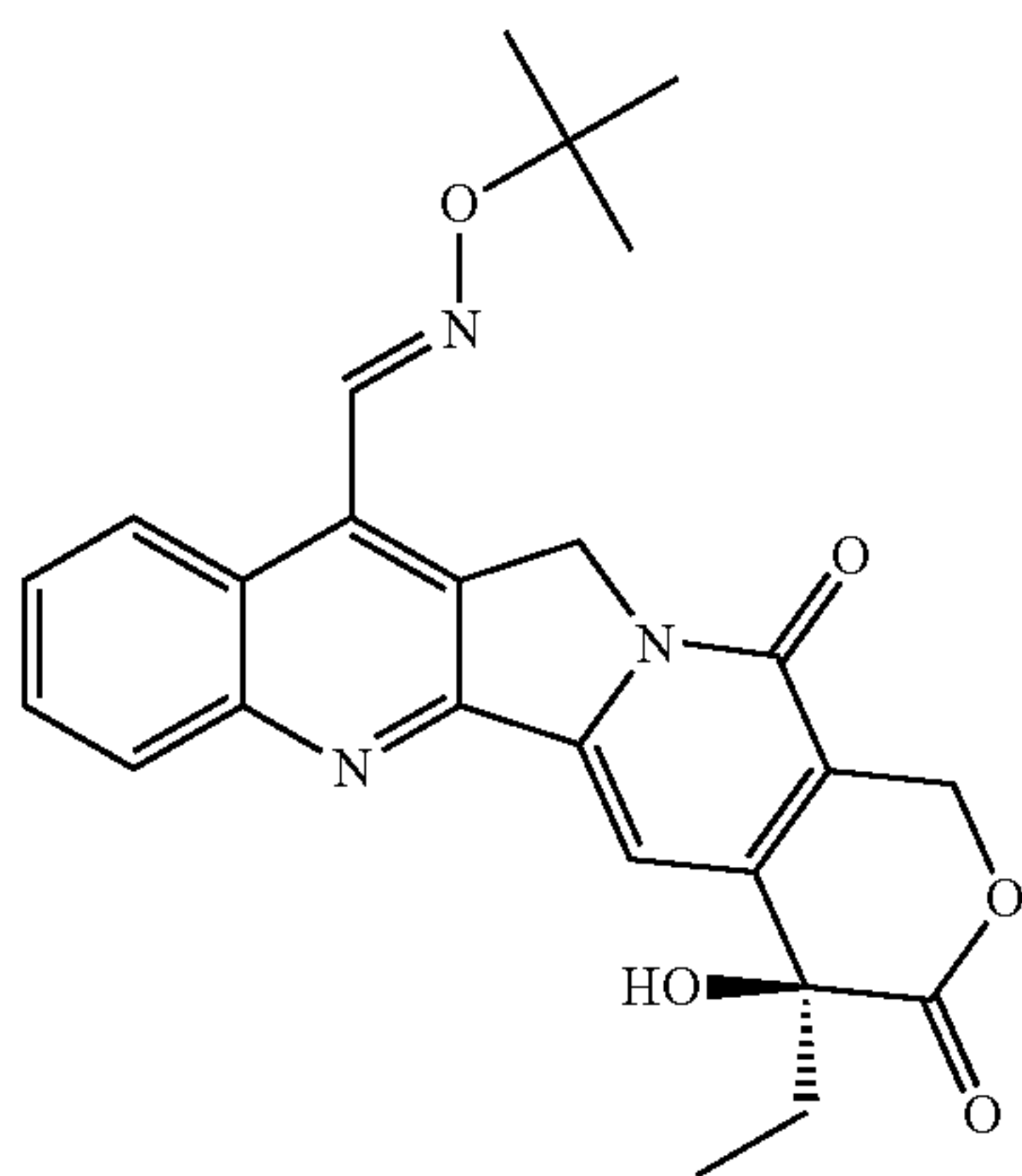
Gimatecan
