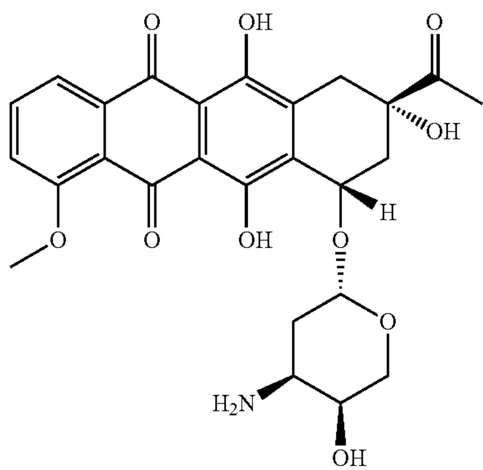
daunorubicin
