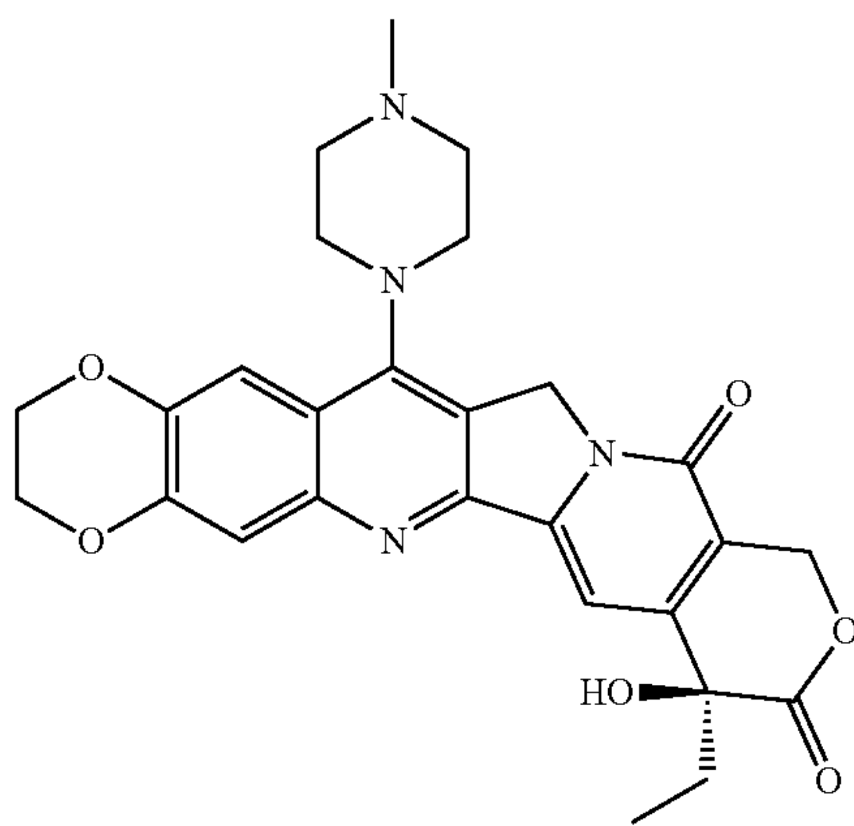
Lurtotecan
