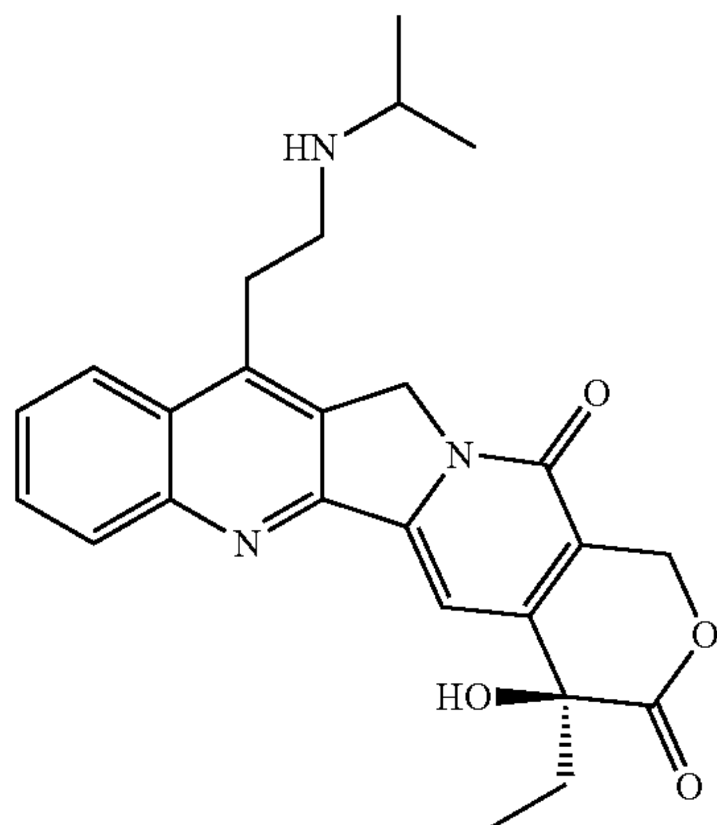
CKD 602
