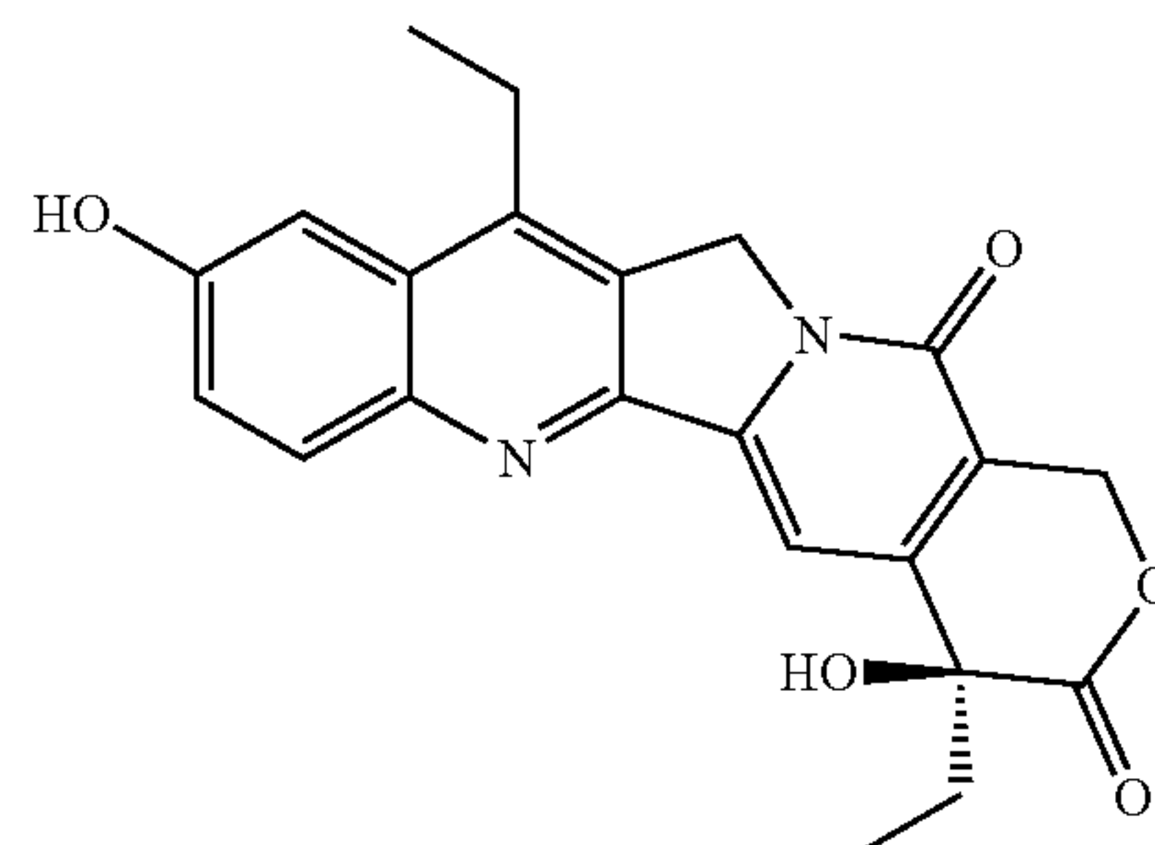
SN-38
