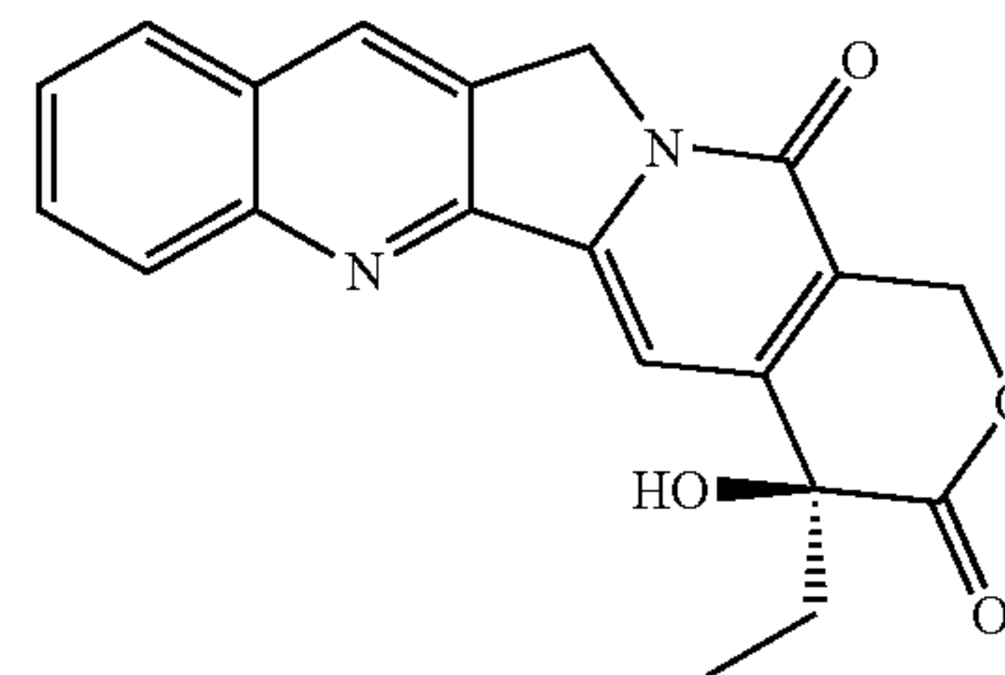
Camptothecin
