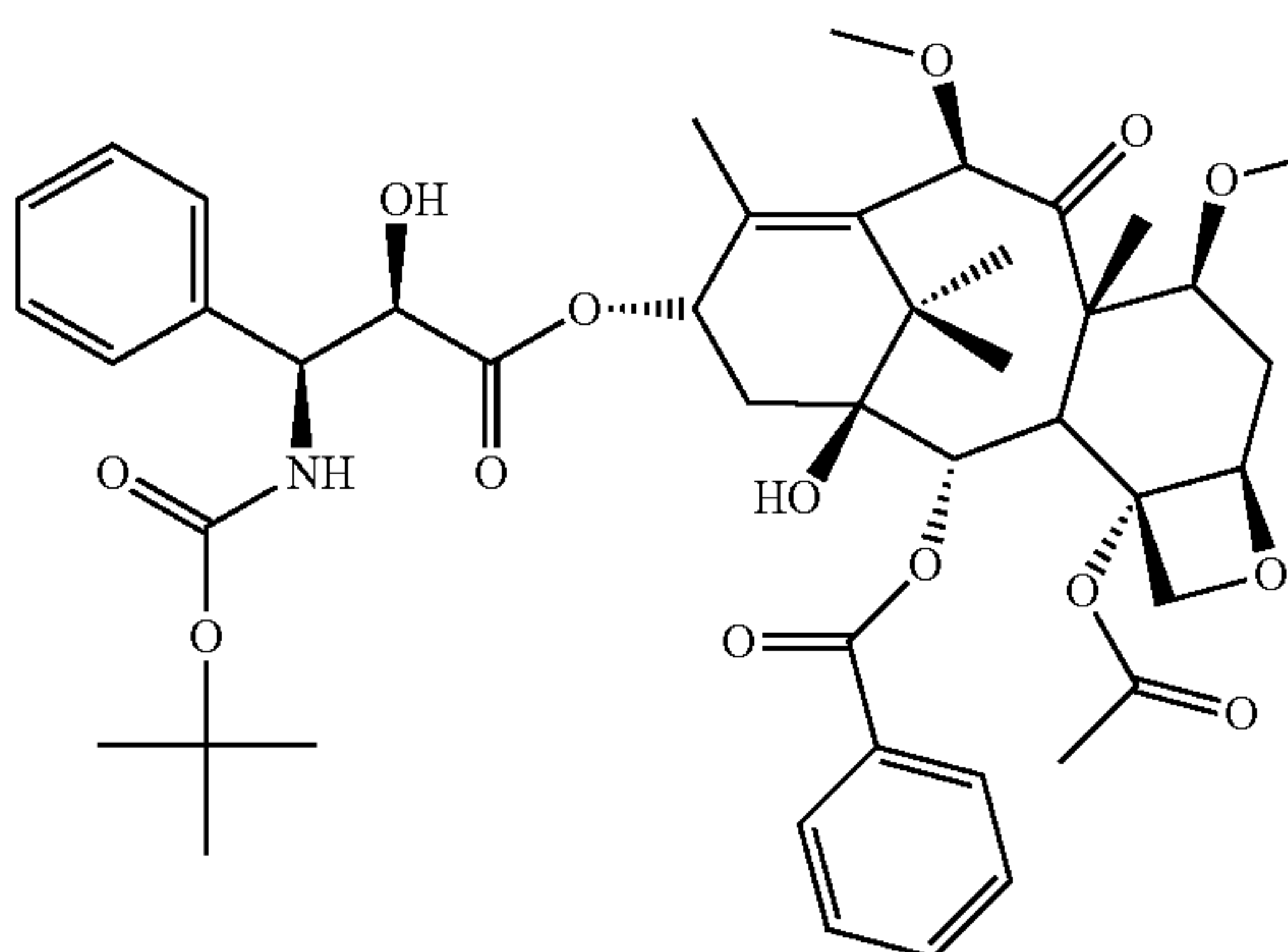
Cabazitaxel
