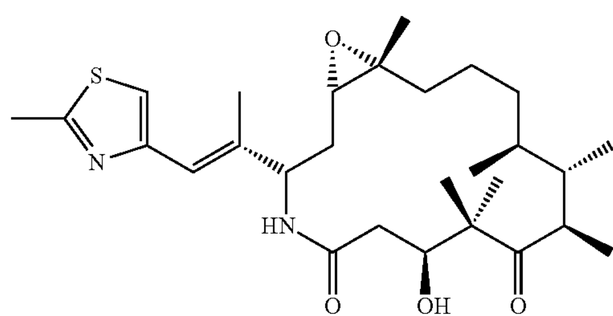
Ixepilone
