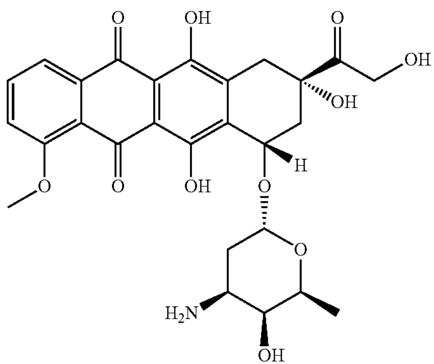
doxorubicin
