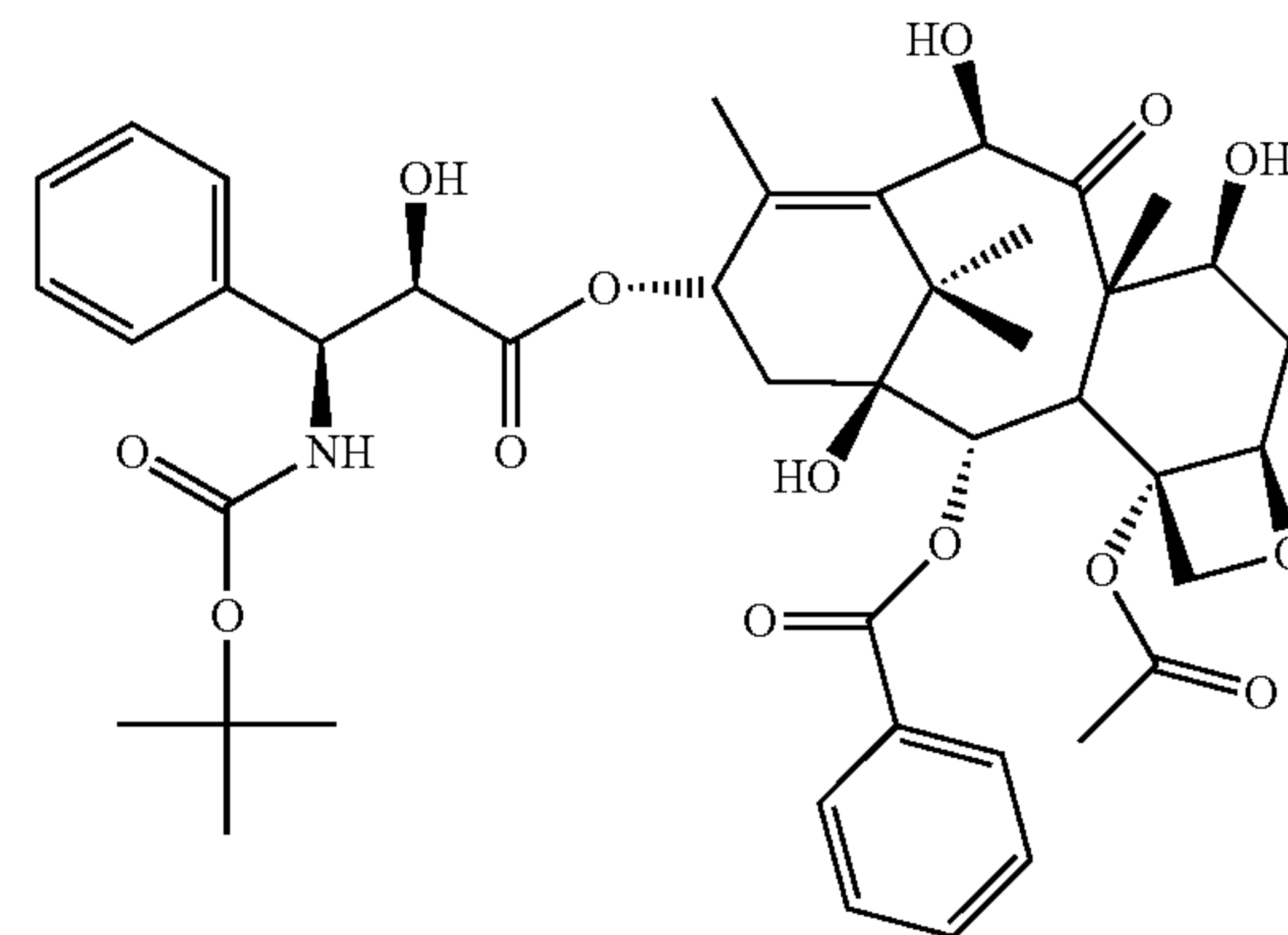
Doxetaxel
