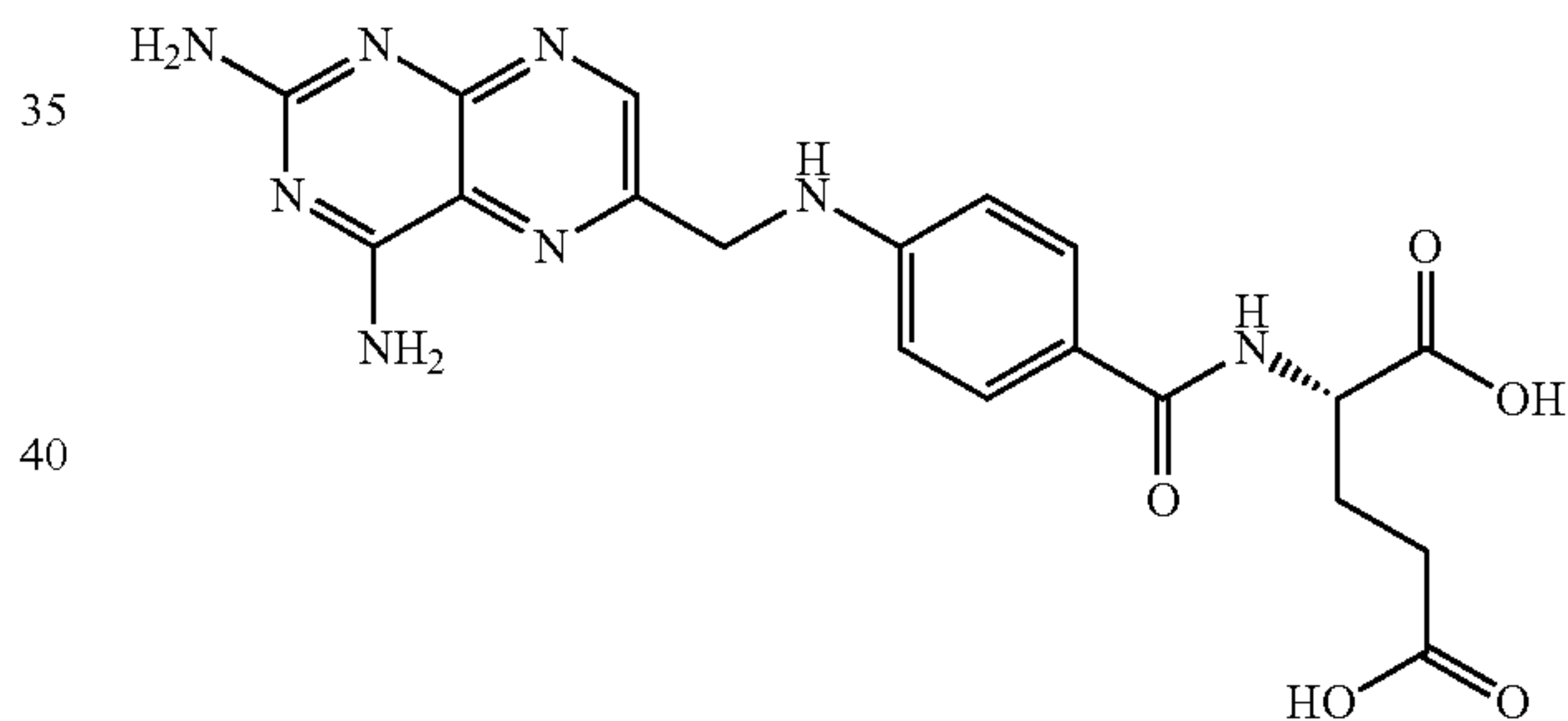
Aminopterin
