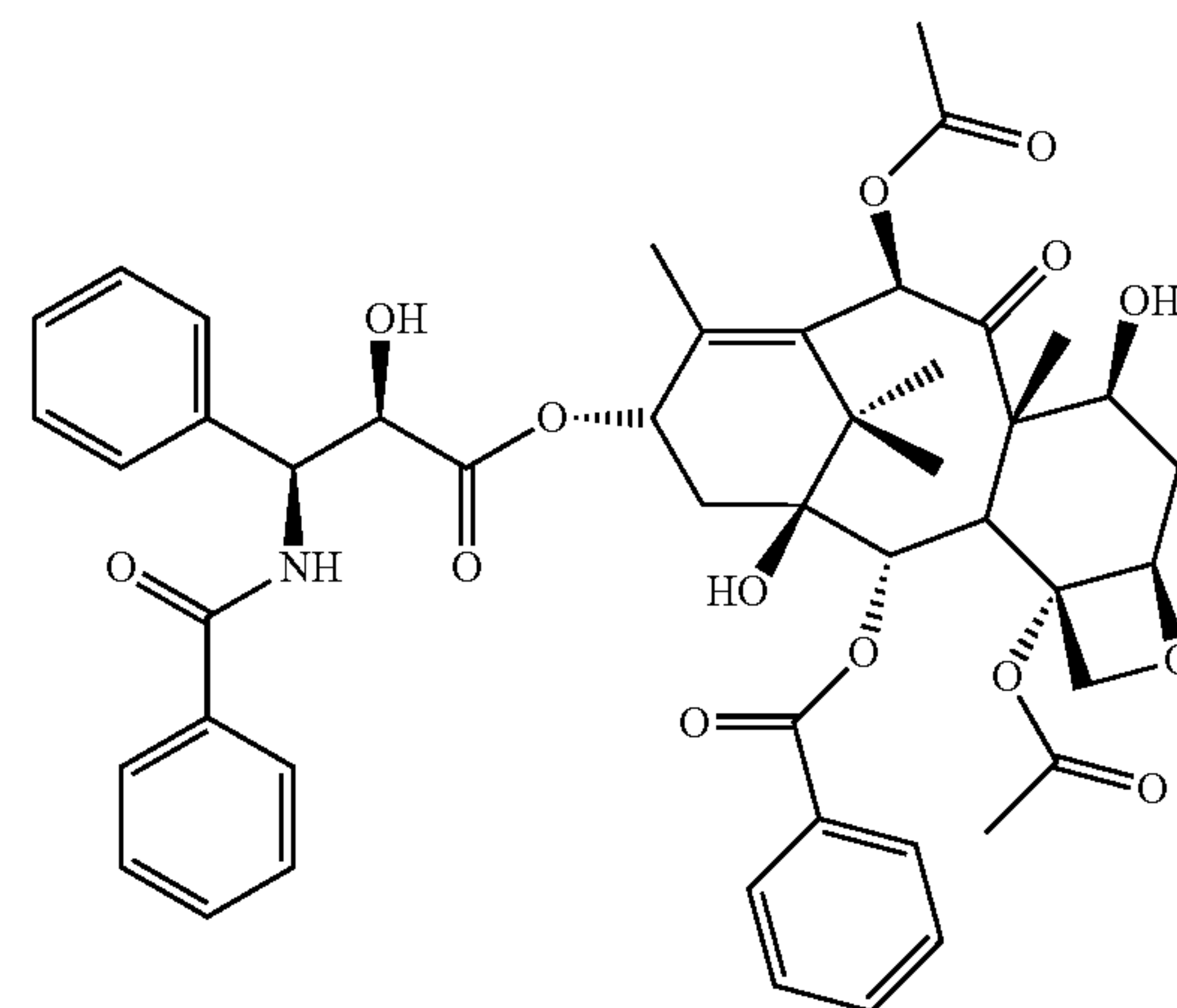
Paclitaxel
