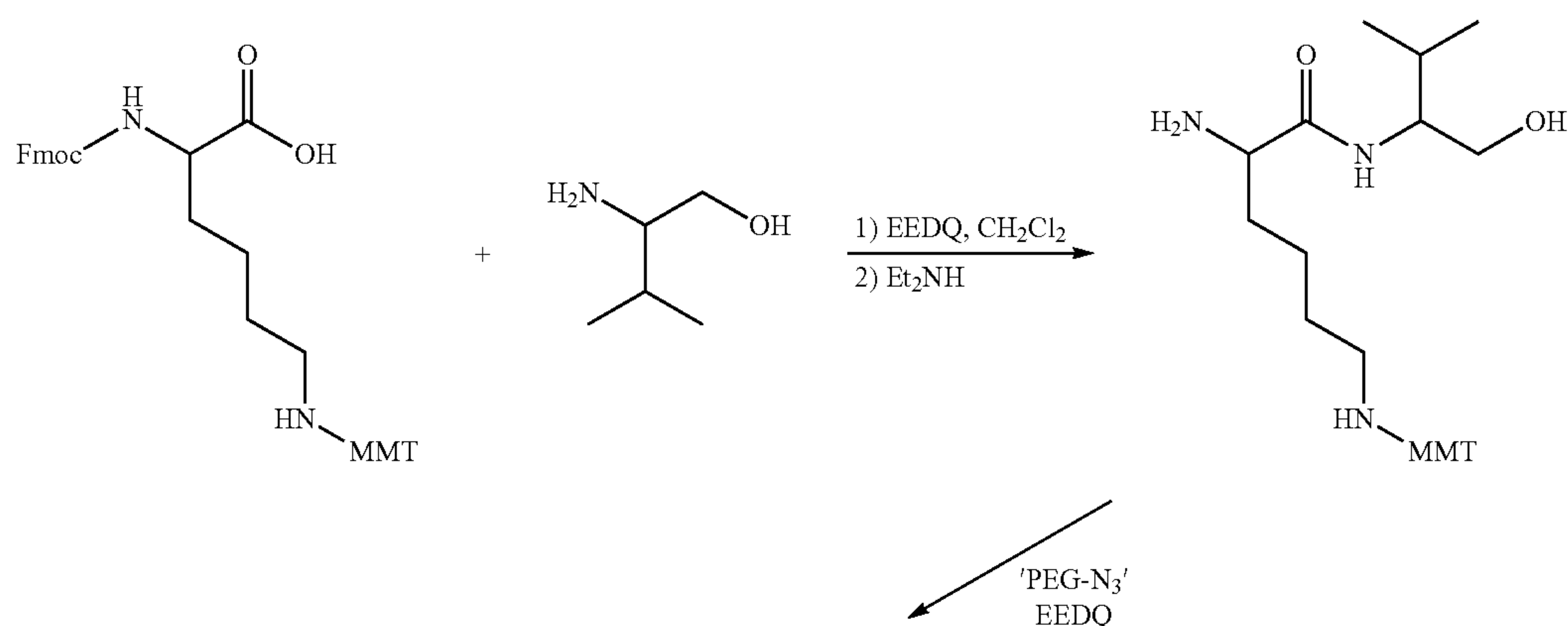
Scheme-2
