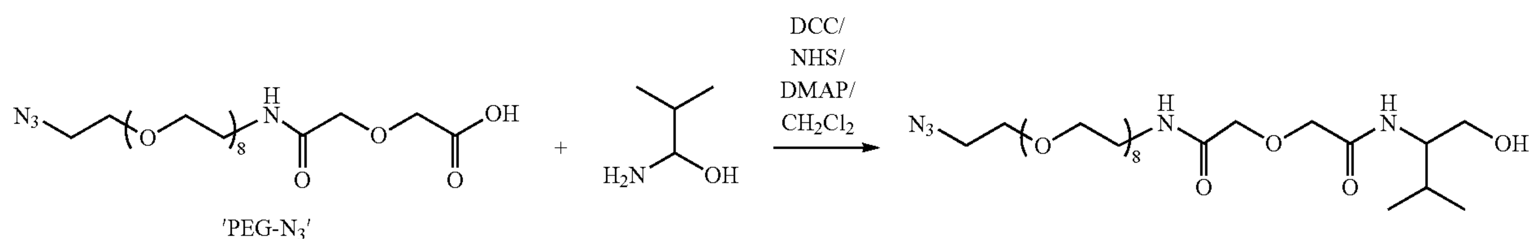
Scheme-1
