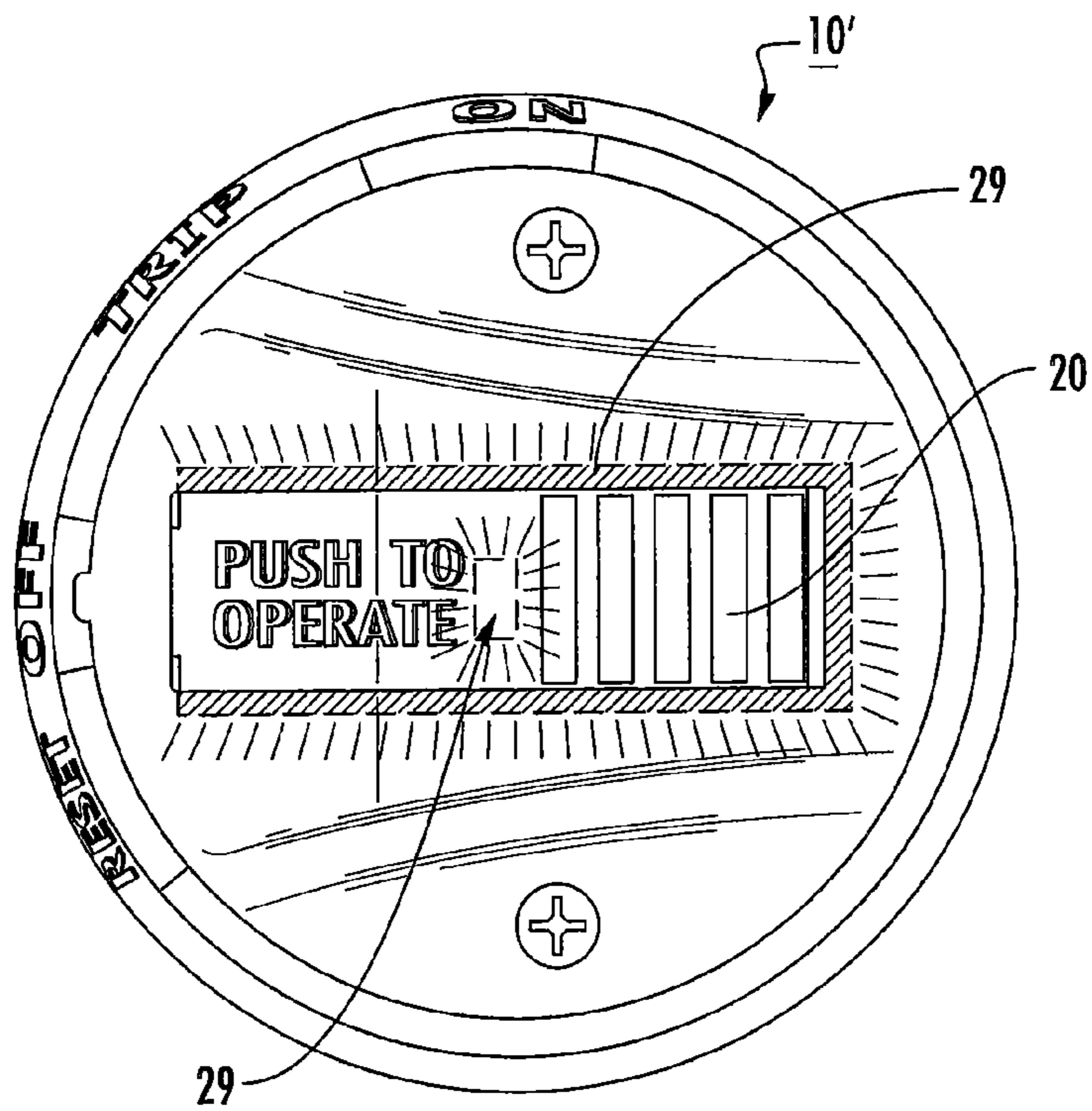
FIG. 13C
