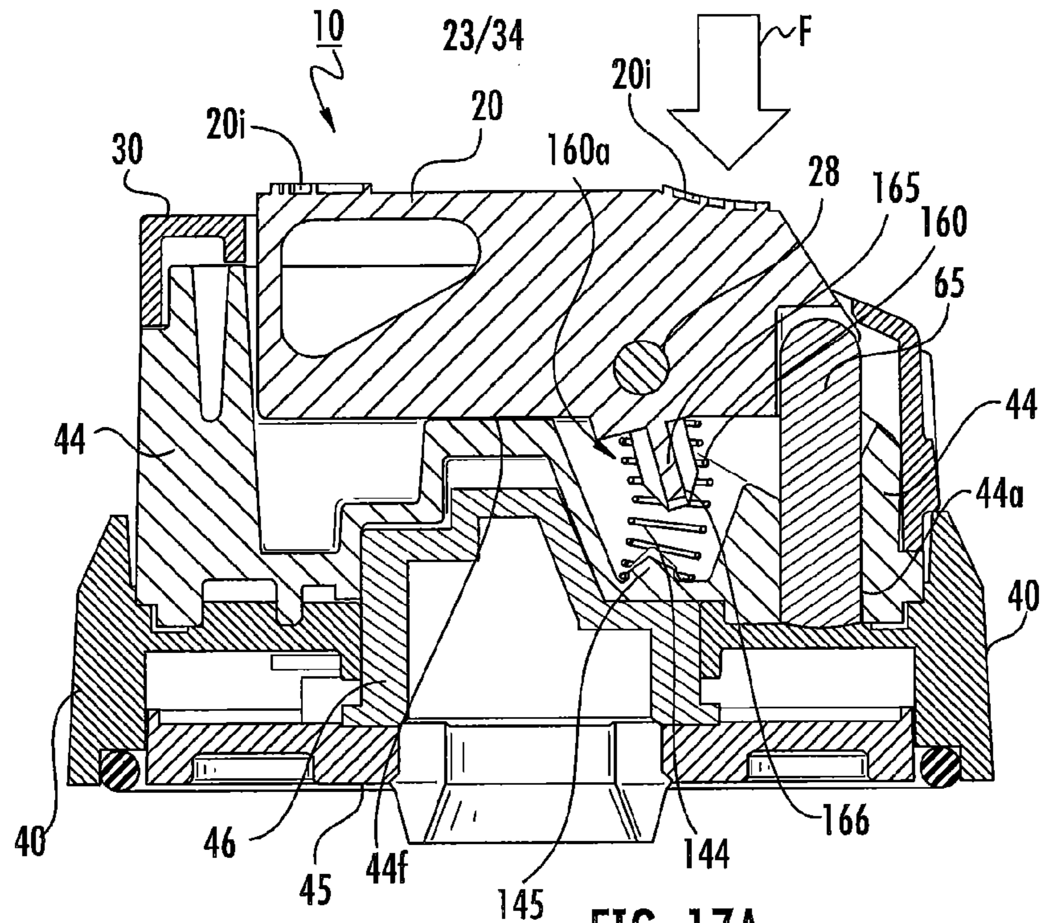
FIG. 17A
