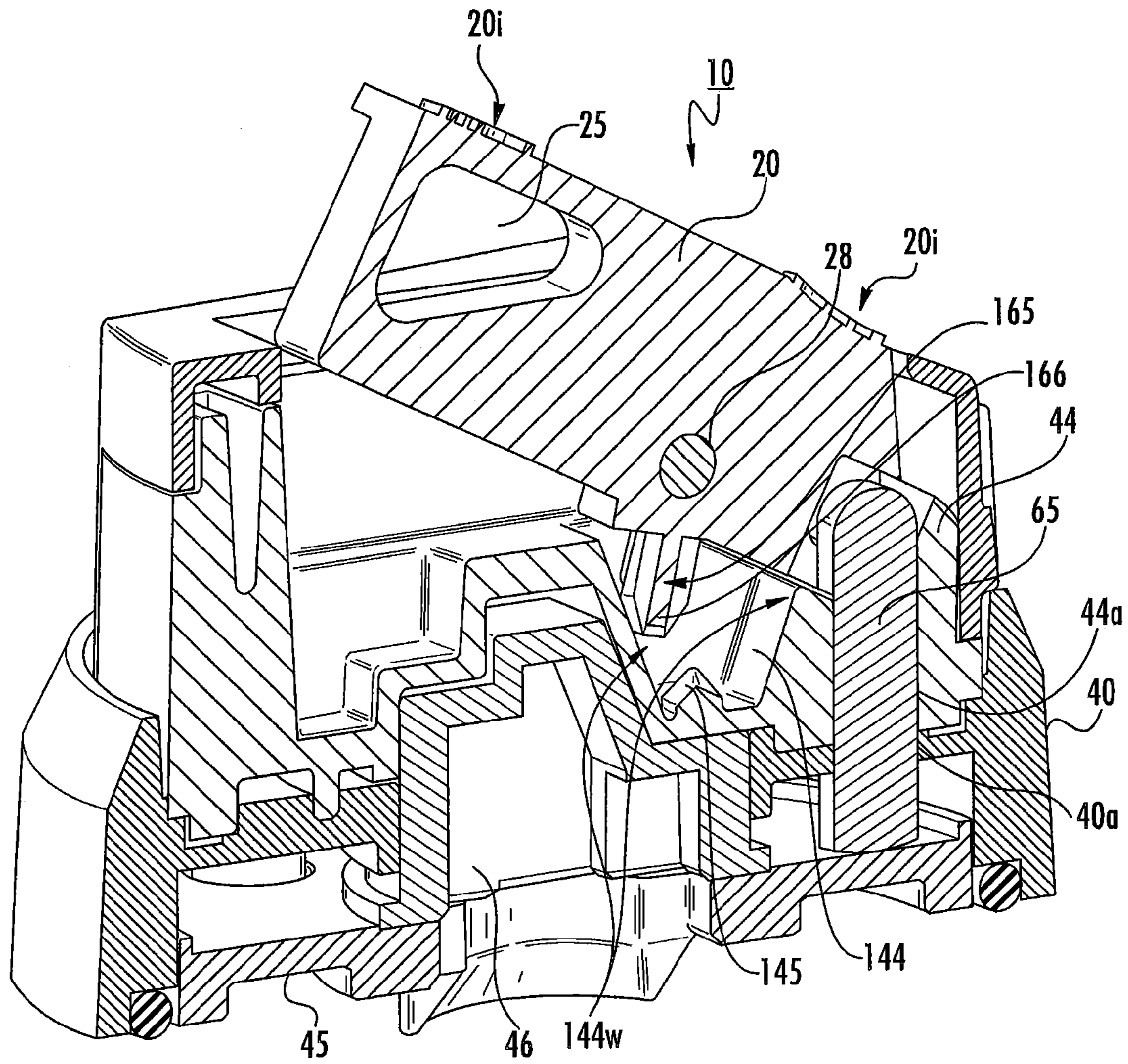
FIG. 18A
