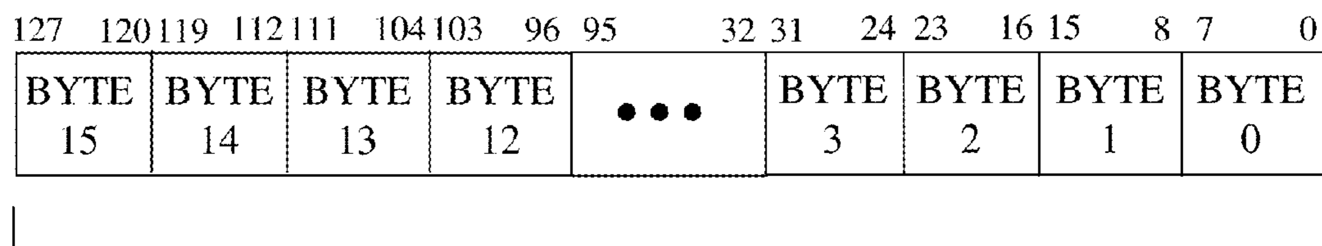
310 PACKED BYTE
