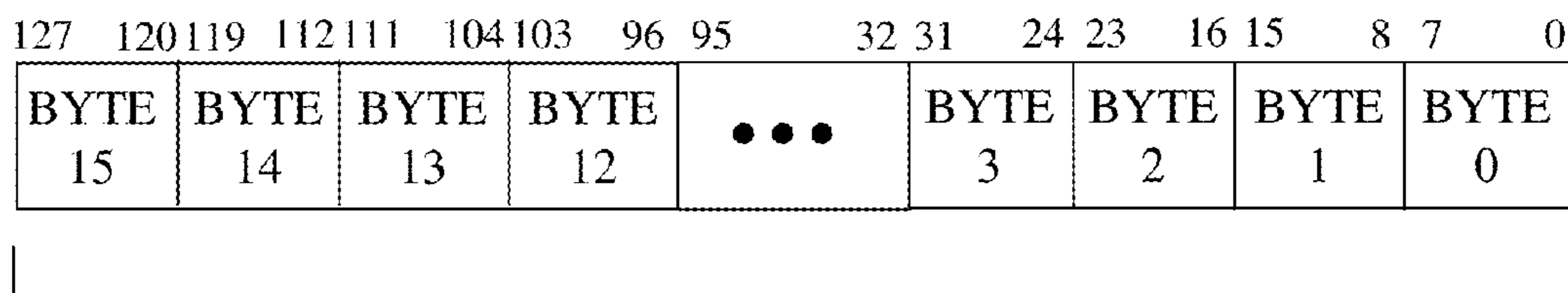
310 PACKED BYTE
