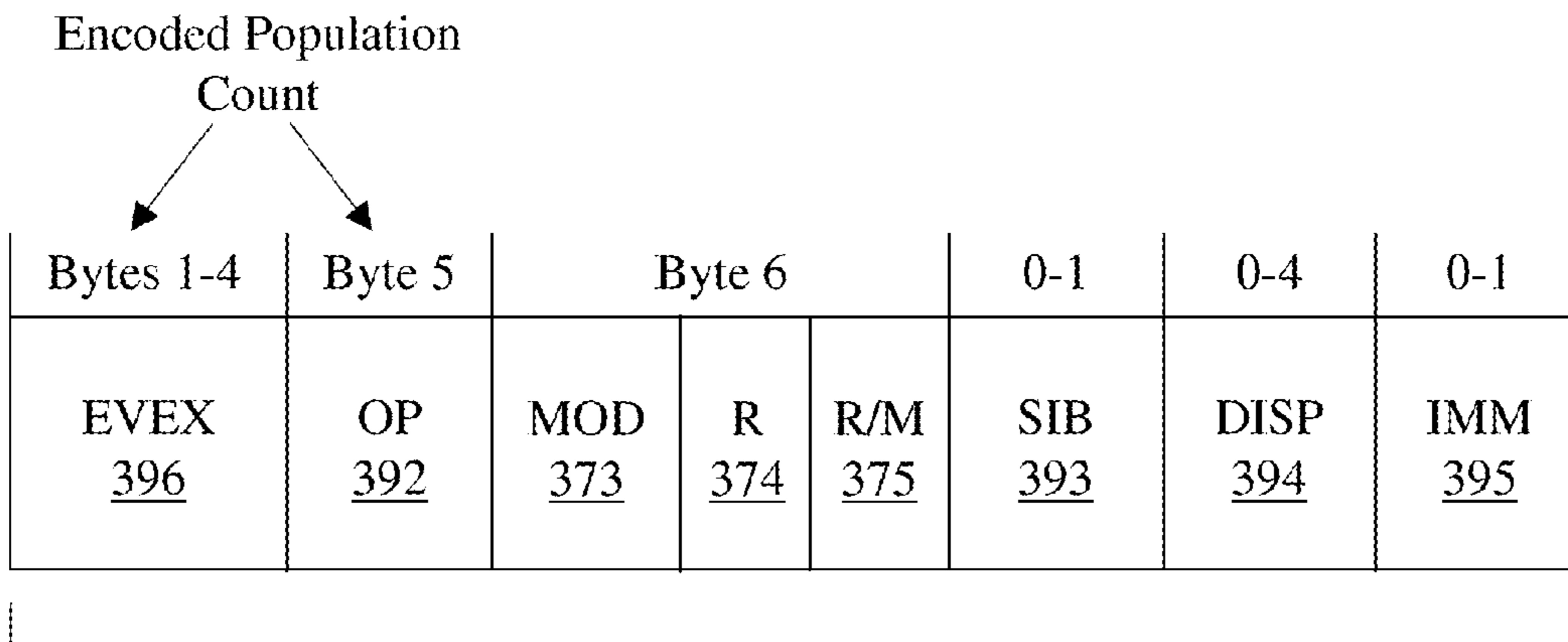
398 FIG. 3H
