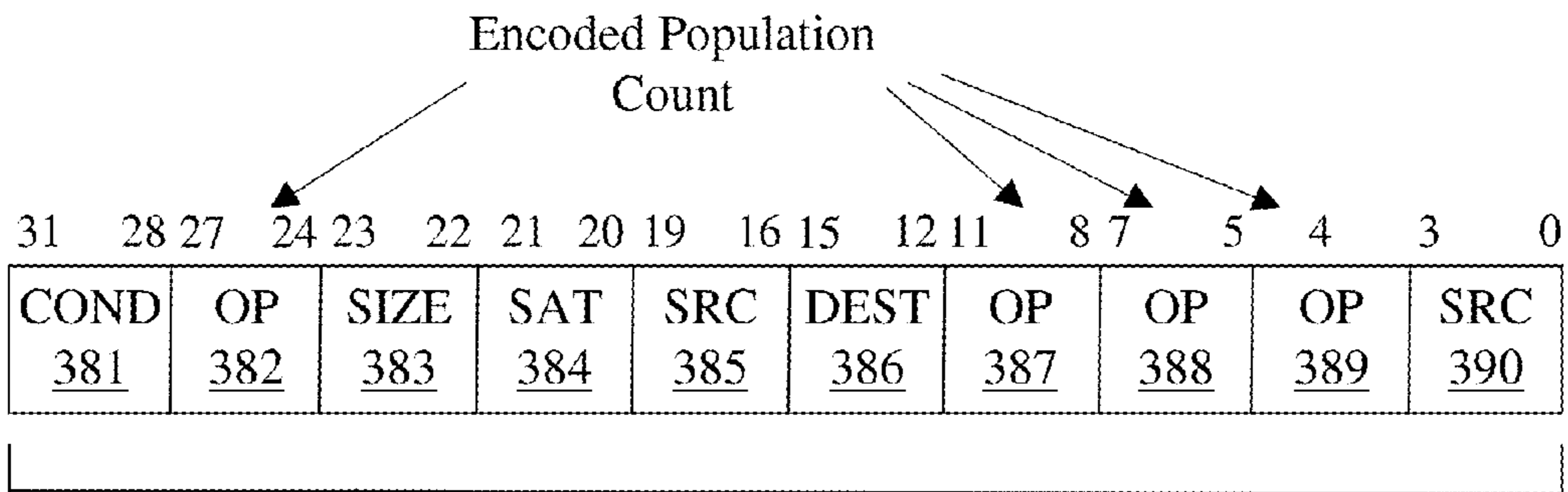
380 FIG. 3F
