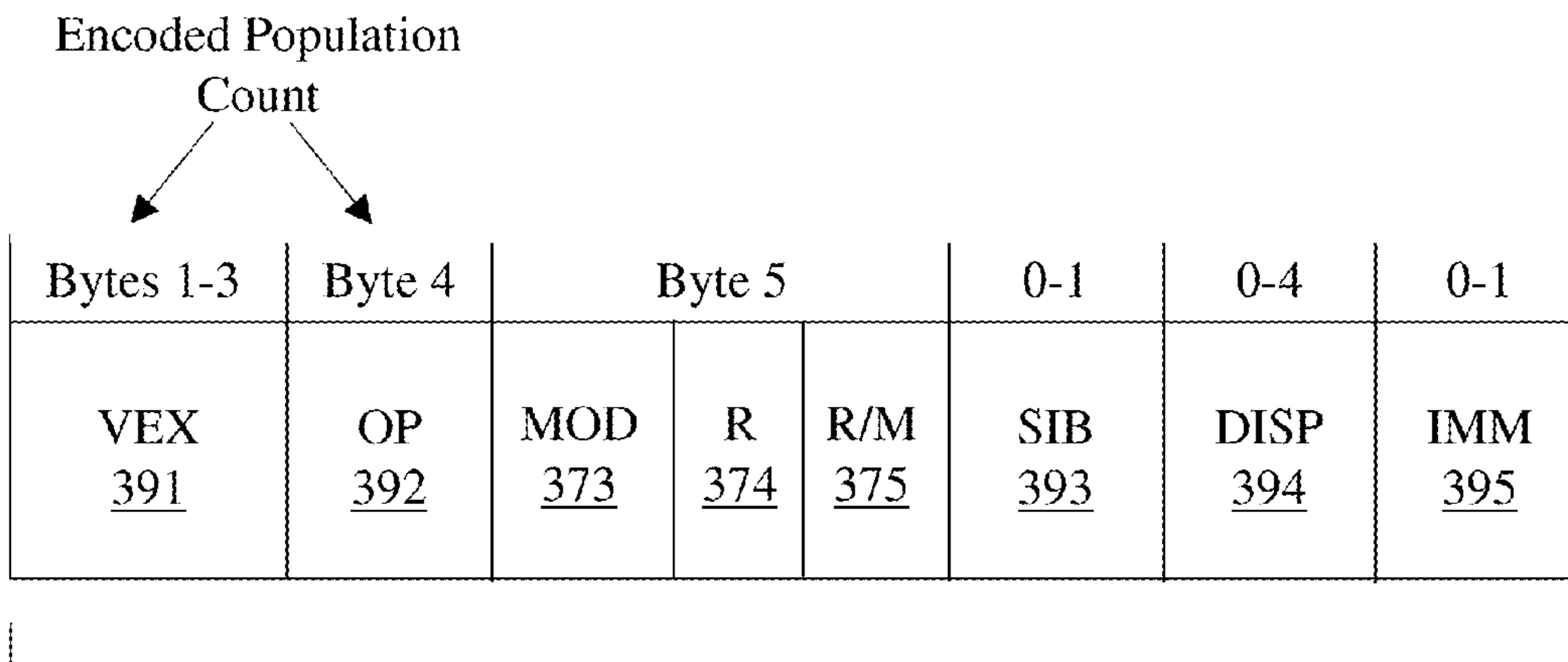
380 FIG. 3F
