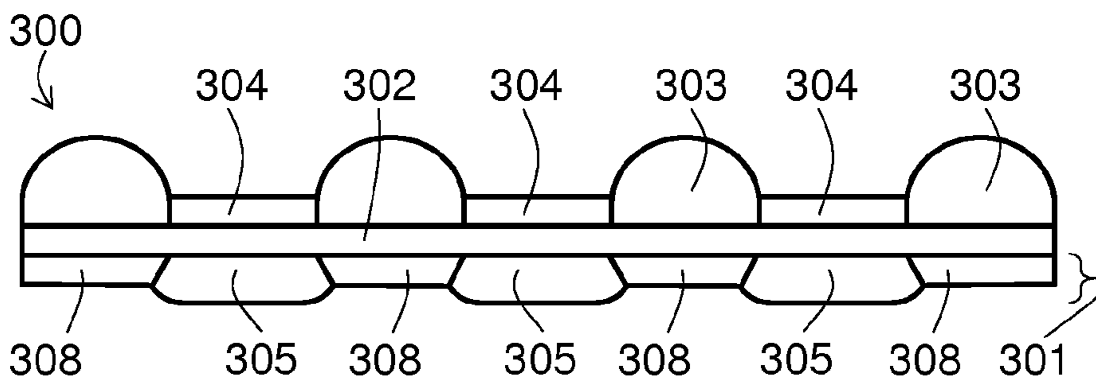
FIG. 29C
