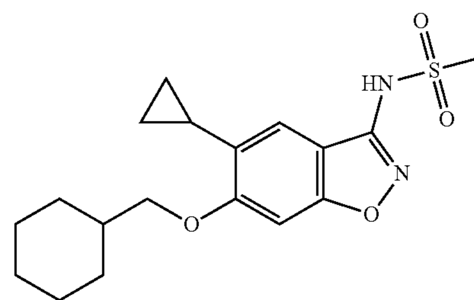
N-(6-(cyclohexylmethoxy)-5-cyclopropylbenzo[d]isoxazol-3-yl)methanesulfonamide
