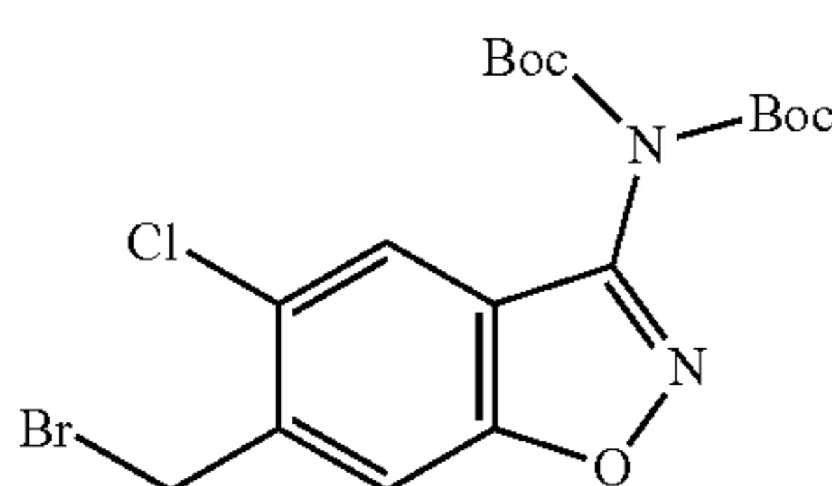
tert-butyl N-[6-(bromomethyl)-5-chloro-1,2-benzoxazol-3-yl]-N-[(tert-butoxy)carbonyl]carbamate
