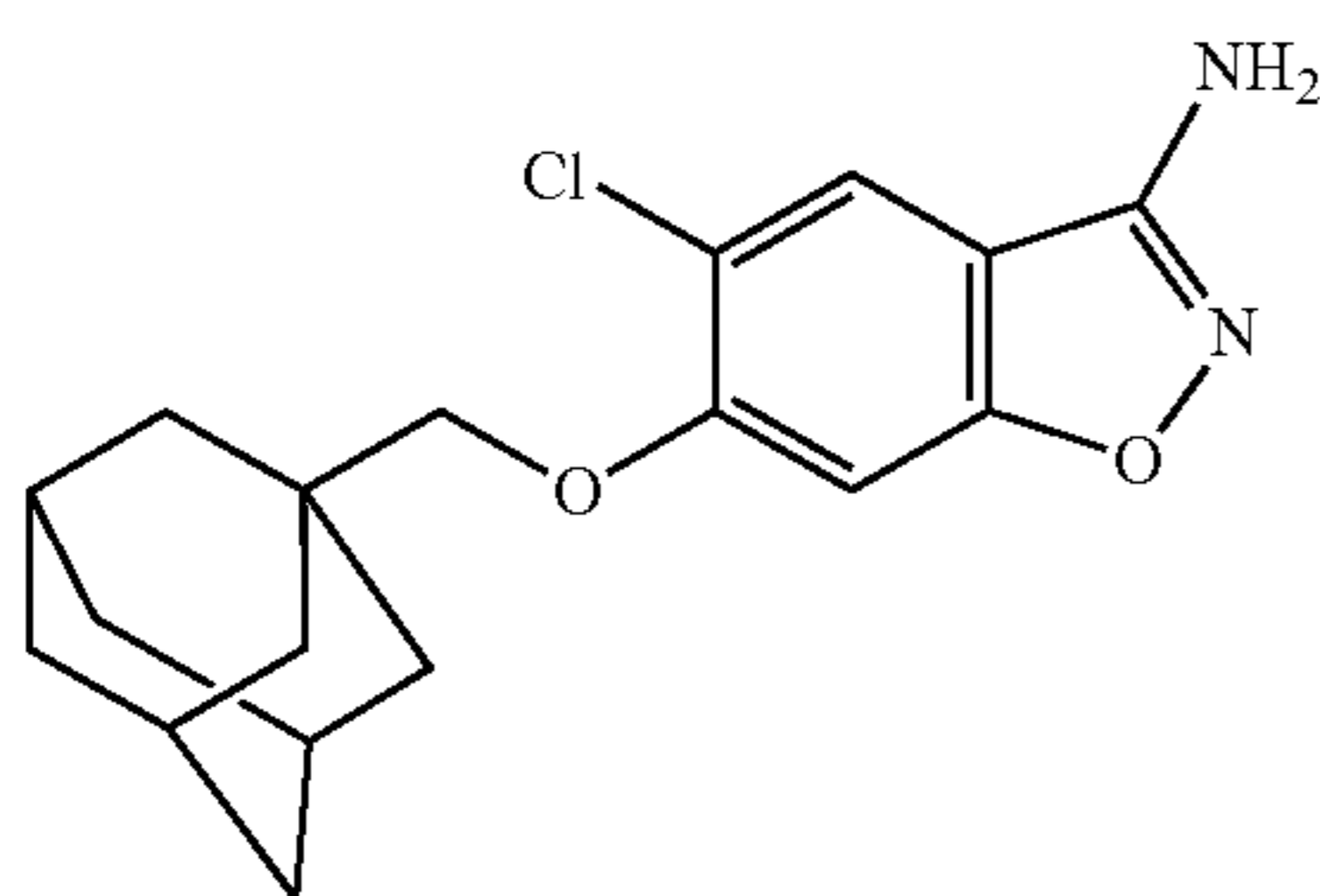
6-(adamantan-1-ylmethoxy)-5-chloro-1,2-benzoxazol-3-amine
