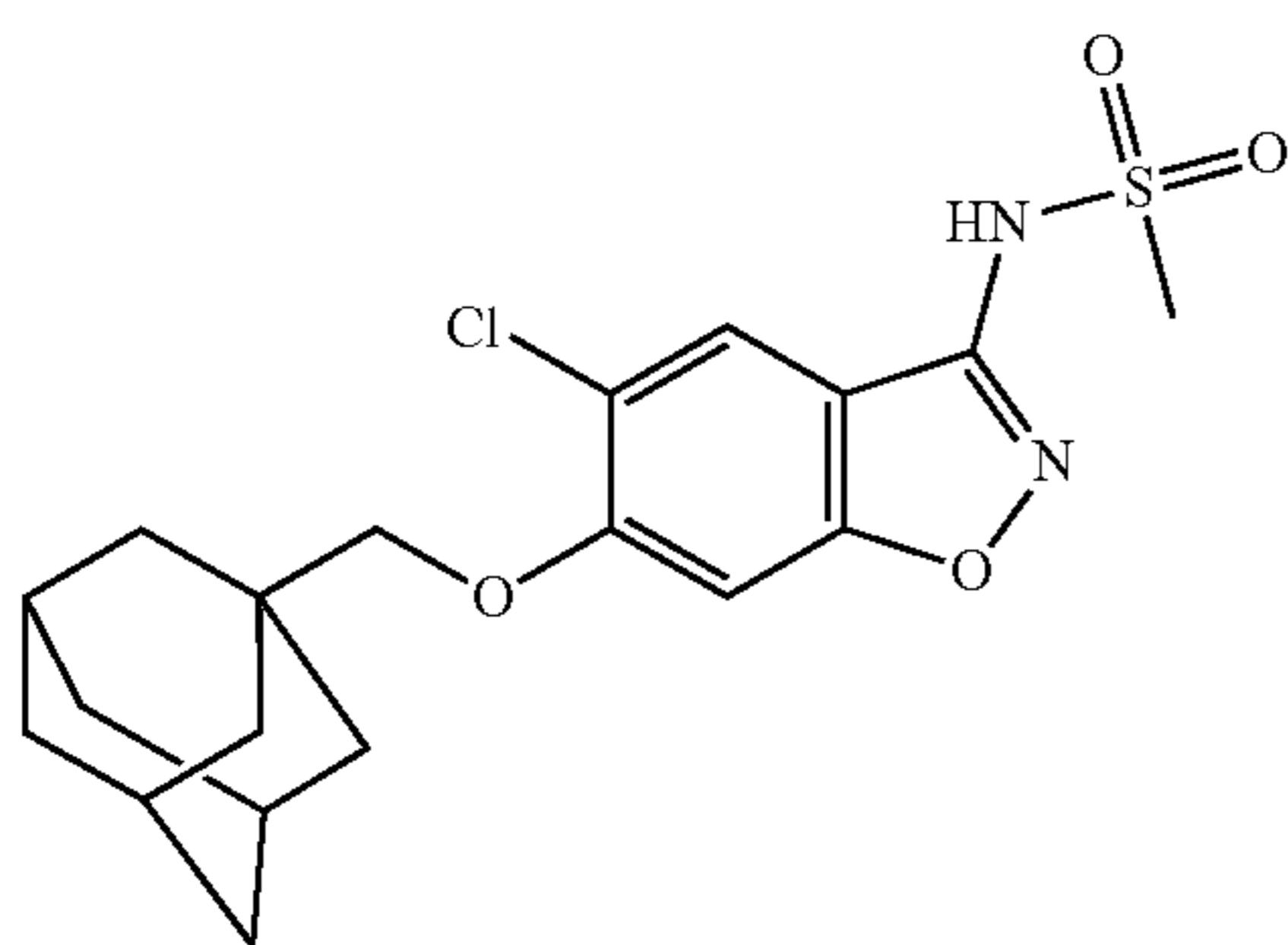
N -[6-(adamantan-1-ylmethoxy)-5-chloro-1,2-benzoxazol-3-yl]methanesulfonamide
