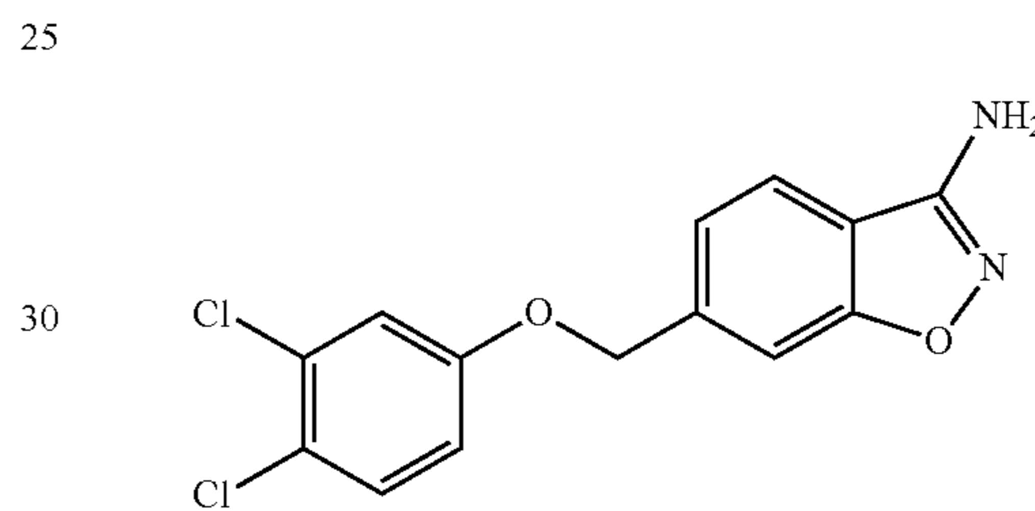
6-((3,4-dichlorophenoxy)methyl)benzo[d]isoxazol-3-amine
