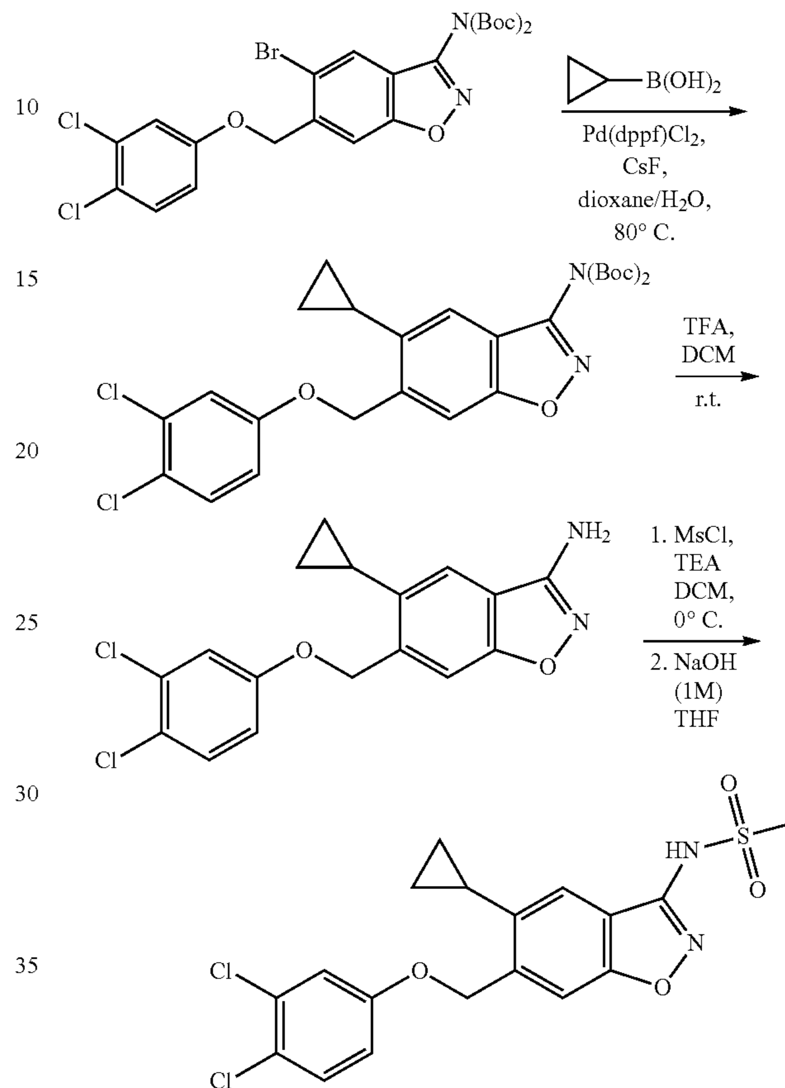
N-(6-((3,4-dichlorophenoxy)methyl)-5-methylbenzo[d]isoxazol-3-yl)methanesulfonamide
