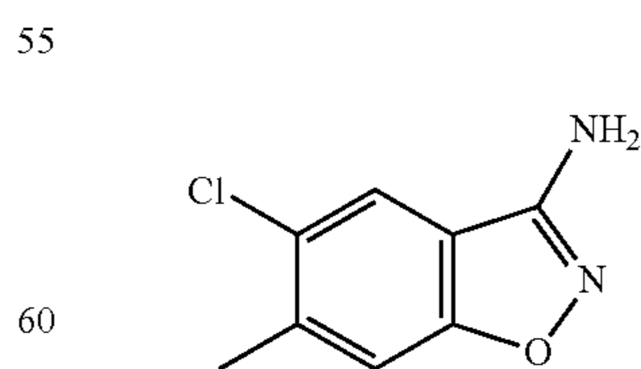
5-chloro-6-methylbenzo[d]isoxazol-3-amine
