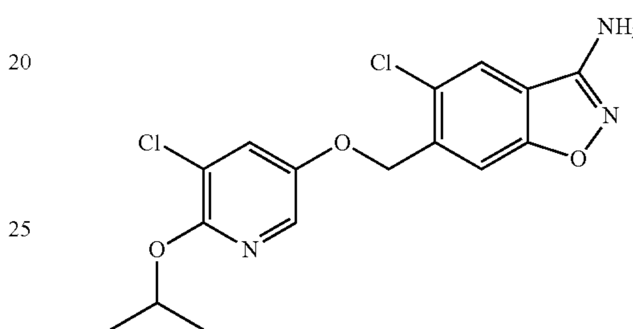
5-chloro-6-((5-chloro-6-isopropoxy-pyridin-3-yl)oxy)methyl)benzo[d]isoxazol-3-amine
