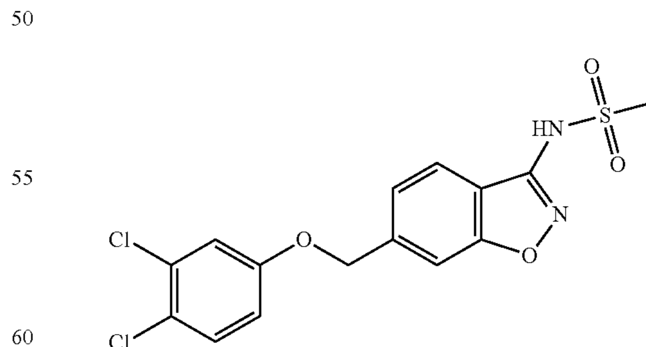
N-(6-((3,4-dichlorophenoxy)methyl)benzo[d]isoxazol-3-yl)methanesulfonamide
