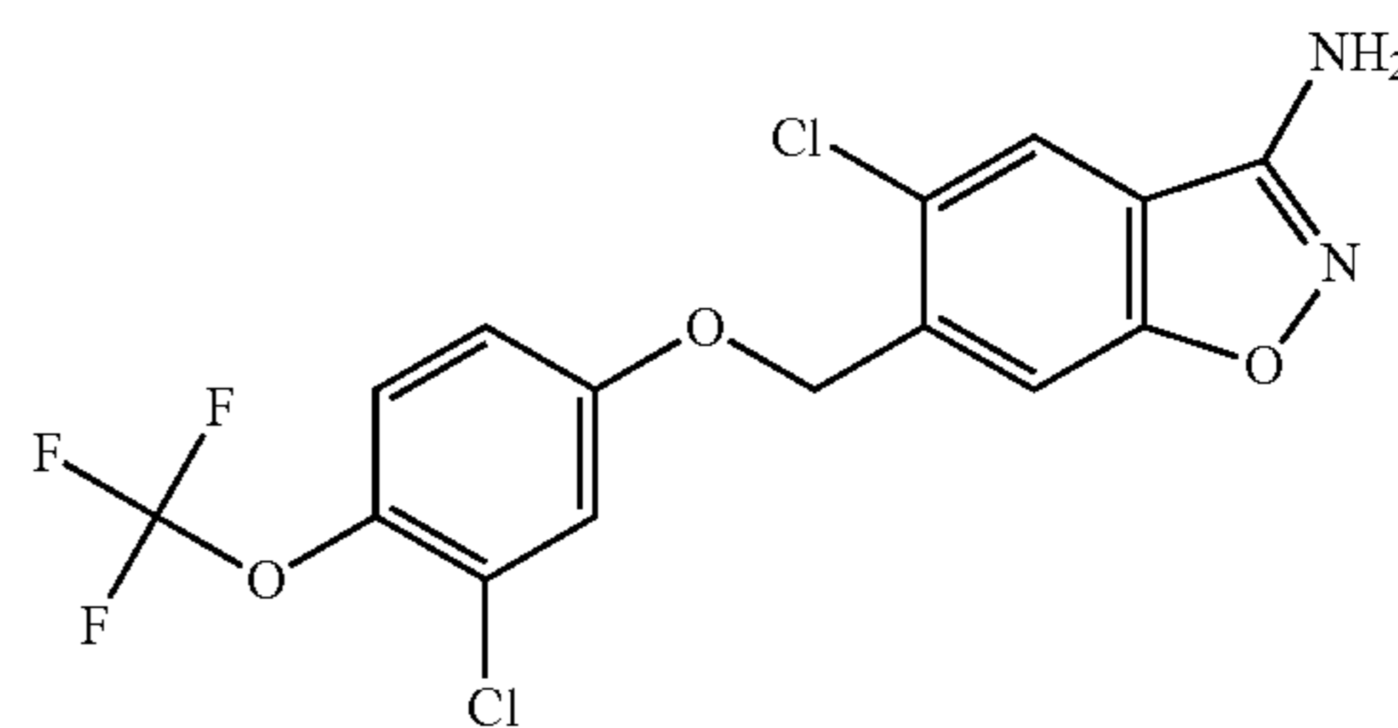
5-chloro-6-[3-chloro-4-(trifluoromethoxy)phenoxy)methyl]-1,2-benzoxazol-3-amine
