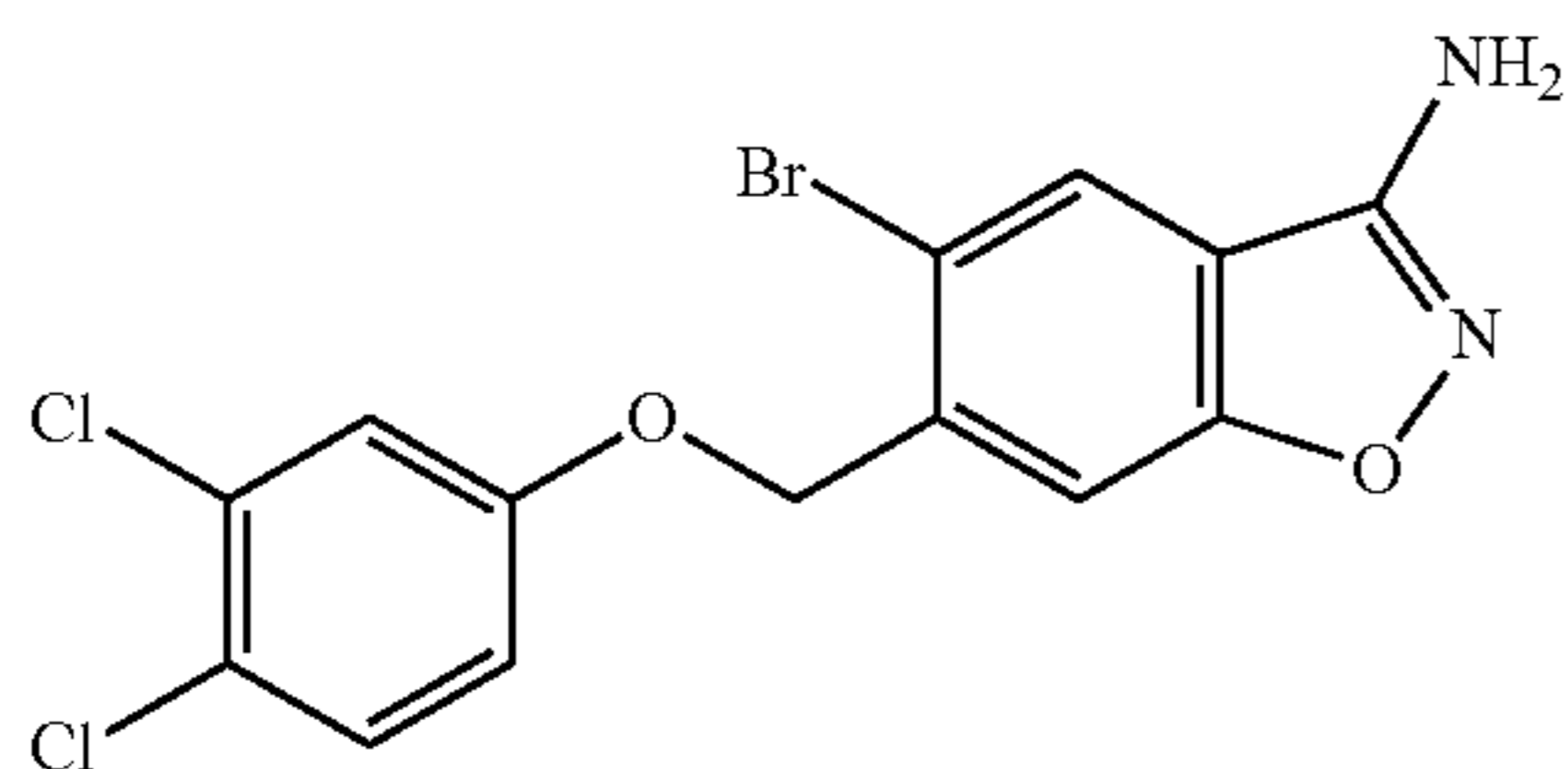
5-bromo-6-((3,4-dichlorophenoxy)methyl)benzo[d]isoxazol-3-amine
