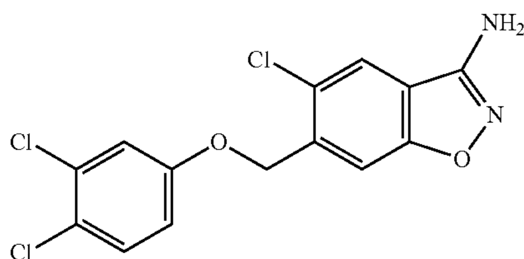
5-chloro-6-((3,4-dichlorophenoxy)methyl)benzo[d]isoxazol-3-amine
