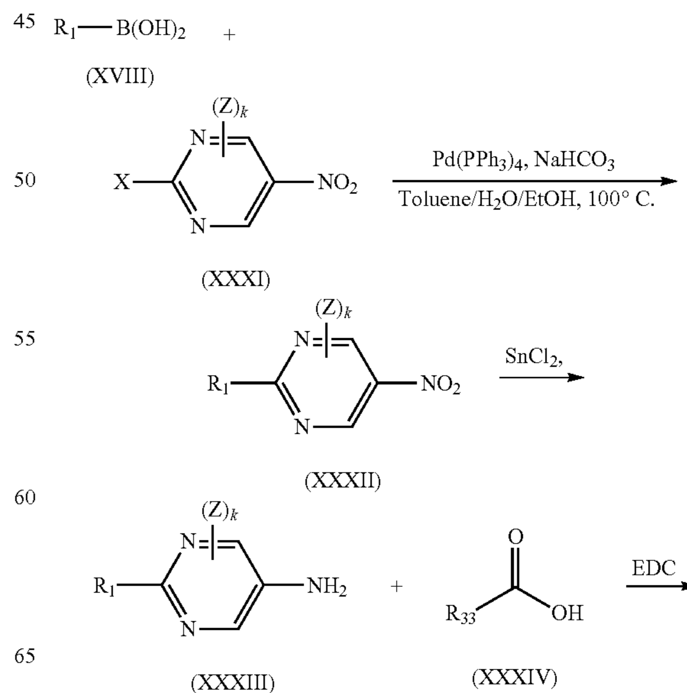
Scheme VI
