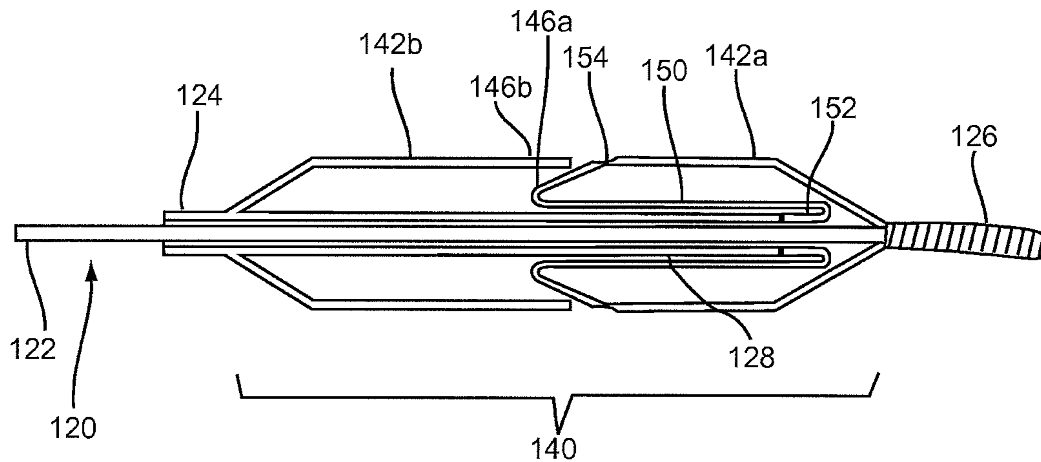
FIG. 4D
