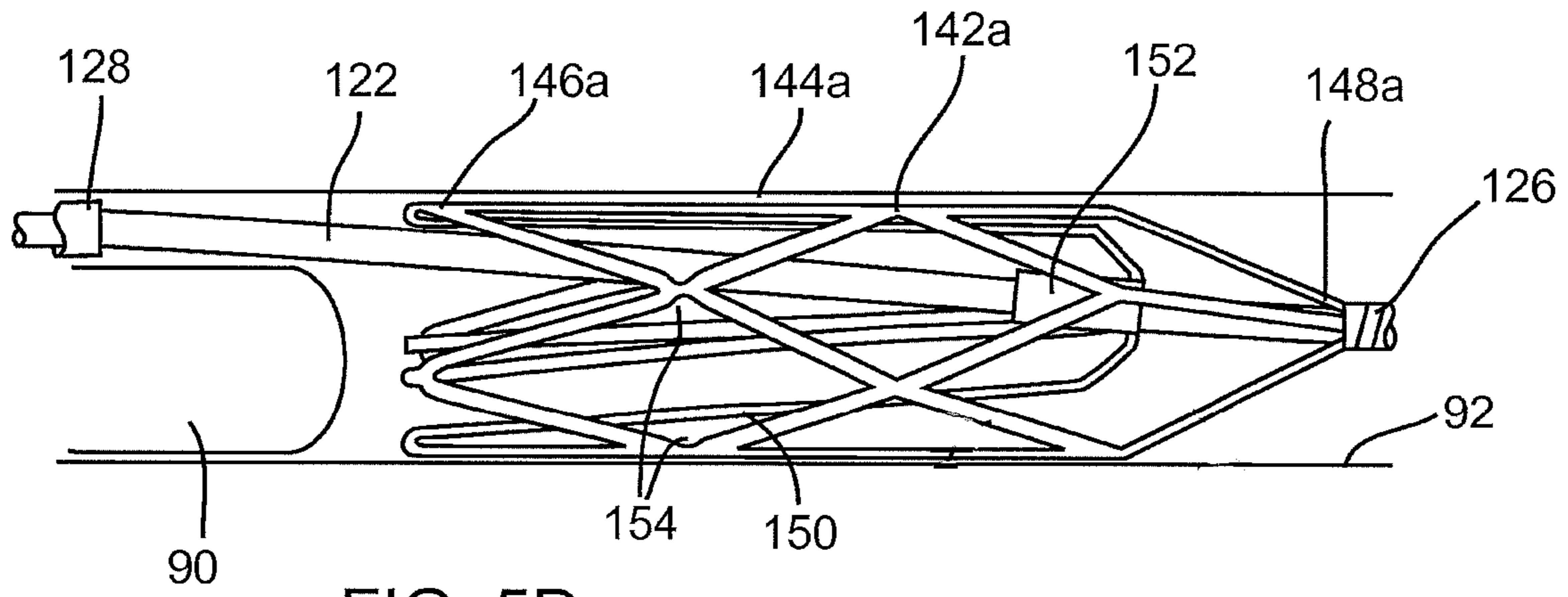
FIG. 5D
