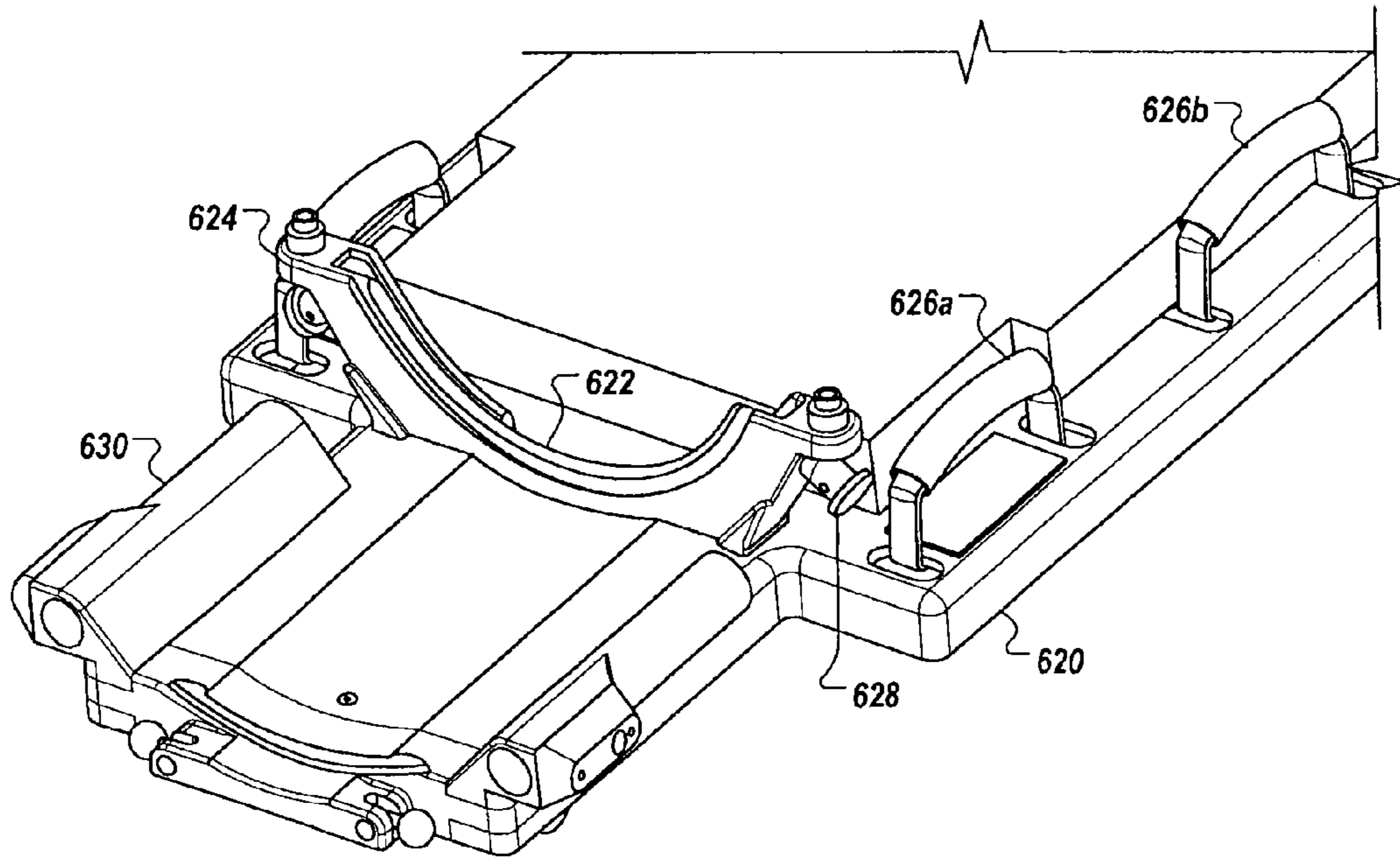
FIG. 6D
