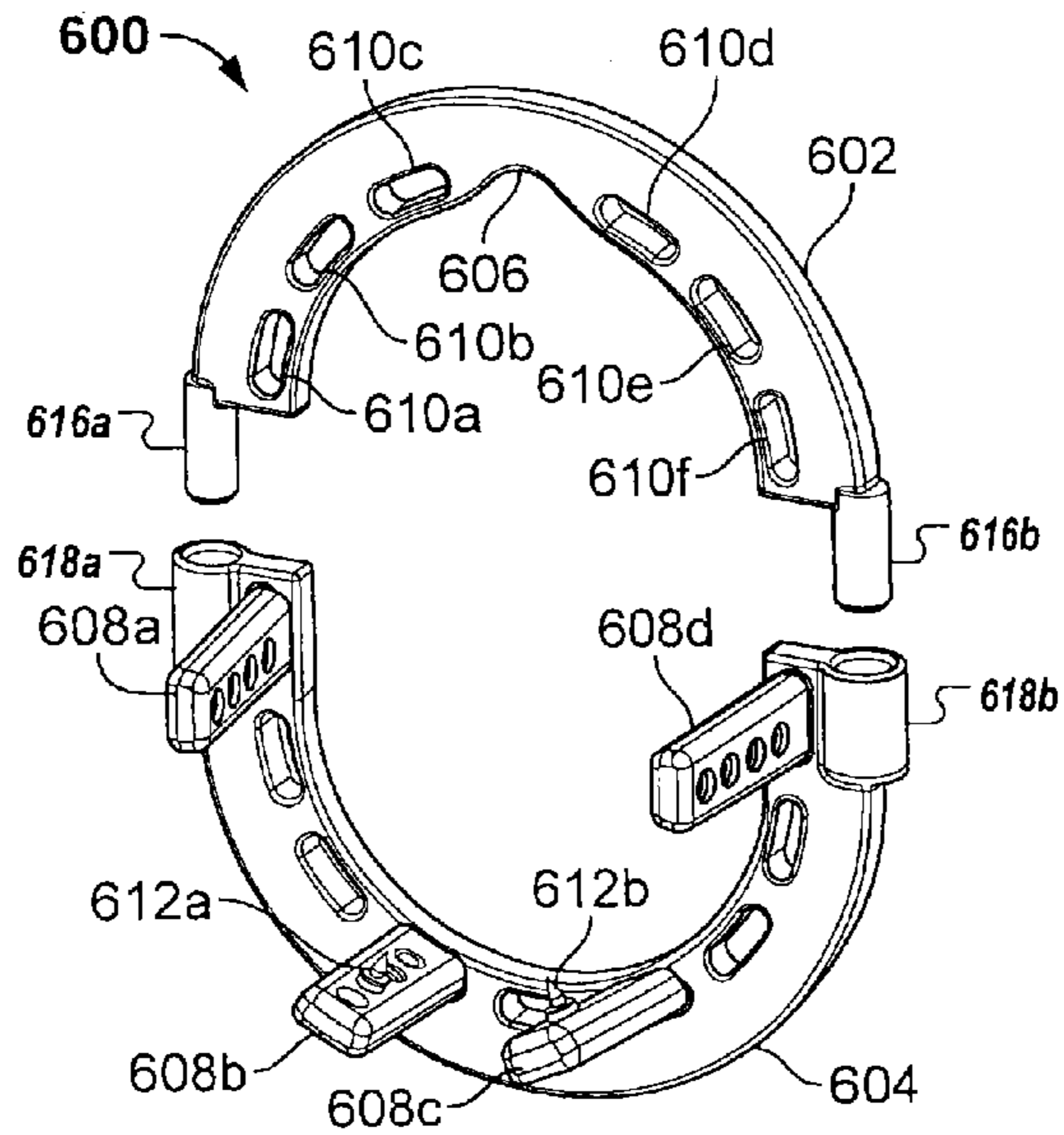
FIG. 6A
