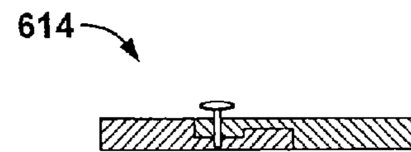
FIG. 6C
