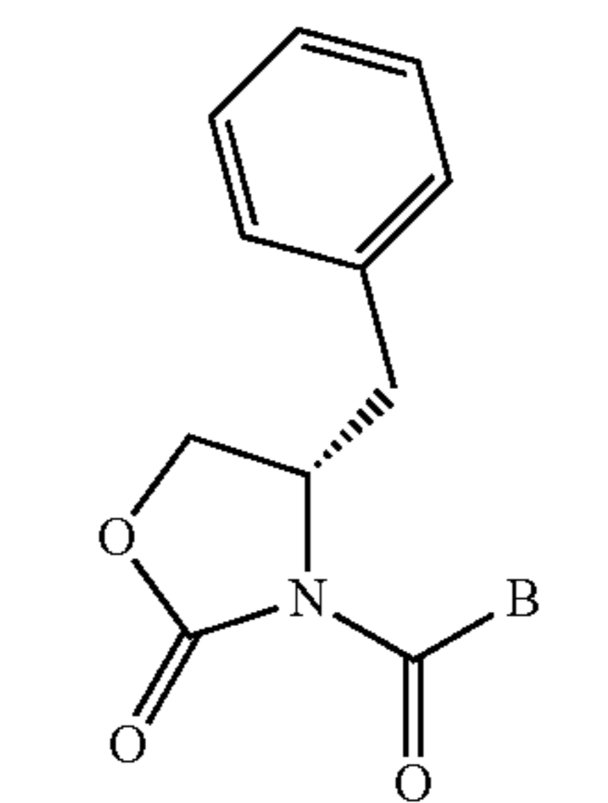
(S)-3-(B-Carbonyl)-4-benzyloxazolidin-2-ones
