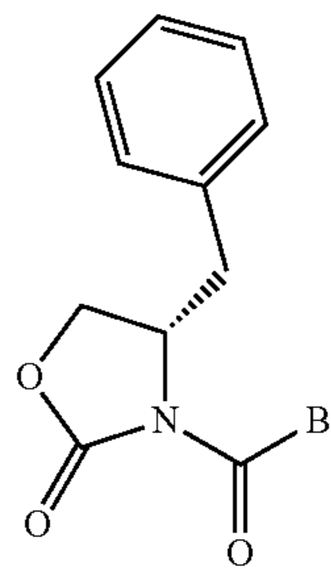
(S)-3-(B-Carbonyl)- 4-benzyloxazolidin-2-ones
