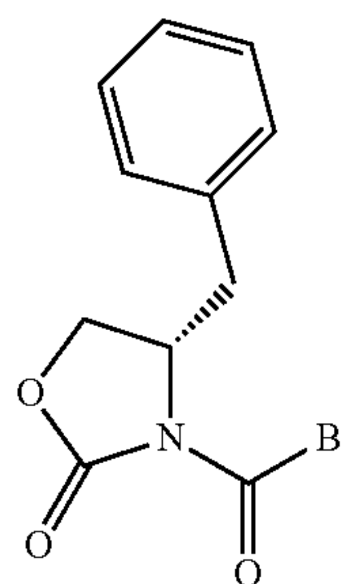
(S)-3-(B-Carbonyl)-4-benzyloxazolidin-2-ones
