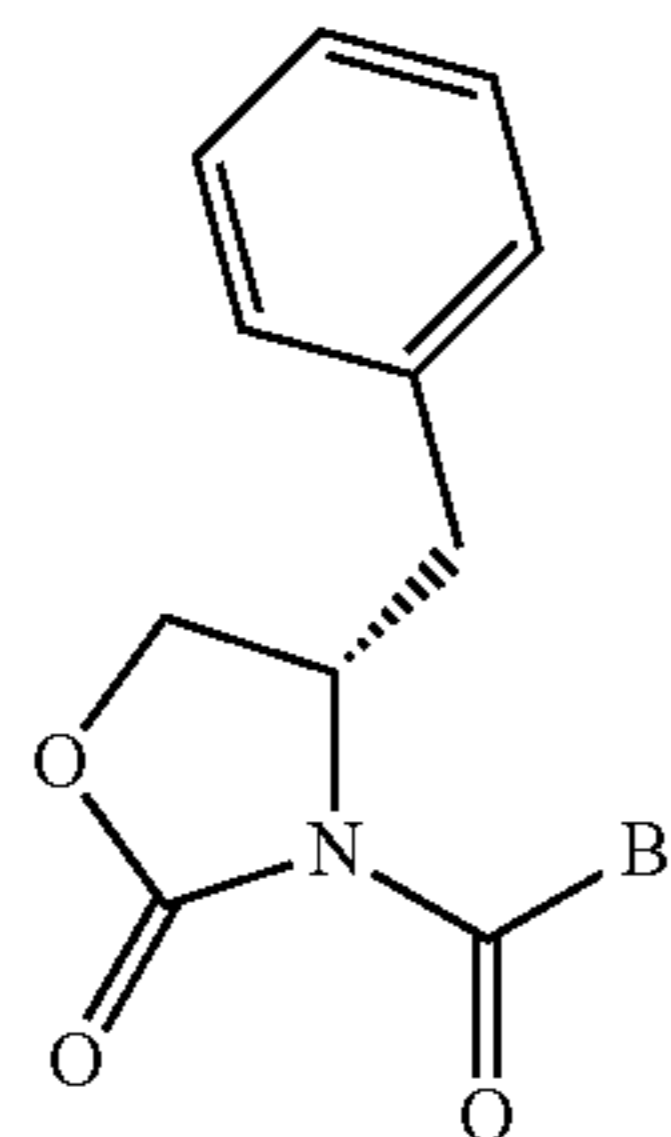
(S)-3-(B-Carbonyl)-4-benzyloxazolidin-2-ones
