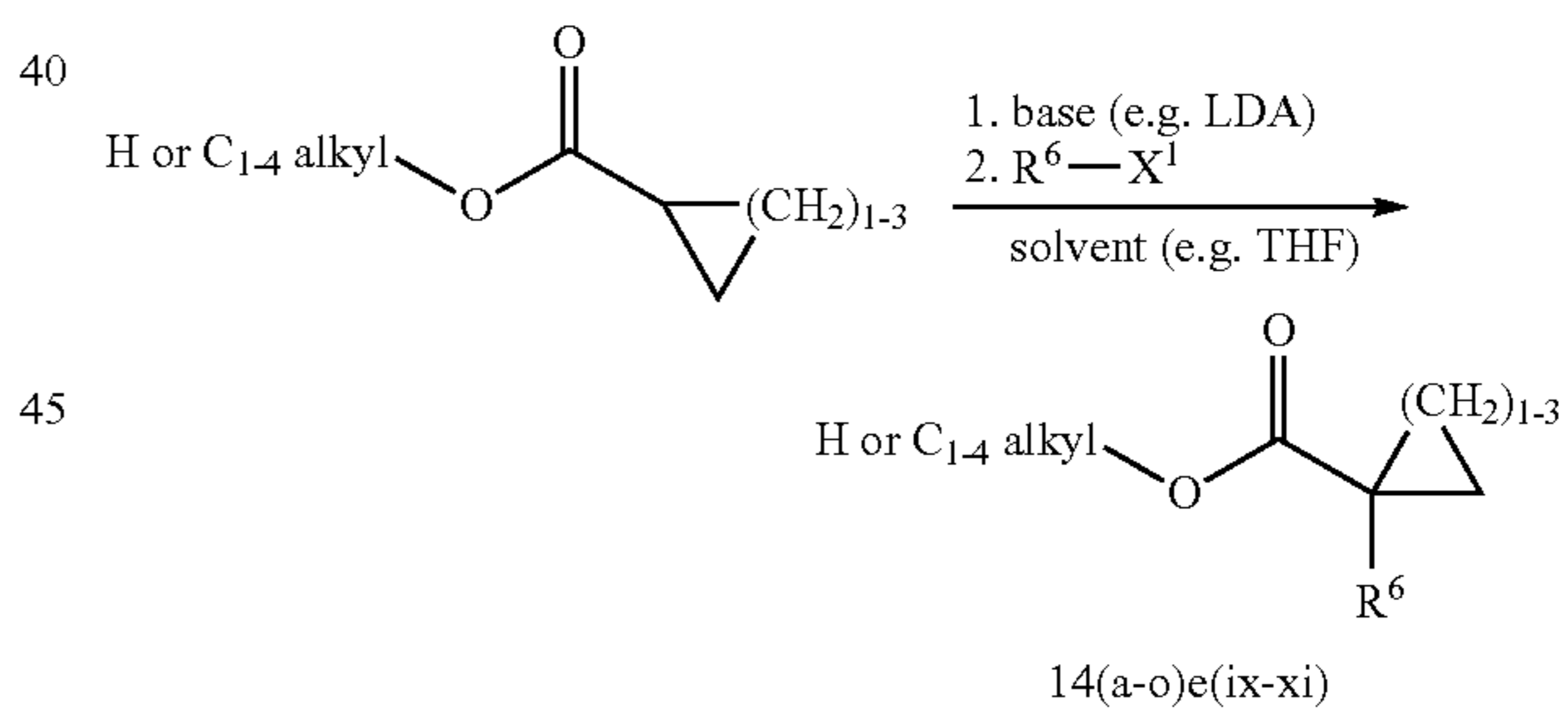
Scheme 7e
