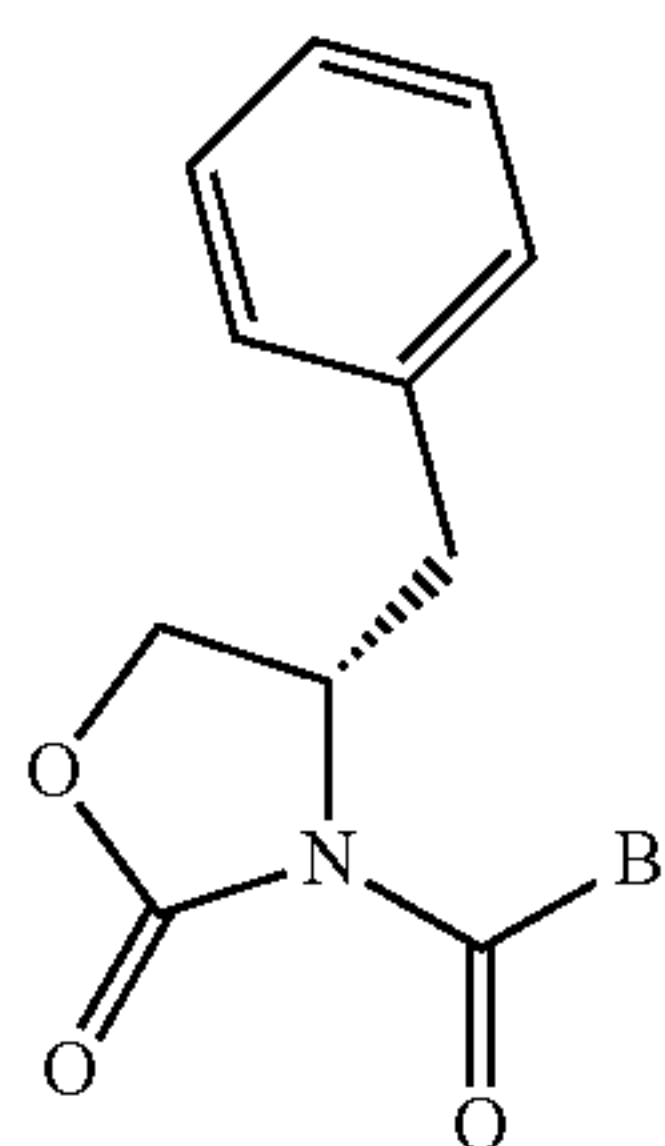
(S)-3-(B-Carbonyl)-4-benzyloxazolidin-2-ones
