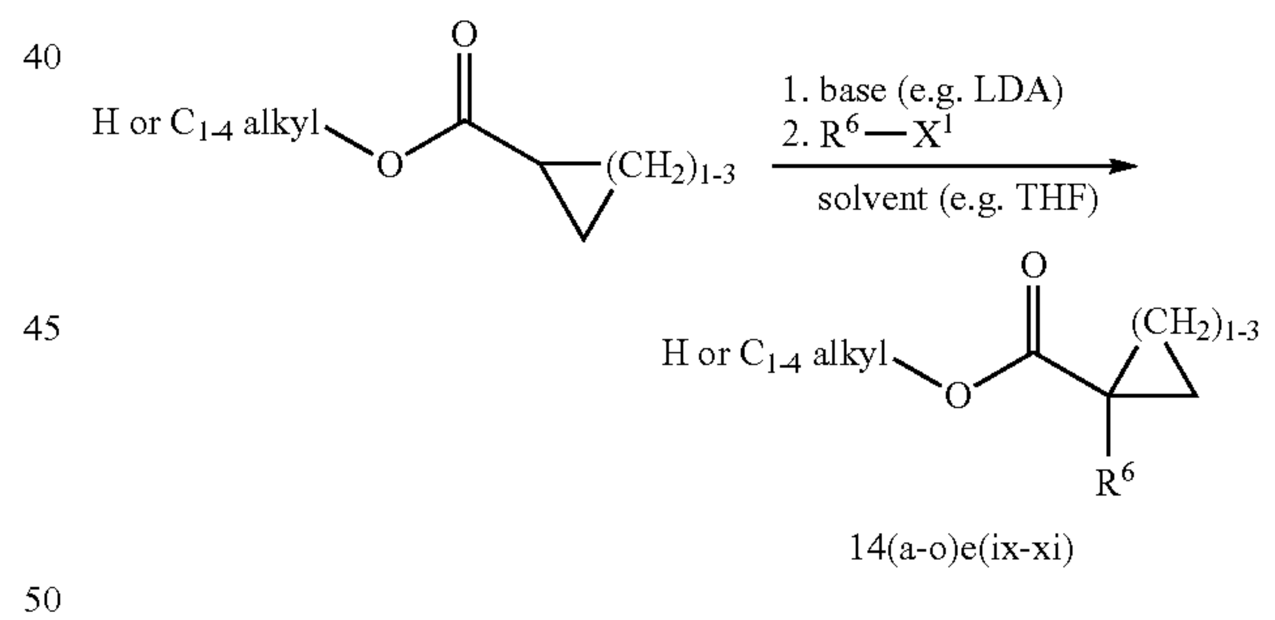
Scheme 7e
