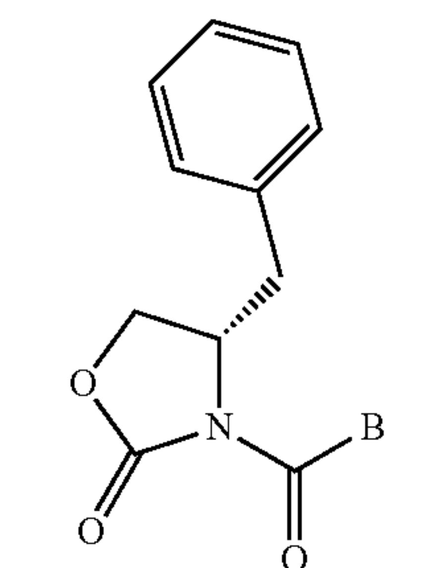
(S)-3-(B-Carbonyl)-4-benzyloxazolidin-2-ones
