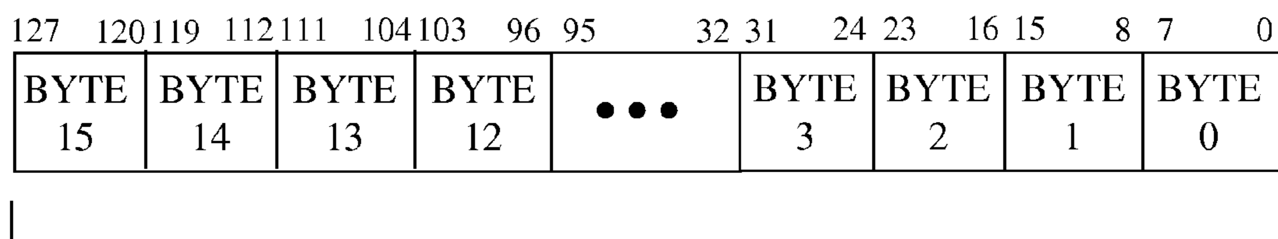
310 Packed Byte
