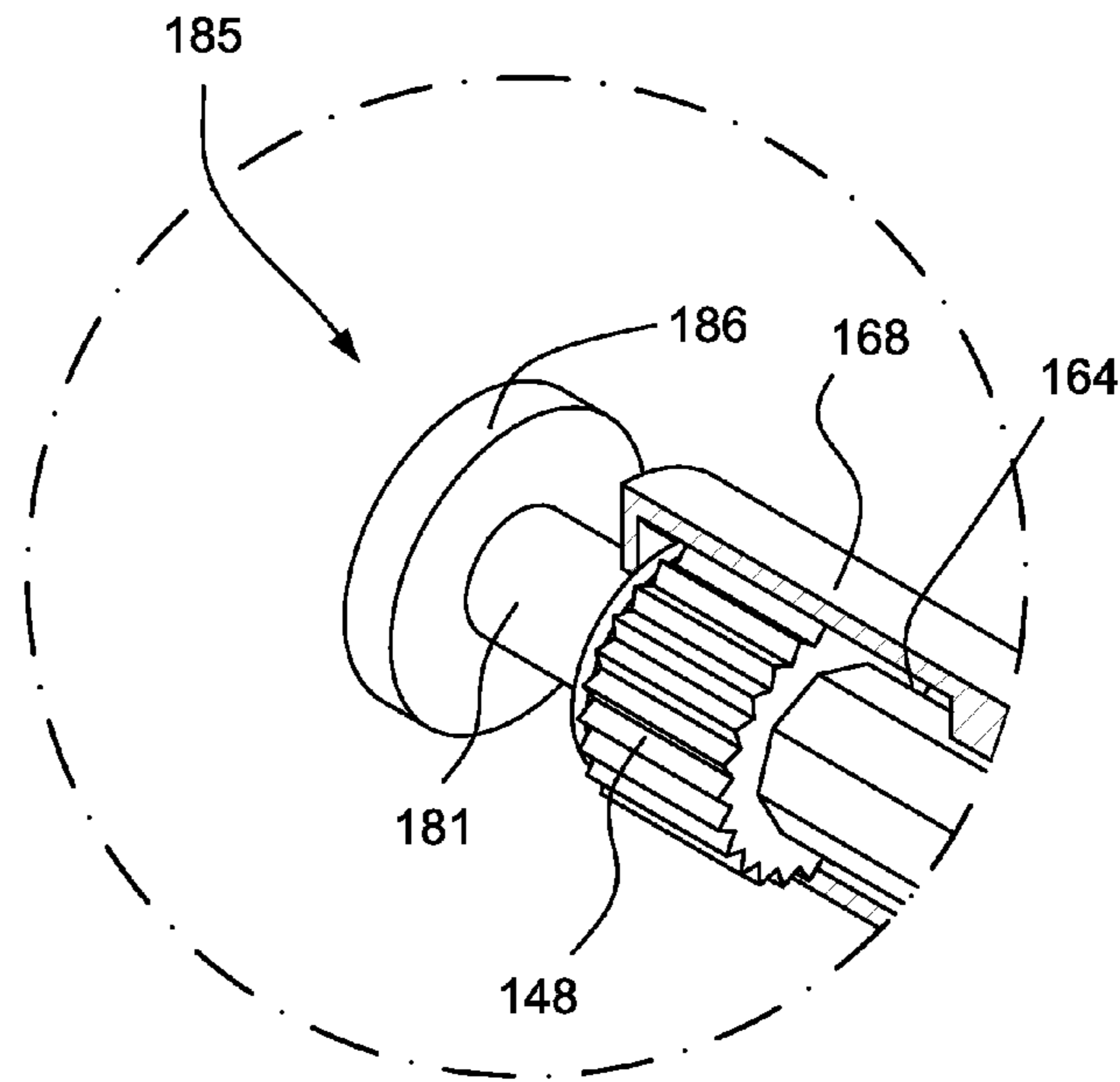
FIG. 29B (Push Button In)
