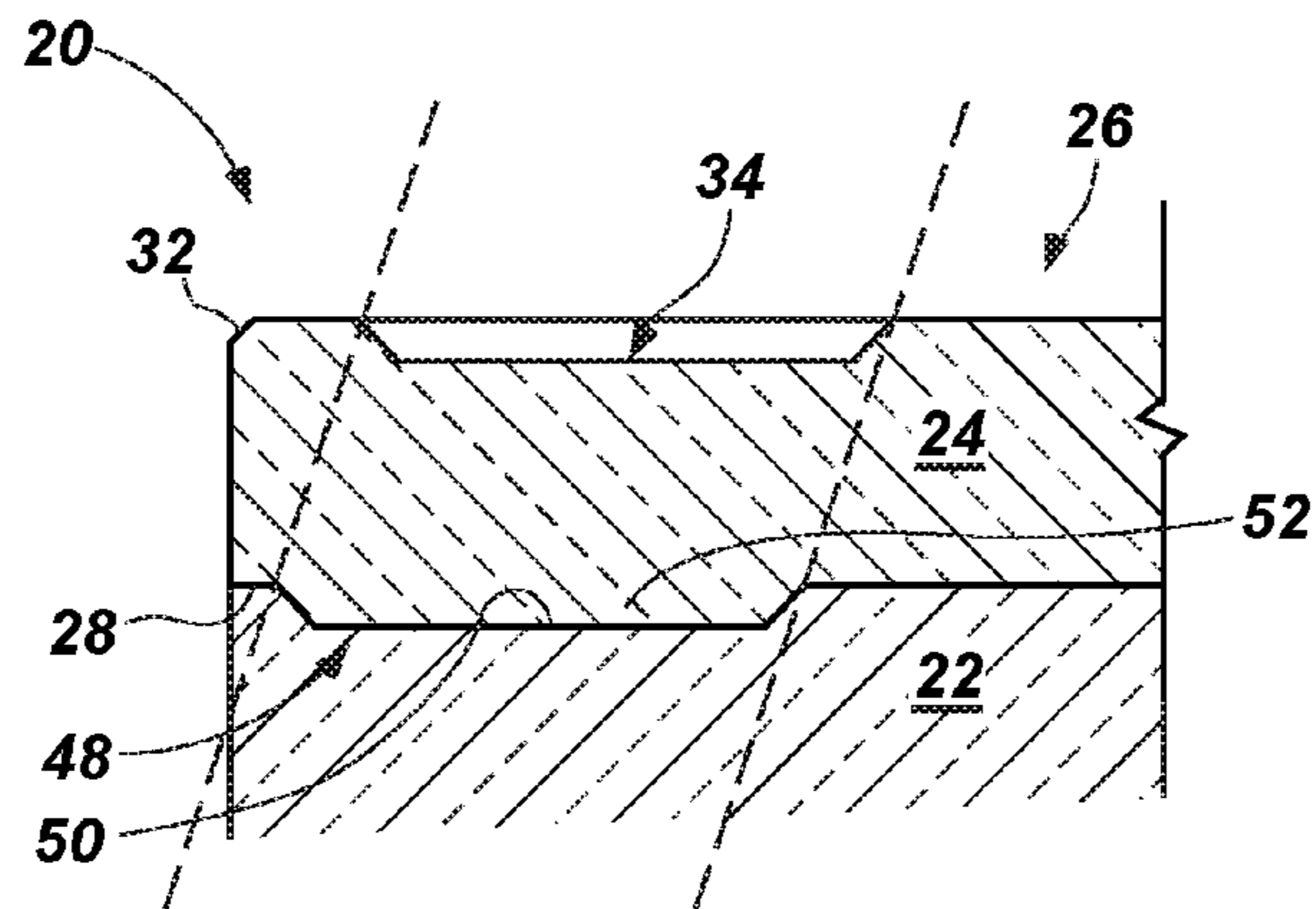
FIG. 26
