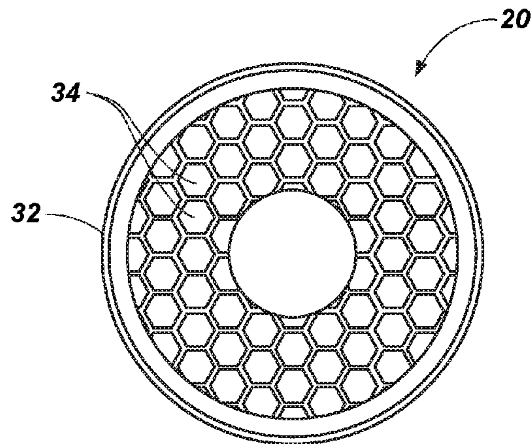
FIG. 15
