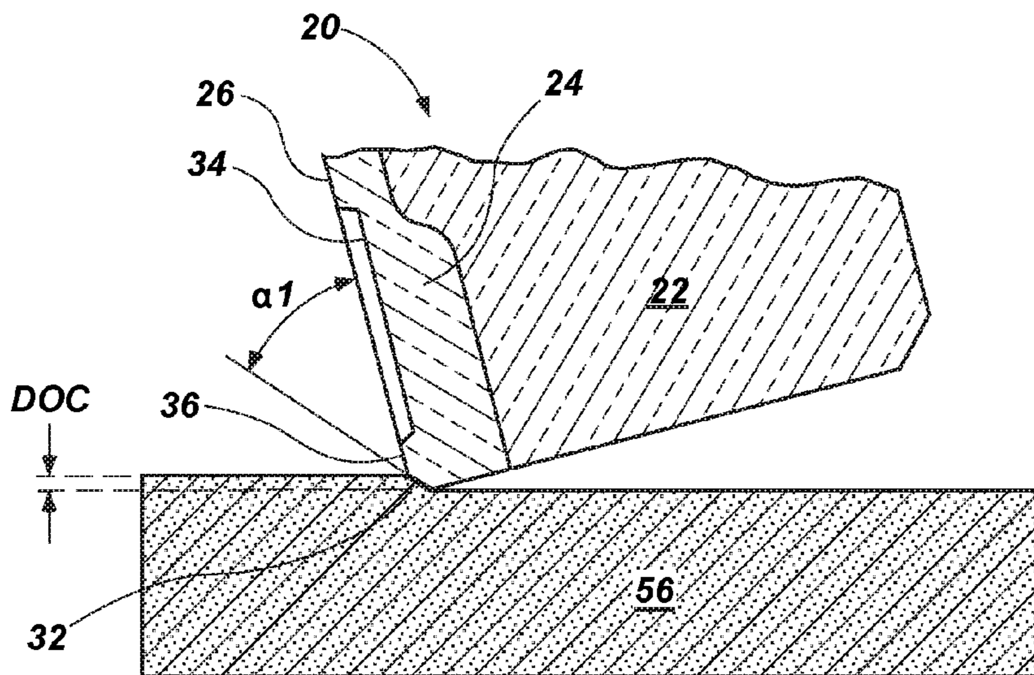
FIG. 27
