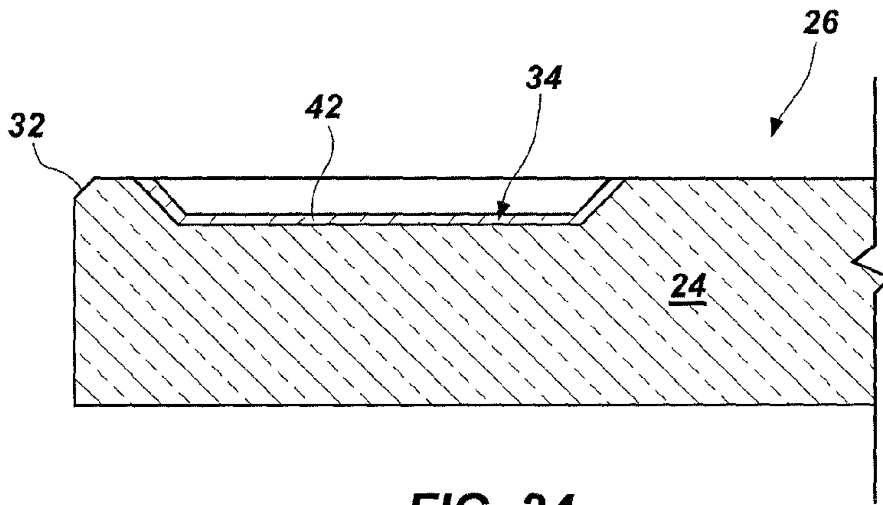
FIG. 24
