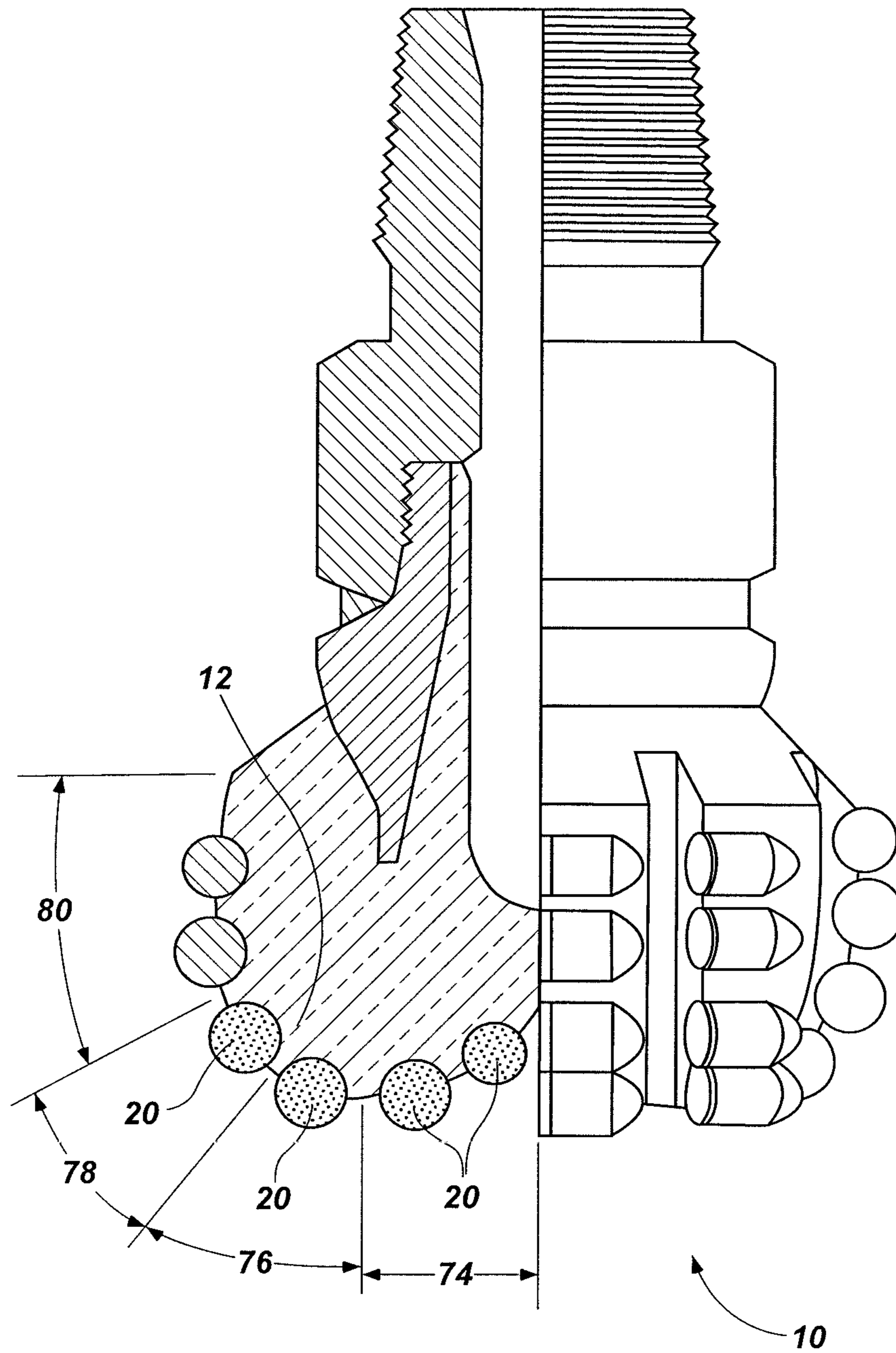
FIG. 31
