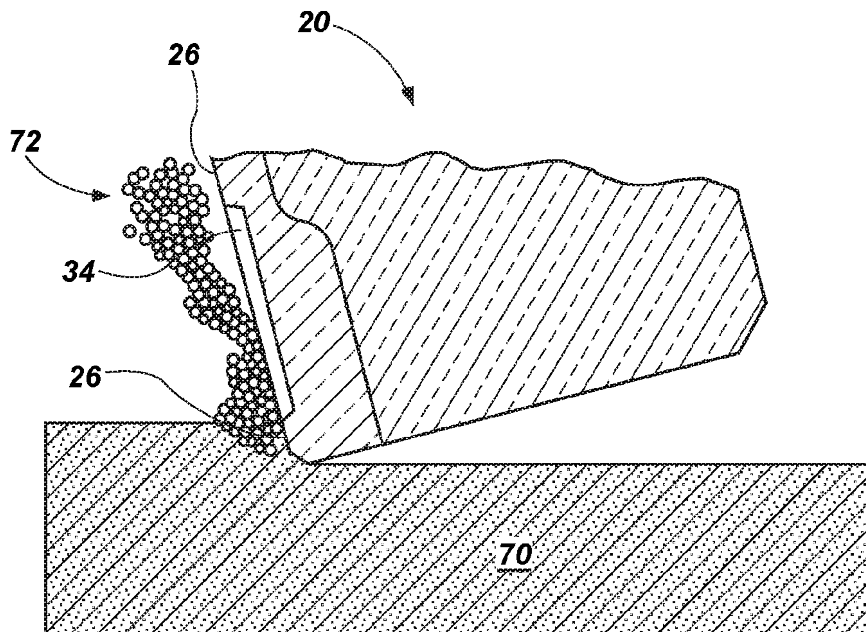
FIG. 30
