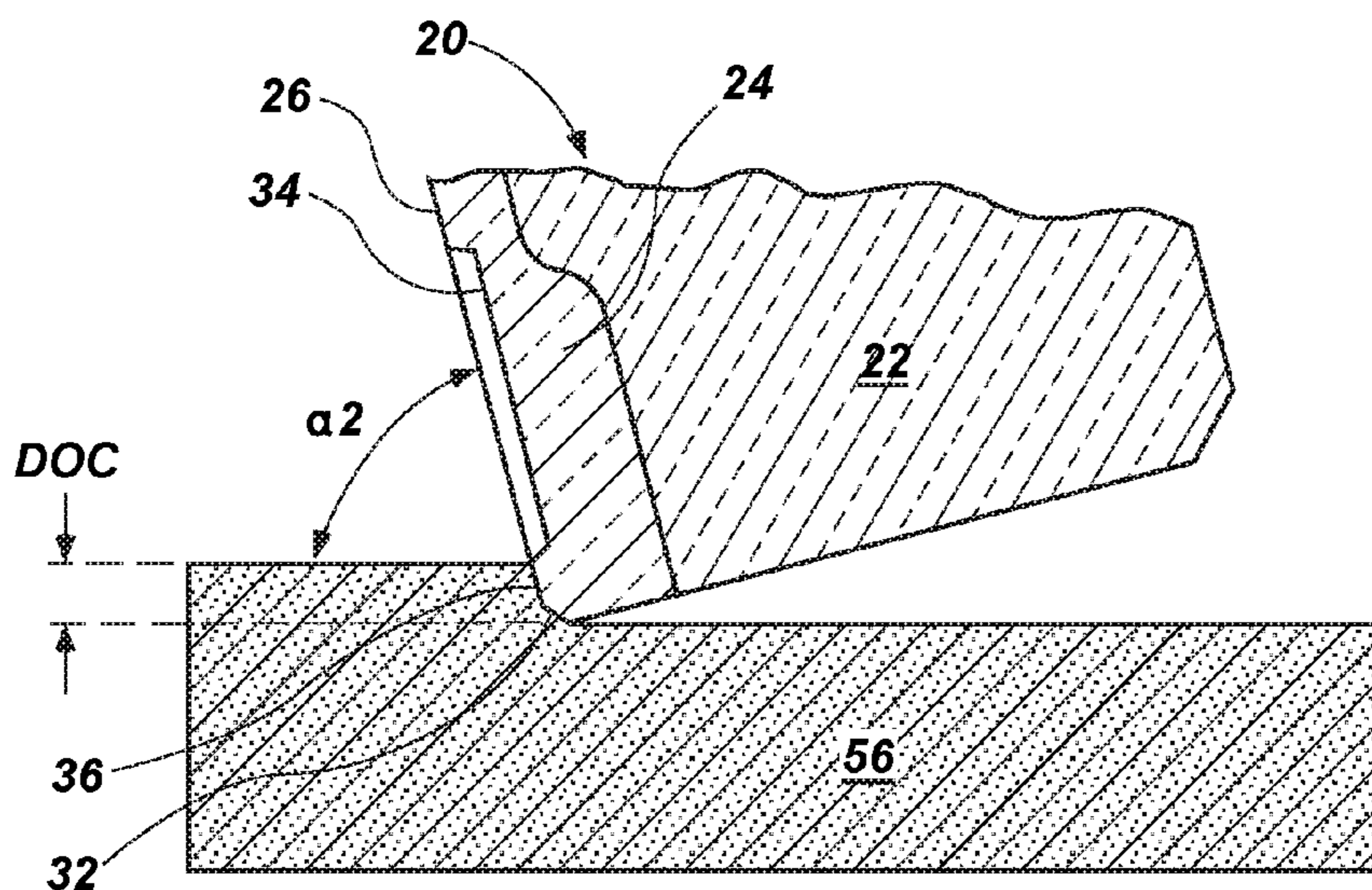
FIG. 28
