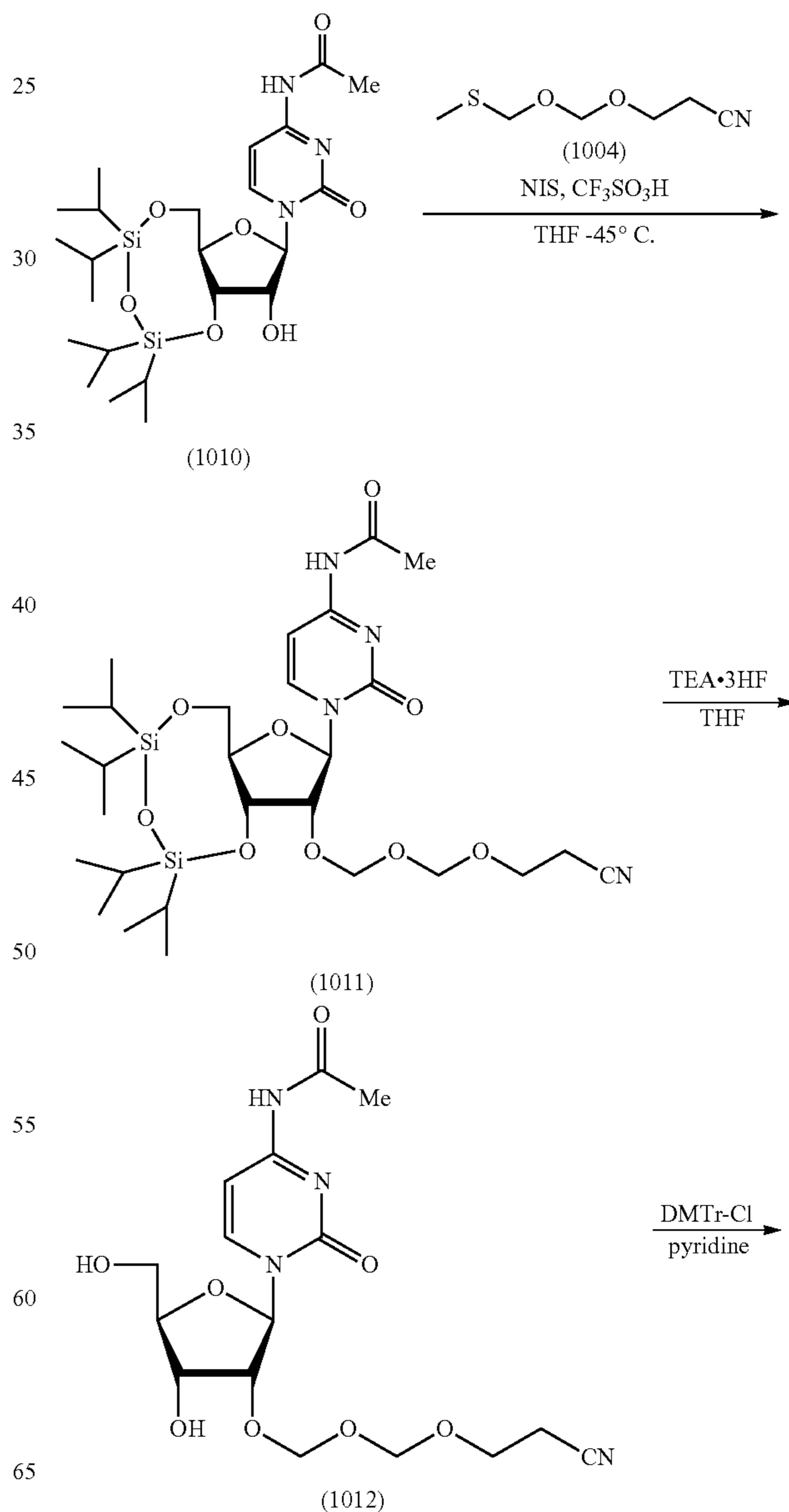
Scheme E3
