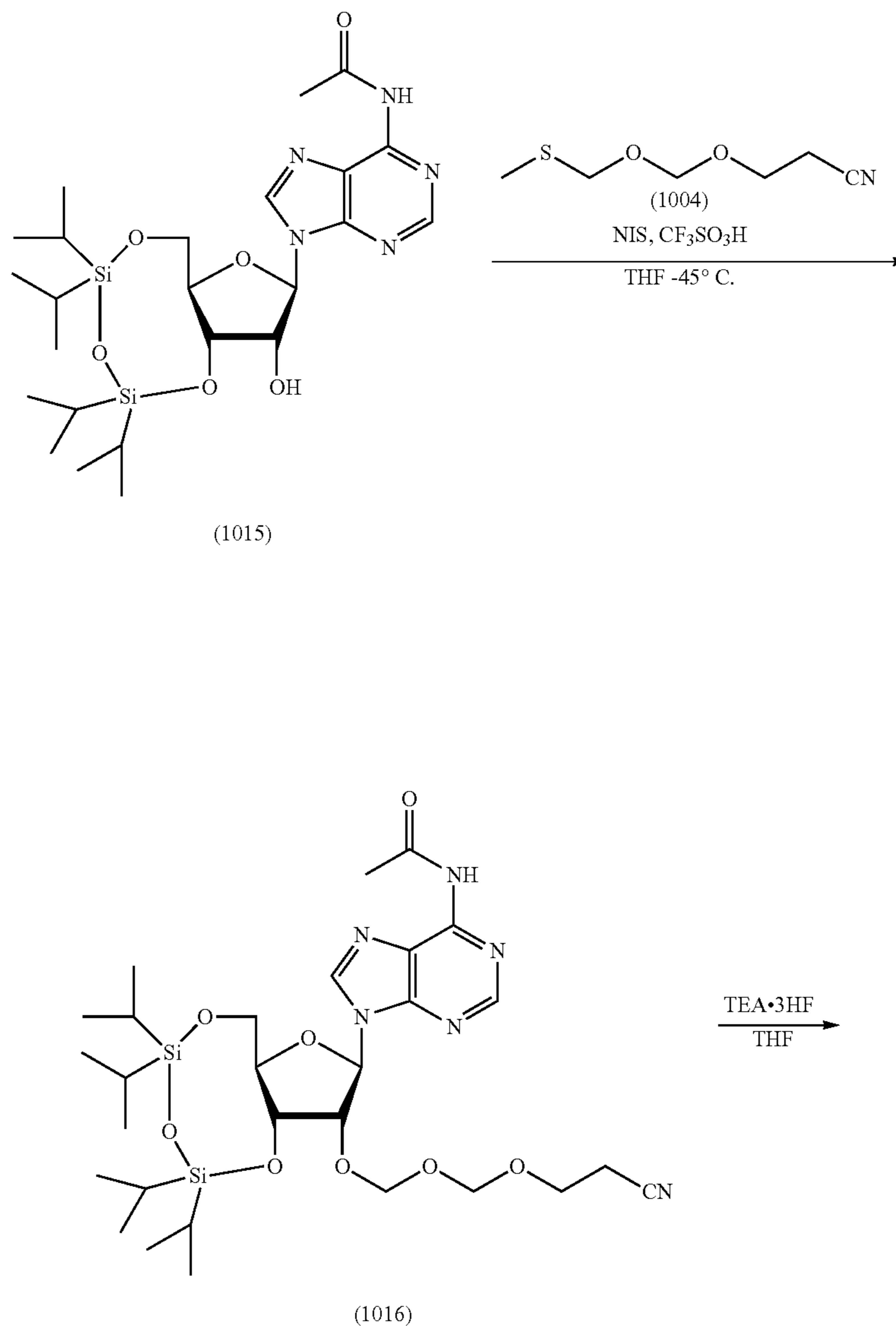
Scheme E4
