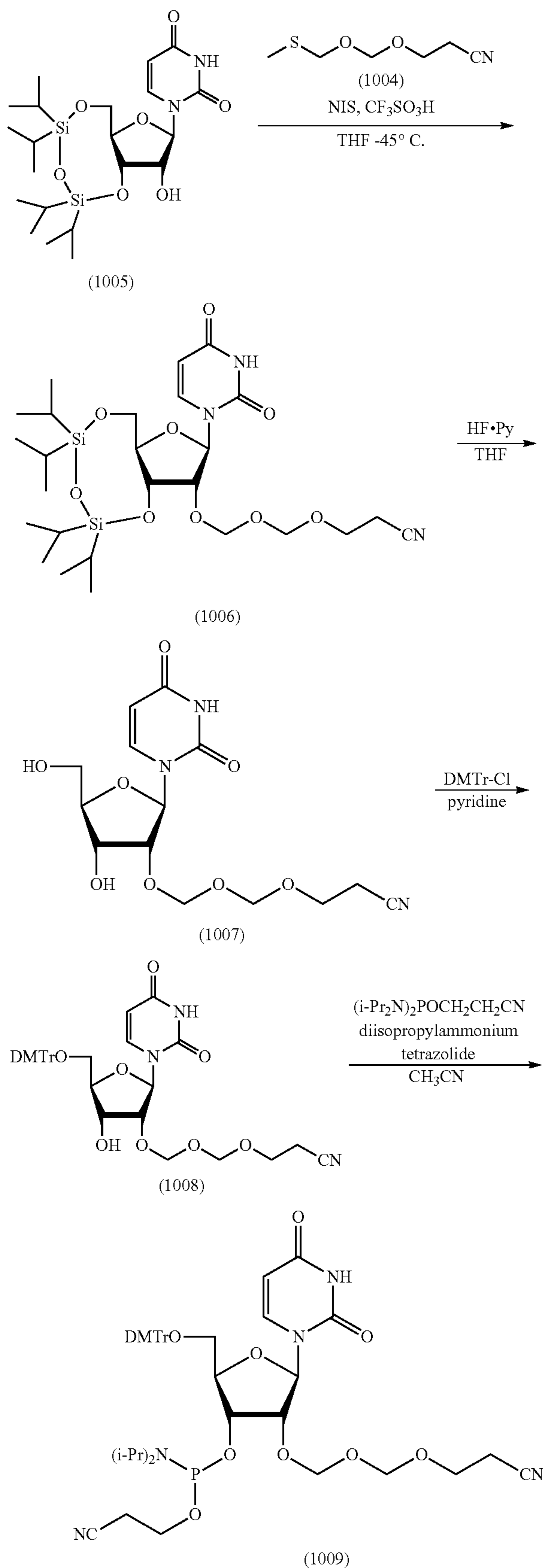
Scheme E2
