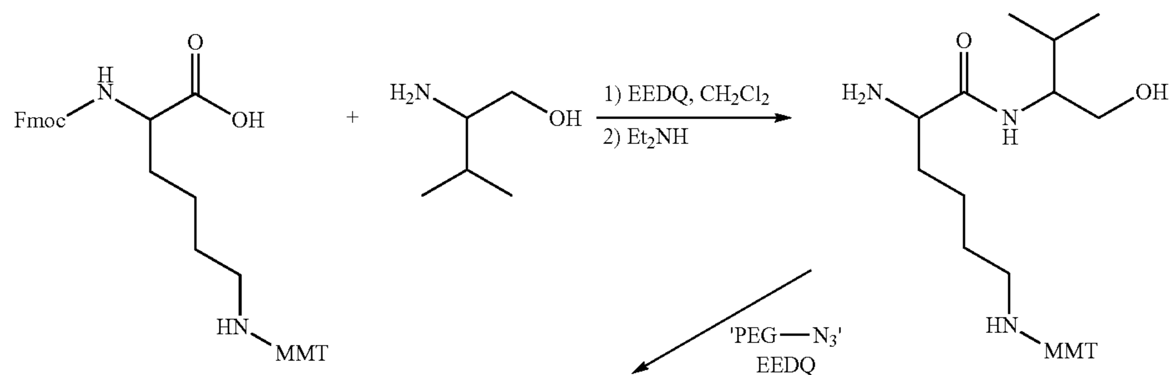
Scheme-2
