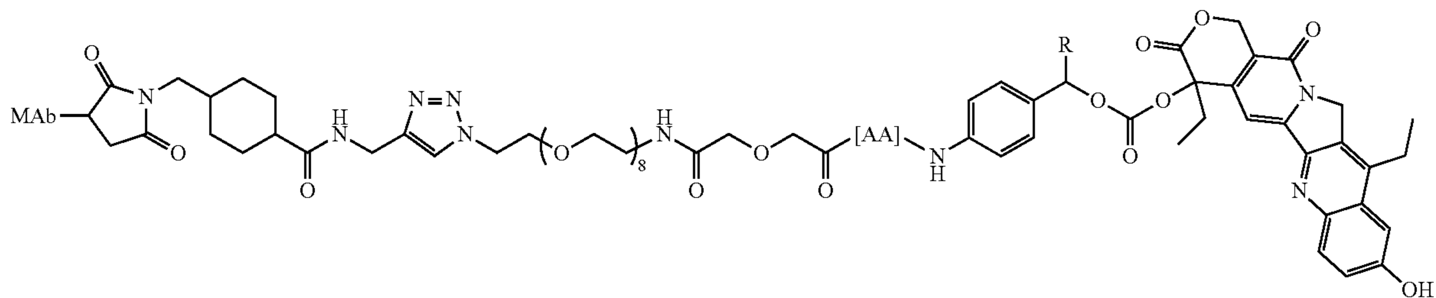
MAb-CLX-SN-38
