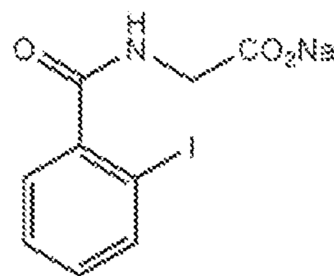
o-Iodohippurate (2) MW: 327
