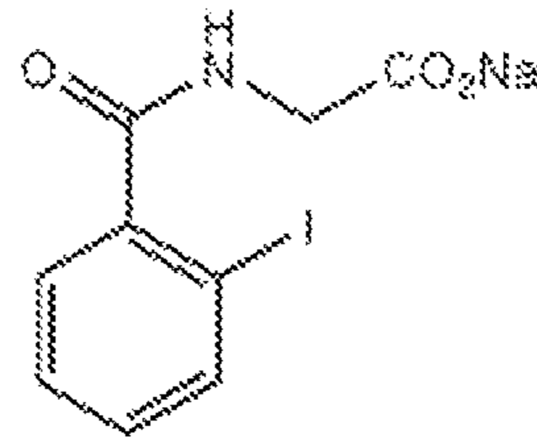
o-Iodohippurate (2) MW: 327
