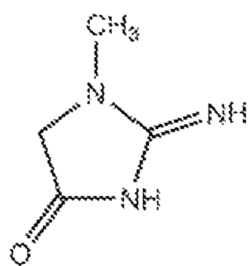
Creatinine (1) MW: 113
