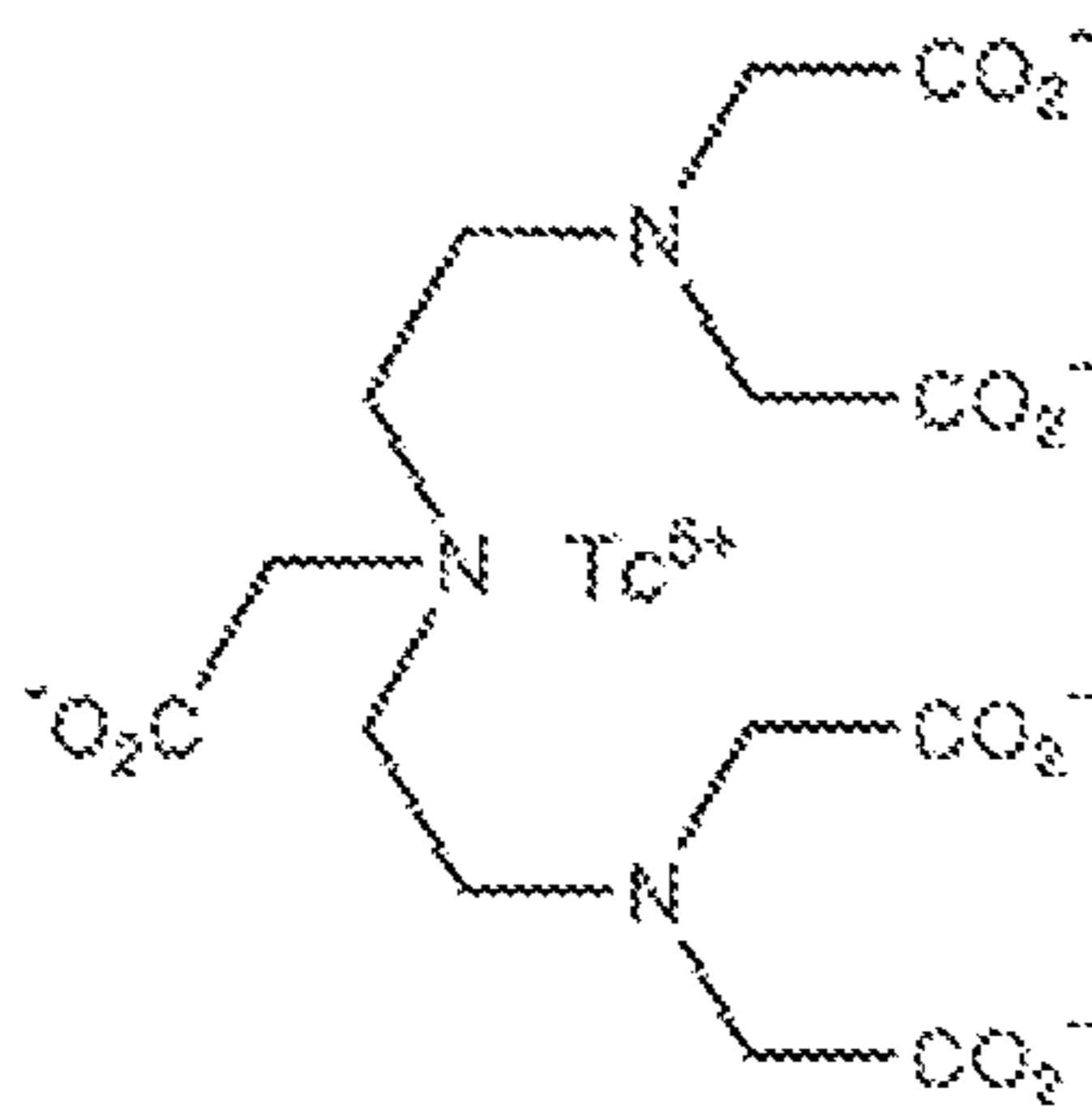
99m Tc-DTPA (3) MW: 487
