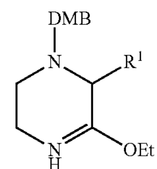
1 (DMB)
