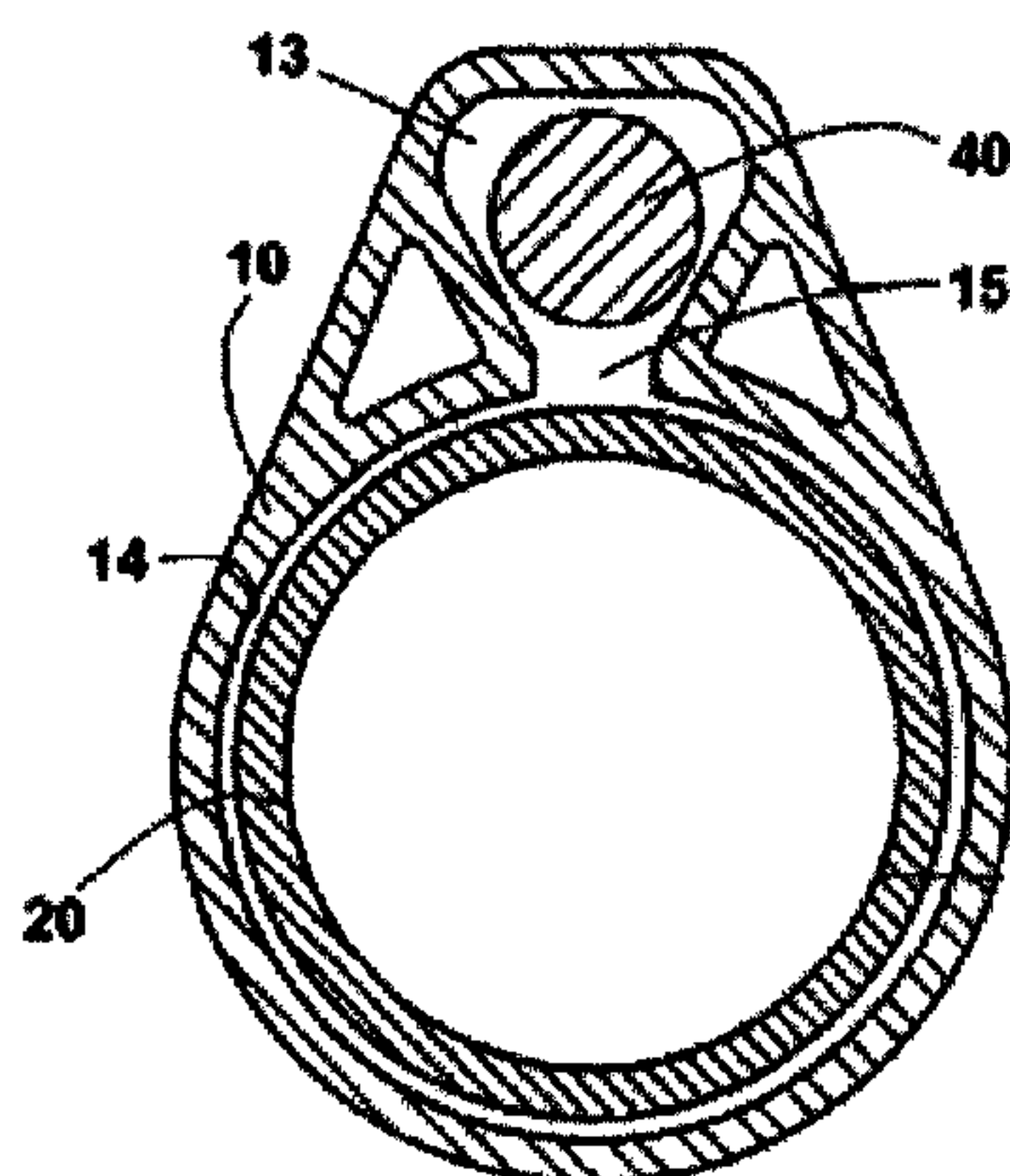
FIG.8 B-B
